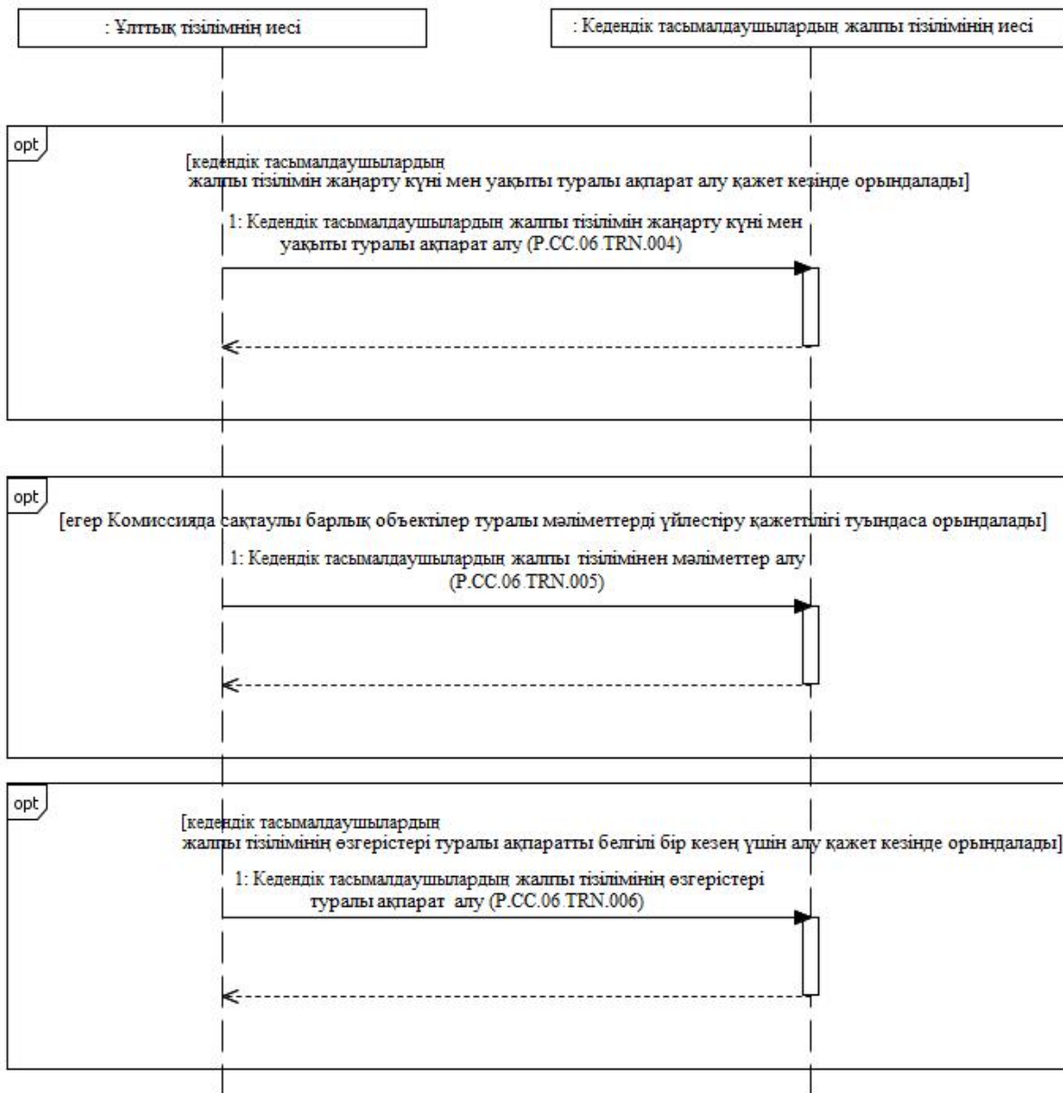
3-сурет. Кедендік тасымалдаушылардың жалпы тізіліміндегі мәліметтерді мүше мемлекеттердің уәкілетті органдарына ұсыну кезіндегі жалпы процесс транзакцияларының орындалу схемасы
