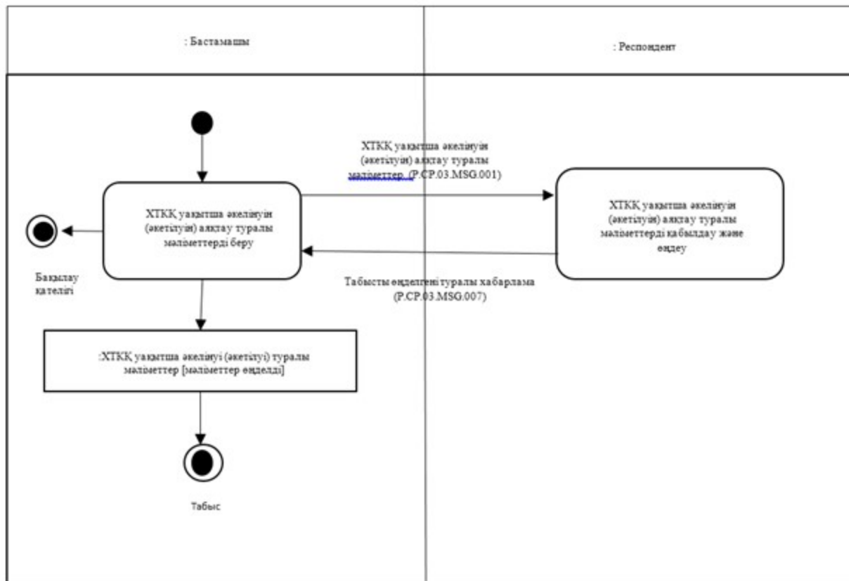
9-сурет. "ХТКҚ уақытша әкелінуін (әкетілуін) аяқтау туралы мәліметтерді беру" ( P.SP.03.TRN.003) жалпы процесінің транзакциясын орындау схемасы 10-кесте
