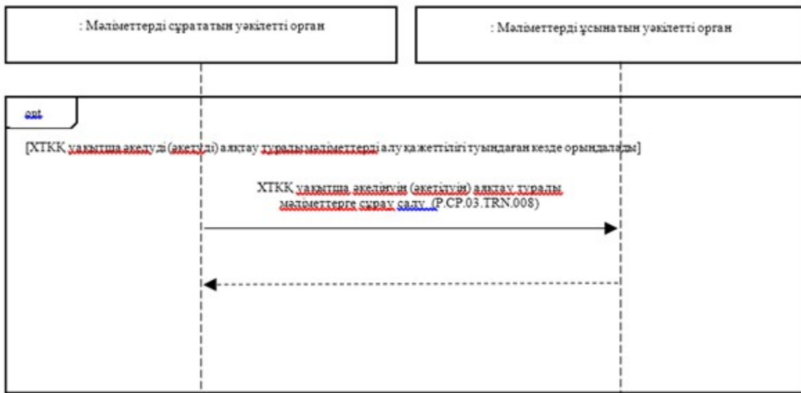
6-сурет. ХТКҚ уақытша әкелінуін (әкетілуін) аяқтау туралы мәліметтерге сұрау салу кезіндегі жалпы процесс транзакцияларын орындау схемасы 6-кесте
