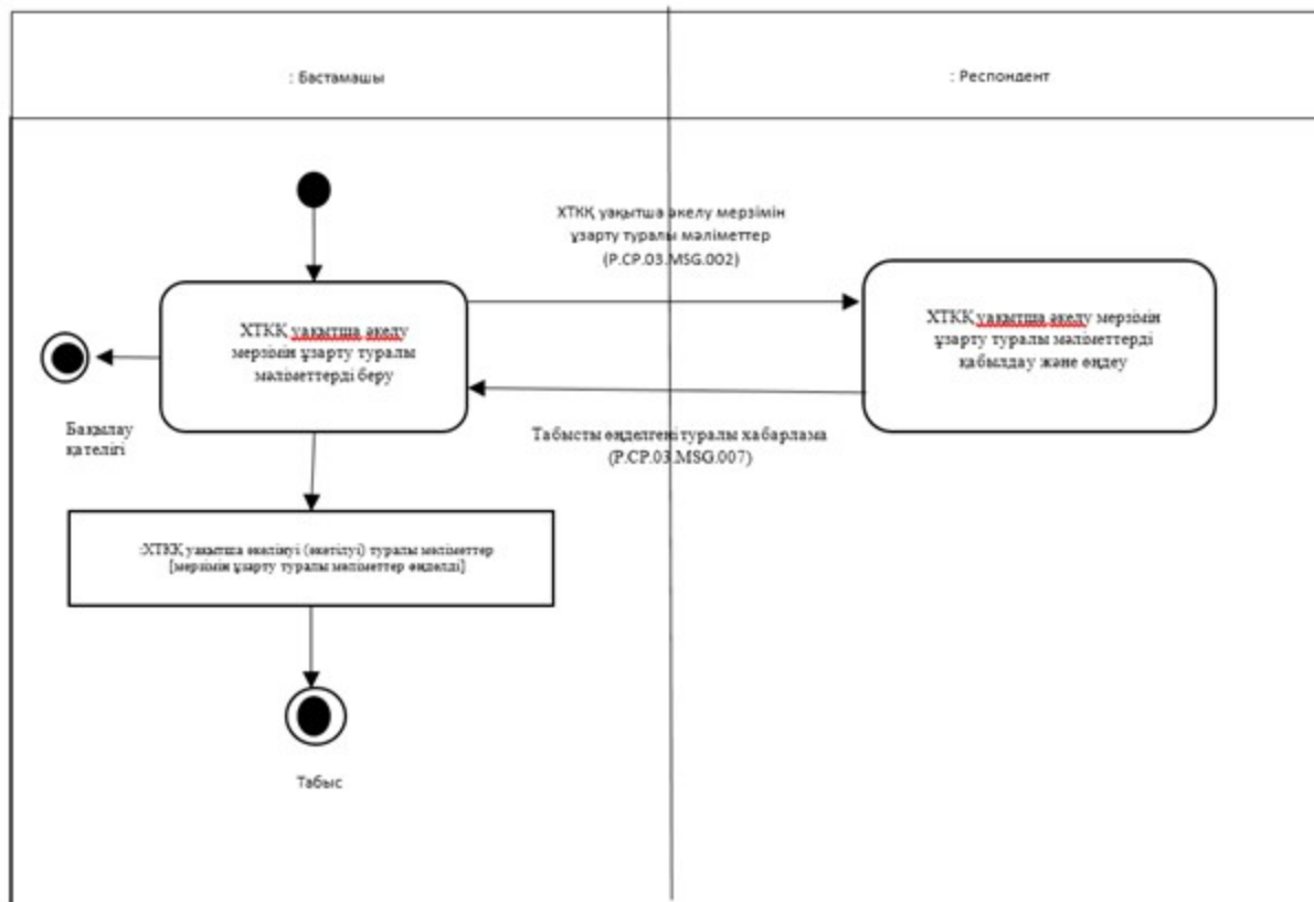
7-сурет. "ХТКҚ уақытша әкелу мерзімін ұзарту туралы мәліметтерді беру" (P.CP.03. TRN.001) жалпы процесінің транзакцияларын орындау схемасы 8-кесте
