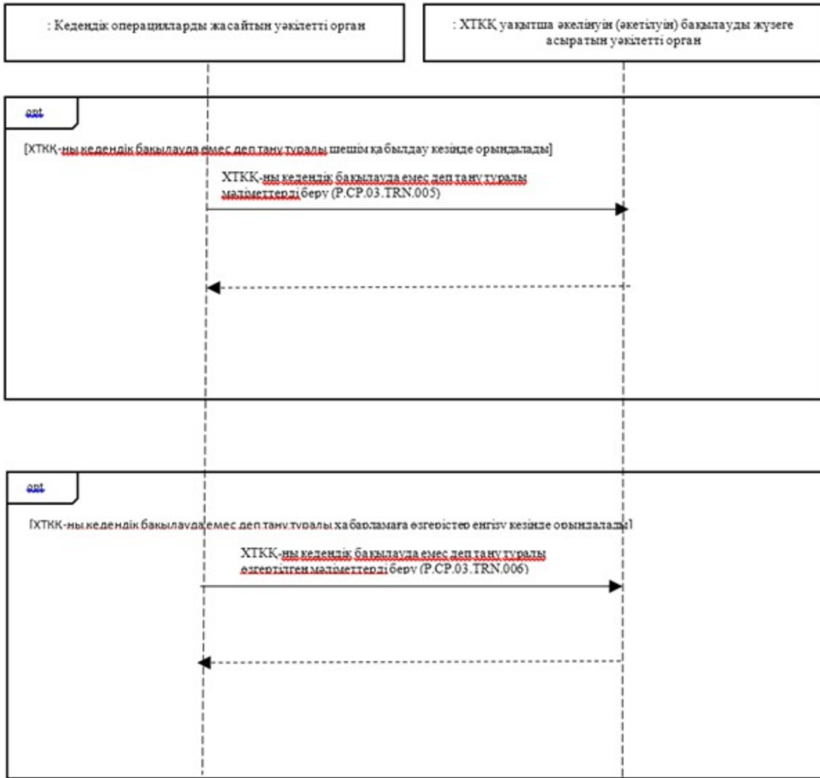
4-сурет. ХТКҚ-ны кедендік бақылауда емес деп тану кезіндегі жалпы процесс транзакцияларын орындау схемасы
