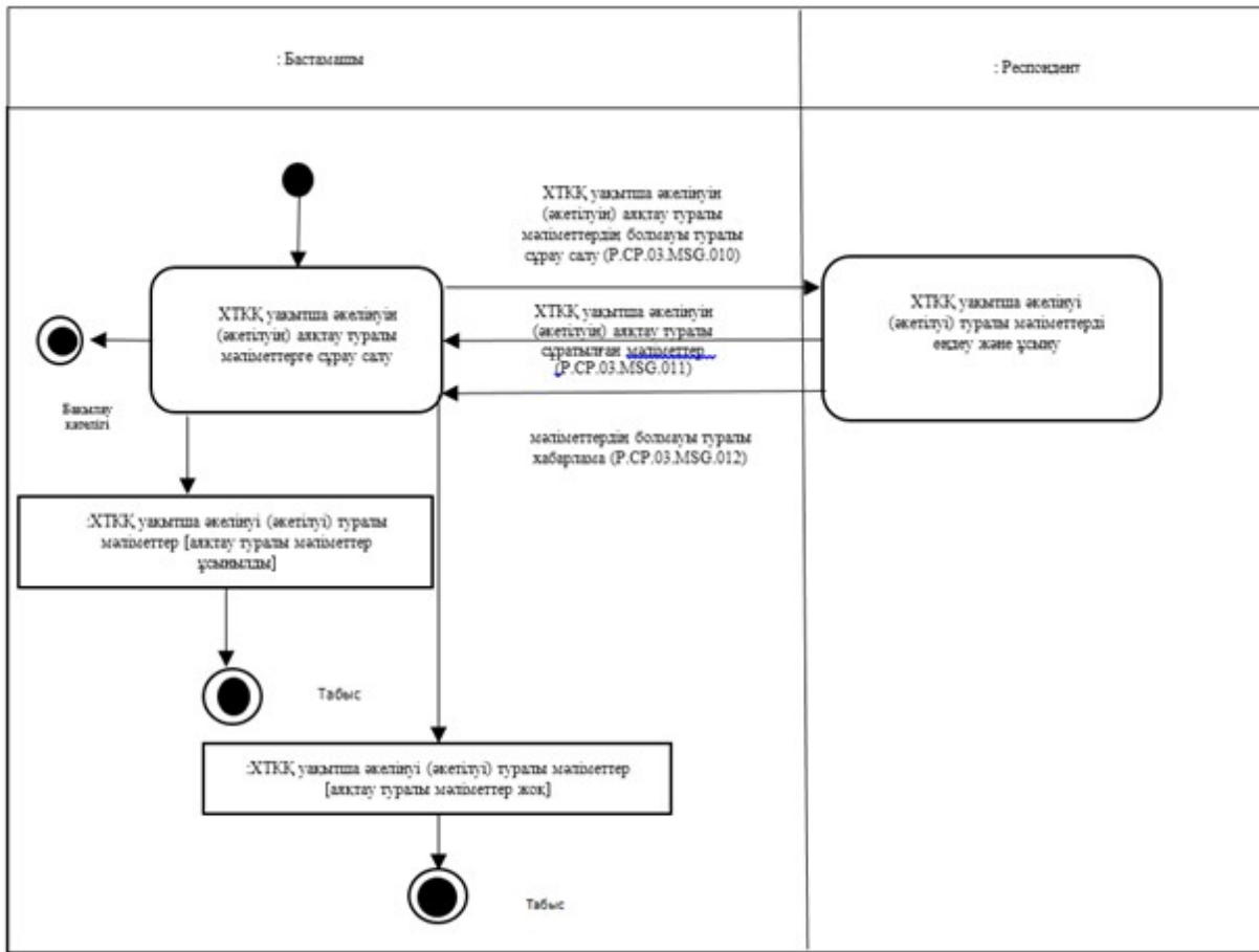
14-сурет. "ХТКҚ уақытша әкелінуін (әкетілуін) аяқтау туралы мәліметтерге сұрау салу" (P.SP.03.TRN.008) жалпы процесінің транзакциясын орындау схемасы 15-кесте
