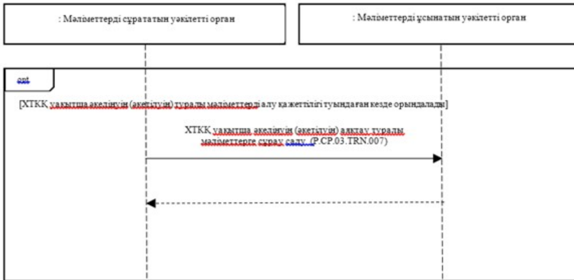
5-сурет. ХТКҚ уақытша әкелінуі (әкетілуі) туралы мәліметтерге сұрау салу кезіндегі жалпы процесс транзакцияларын орындау схемасы
