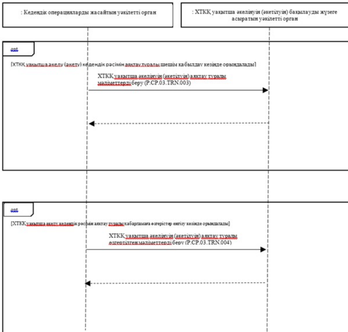
3-сурет. ХТКК уақытша әкелінуін (әкетілуін) аяқтау кезіндегі жалпы процесс транзакцияларын орындау схемасы
