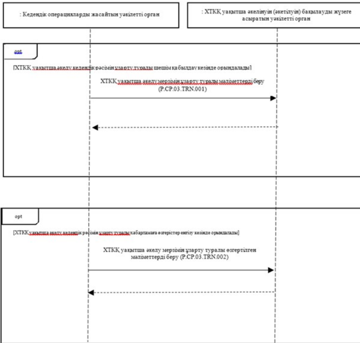
2-сурет. ХТКҚ уақытша әкелу мерзімін ұзарту кезіндегі жалпы процесс транзакциясын орындау схемасы
