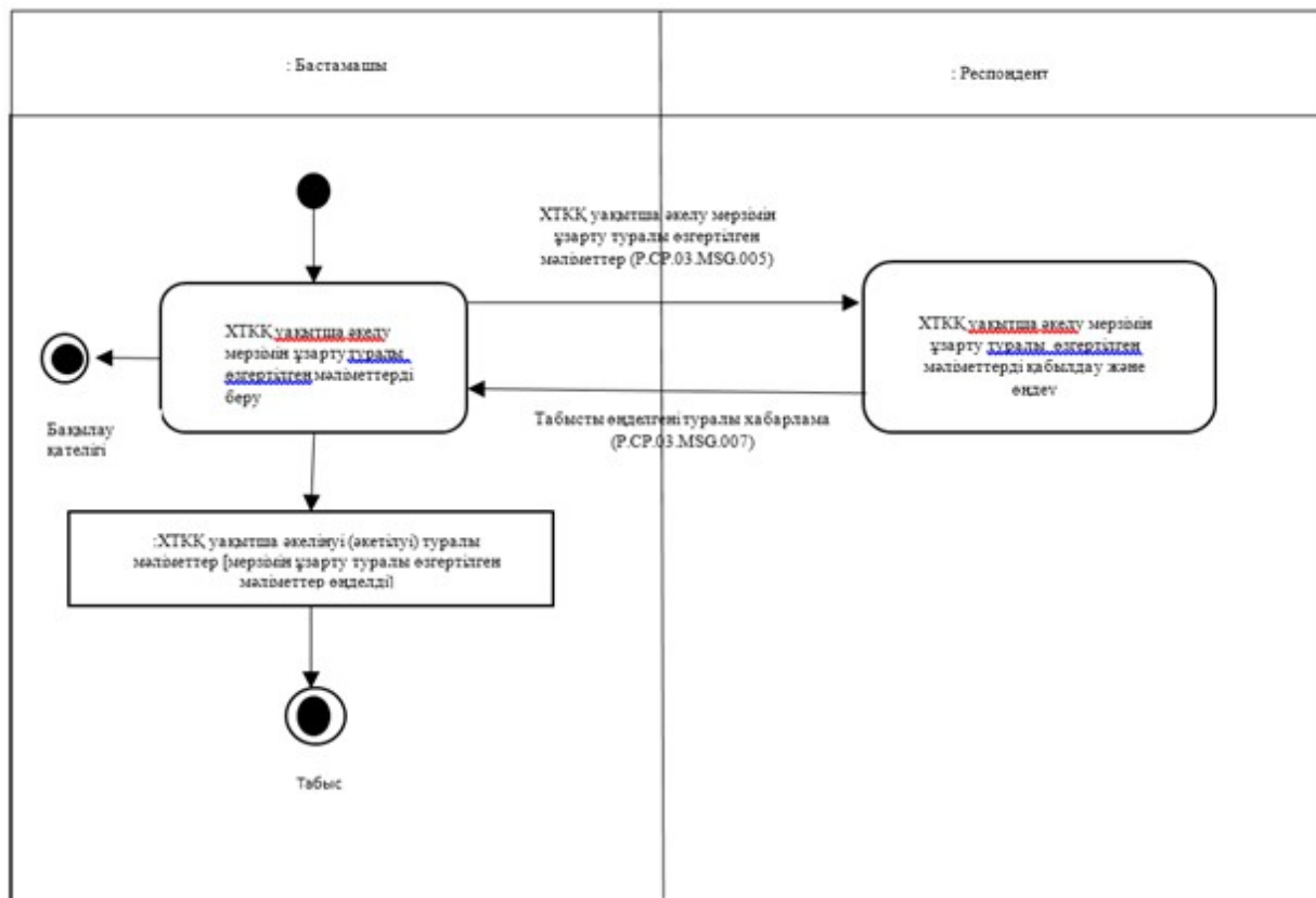
8-сурет. "ХТКҚ уақытша әкелу мерзімін ұзарту туралы өзгертілген мәліметтерді беру" (P.CP.03.TRN.002) жалпы процесінің транзакцияларын орындау схемасы 9-кесте
