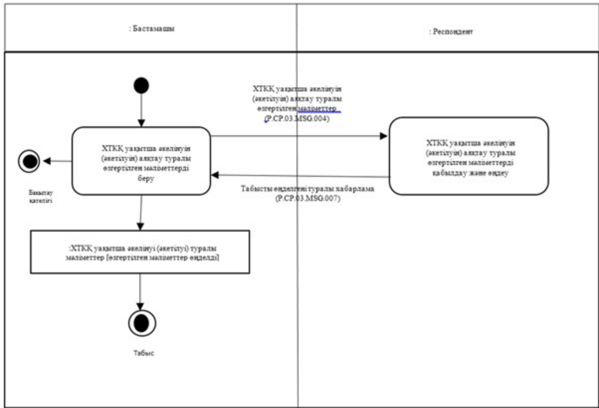
10-сурет. "ХТКҚ уақытша әкелінуін (әкетілуін) аяқтау туралы өзгертілген мәліметтерді беру" (P.SP.03.TRN.004) жалпы процесінің транзакциясын орындау схемасы
