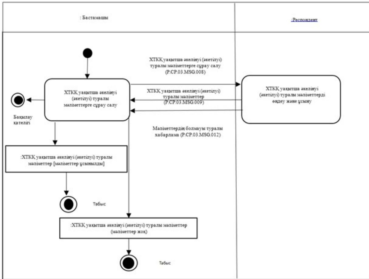
13-сурет. "ХТКҚ уақытша әкелінуі (әкетілуі) туралы мәліметтерге сұрау салу" (P.SP.03.TRN.007) жалпы процесінің транзакцияларын орындау схемасы 14-кесте
