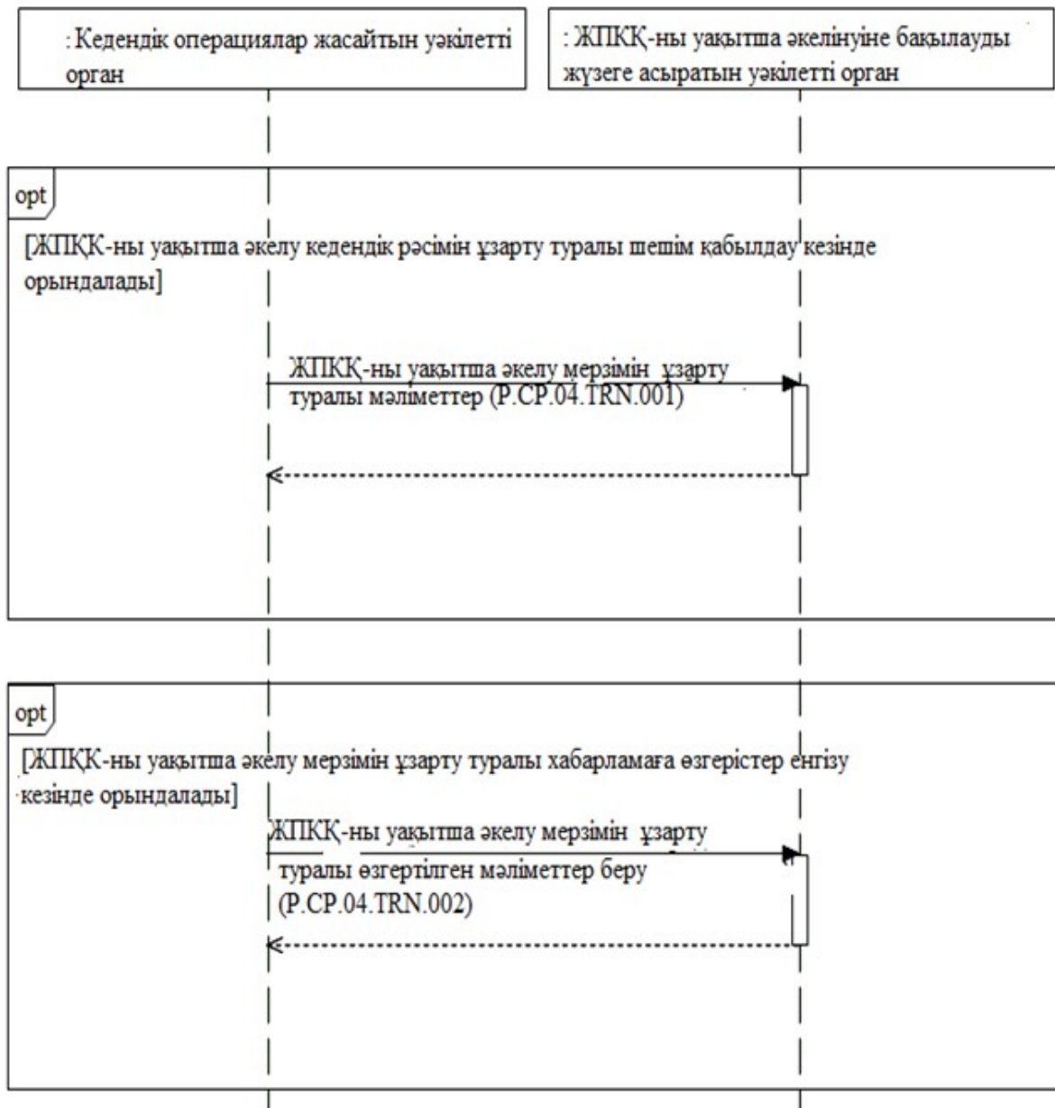
2-сурет. ЖПКҚ уақытша әкелу мерзімін ұзарту кезіндегі жалпы процестің транзакцияларын орындау схемасы
