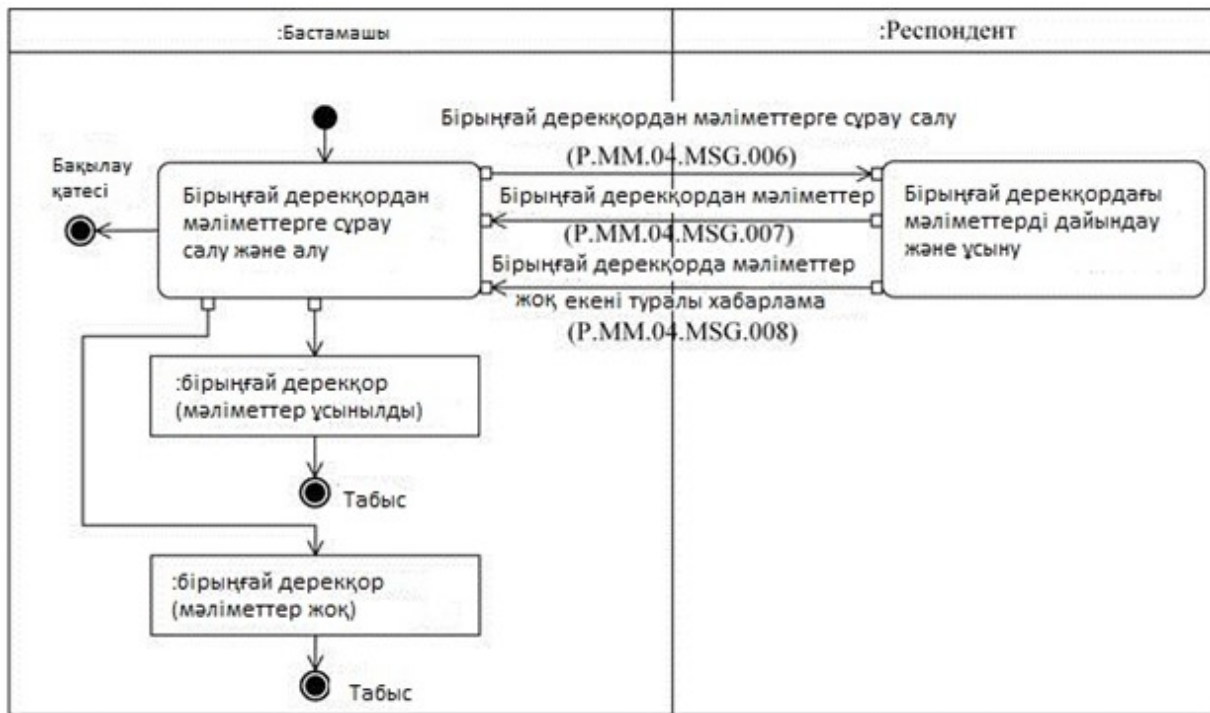
7-сурет. "Бірыңғай дерекқордан мәліметтерді алу" (P.MM.04.TRN.004) жалпы процесс транзакциясын орындау схемасы 8-кесте
