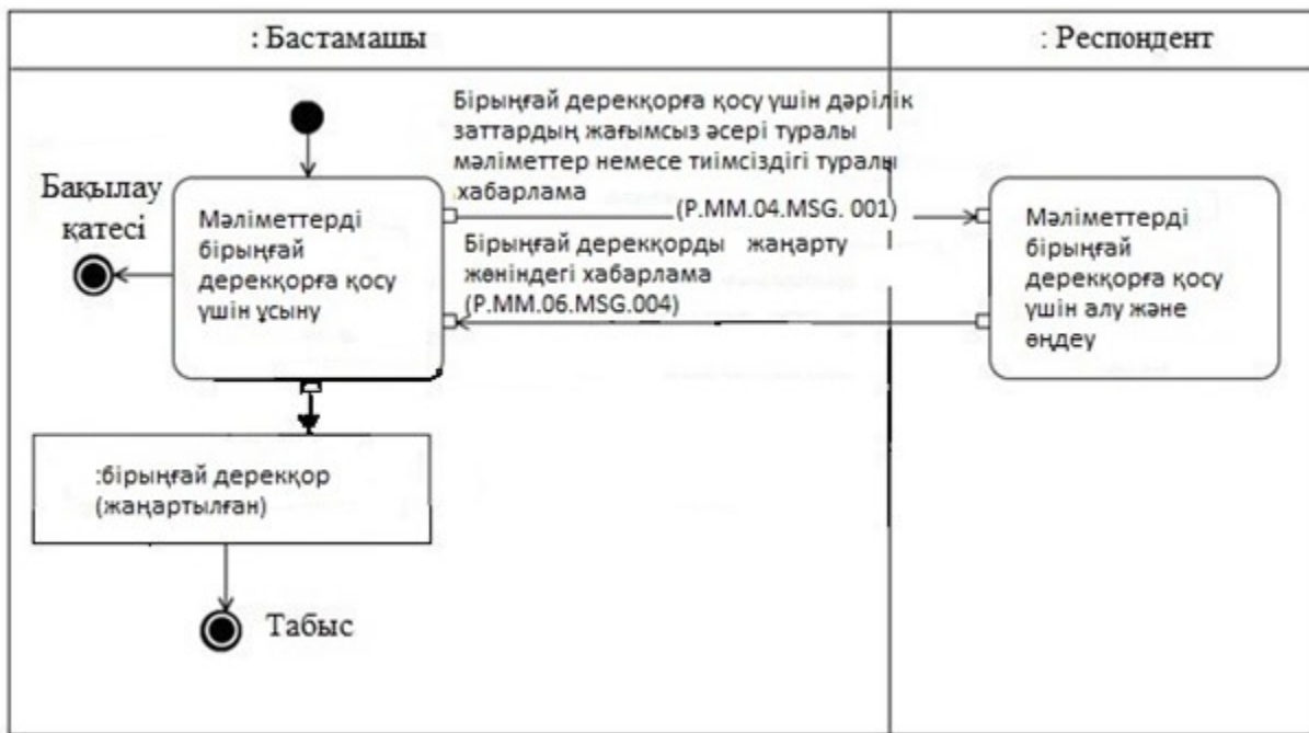
4-сурет. "Мәліметтерді бірыңғай дерекқорға қосу үшін беру" (P.MM.04.TRN.001) жалпы процесс транзакциясын орындау схемасы 5-кесте
