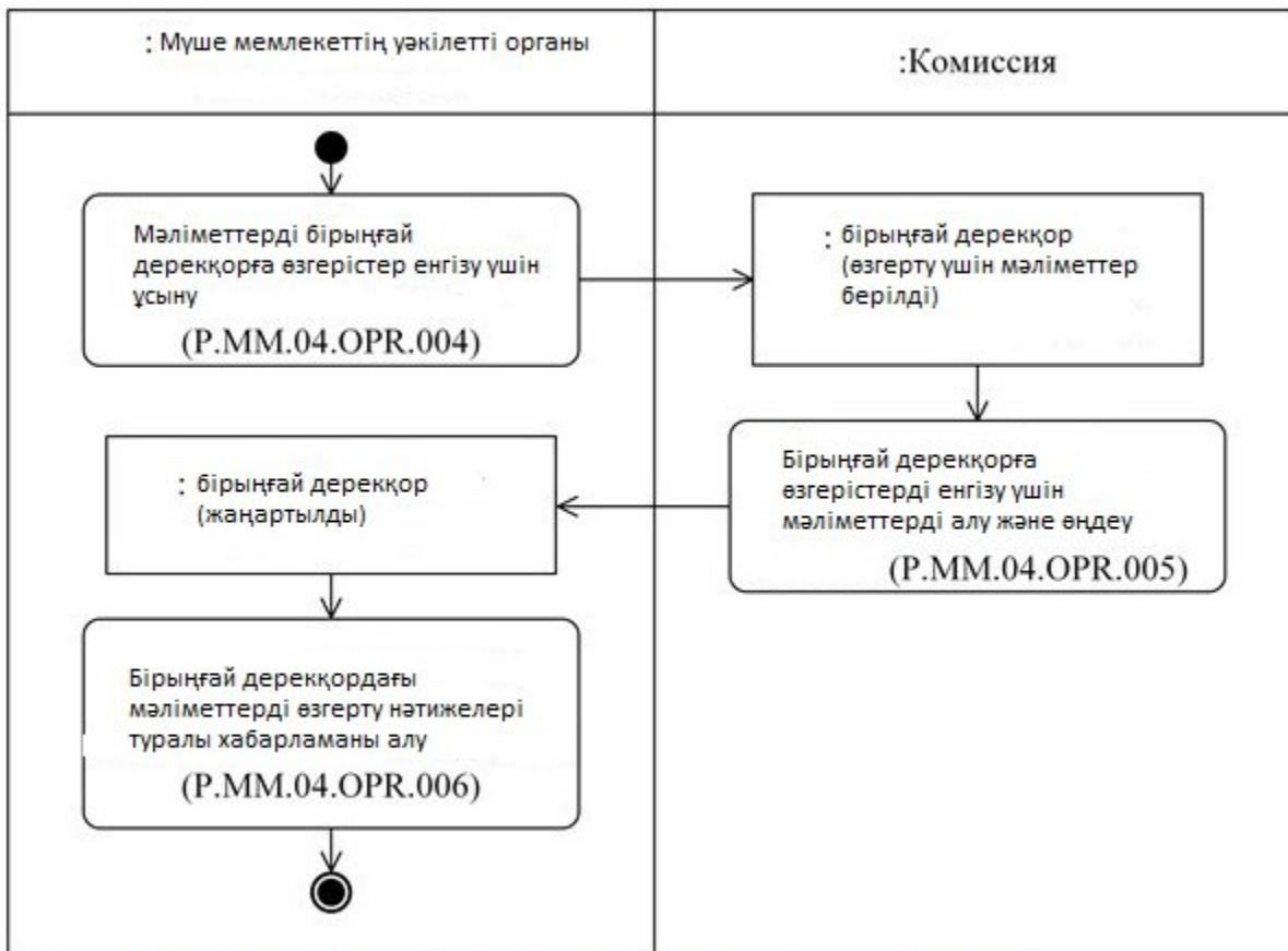
5 сурет. «Бірыңғай дерекқордағы мәліметтерді өзгерту» рәсімін орындау сұлбасы (P.MM.04.PRC.002)
