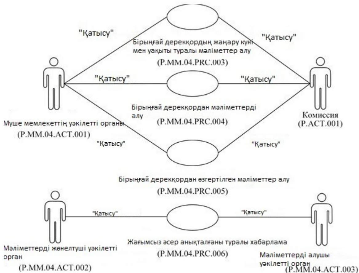
3-сурет. Бірыңғай дерекқордан мәліметтерді алу рәсімдері тобының жалпы кестесі
