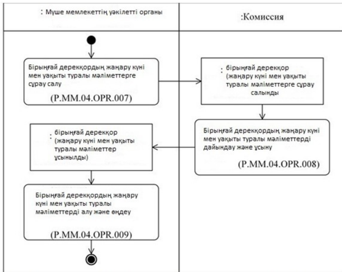
6-сурет. «Бірыңғай дерекқордың жаңару күні мен уақыты туралы мәліметтер алу» рәсімін орындау сұлбасы (P.MM.04.PRC.003)
