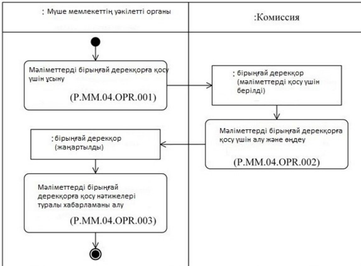
4-сурет. «Мәліметтерді бірыңғай дерекқорға енгізу» рәсімін орындау сұлбасы (P.MM.04.PRC.001)
