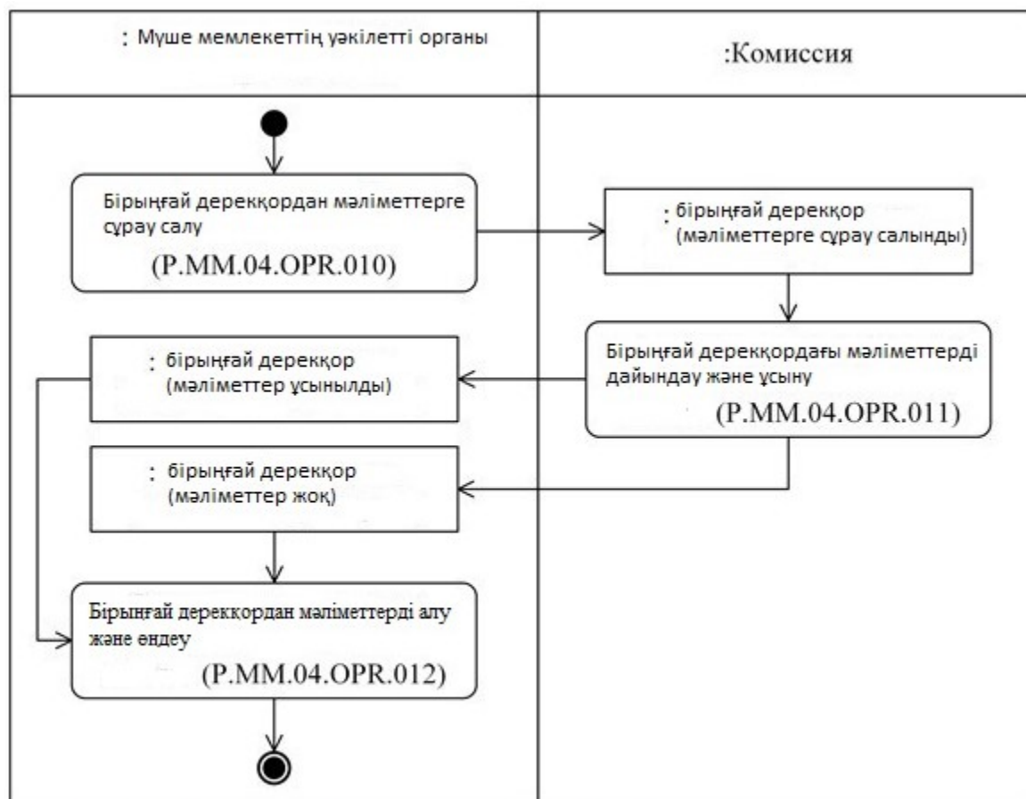
7-сурет. «Бірыңғай дерекқордан мәліметтер алу» рәсімін орындау сұлбасы (P.MM.04.PRC.004)
