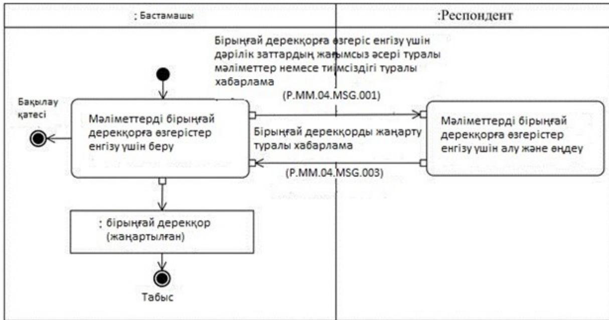
5-сурет. "Мәліметтерді бірыңғай дерекқорға өзгерістер енгізу үшін беру" (P.MM.04. TRN.002) жалпы процесс транзакциясын орындау схемасы 6-кесте
