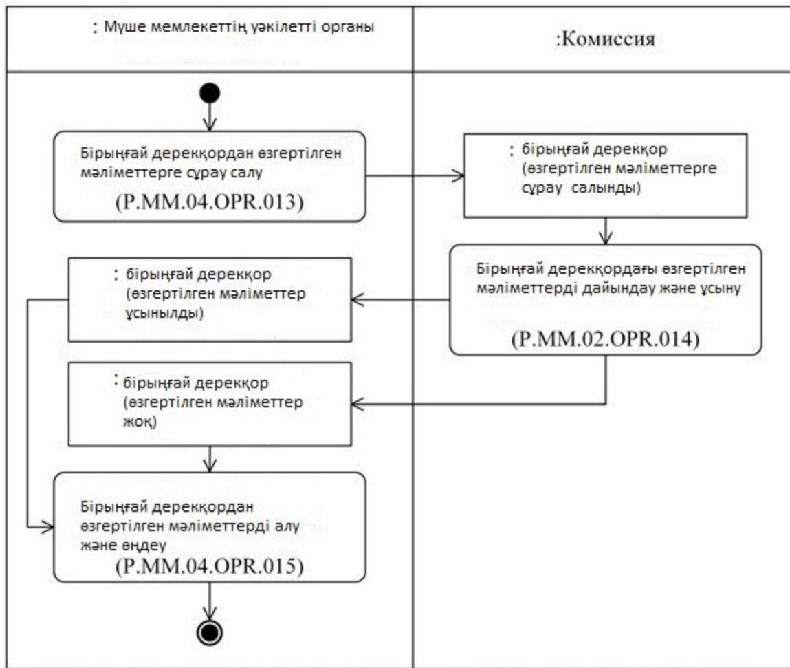
8-сүрет. «Бірыңғай дерекқордан өзгертілген мәліметтер алу» рәсімін орындау сұлбасы (P.MM.04.PRC.005)
