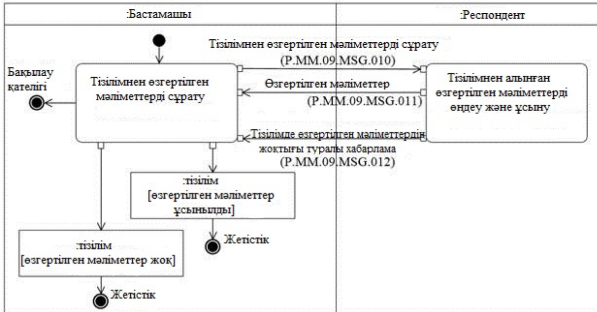
9-сурет. "Тізілімнен өзгертілген мәліметтерді алу" (P.MM.09.PRC.006) жалпы процесс транзакциясын орындау схемасы 10-кесте
