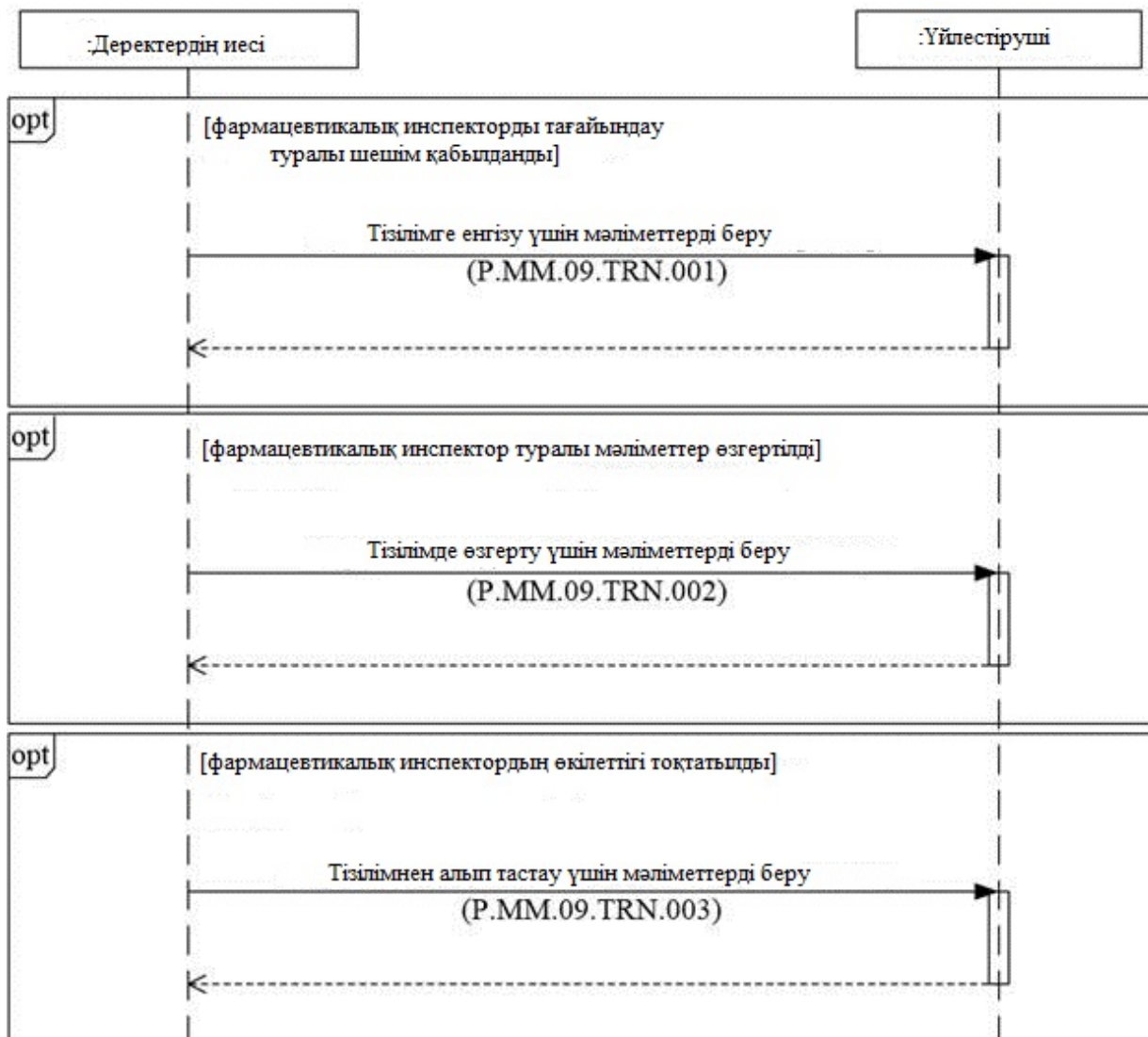
2-сурет. Тізбені қалыптастырған және жүргізген кездегі жалпы процесс транзакциясын орындау схемасы
