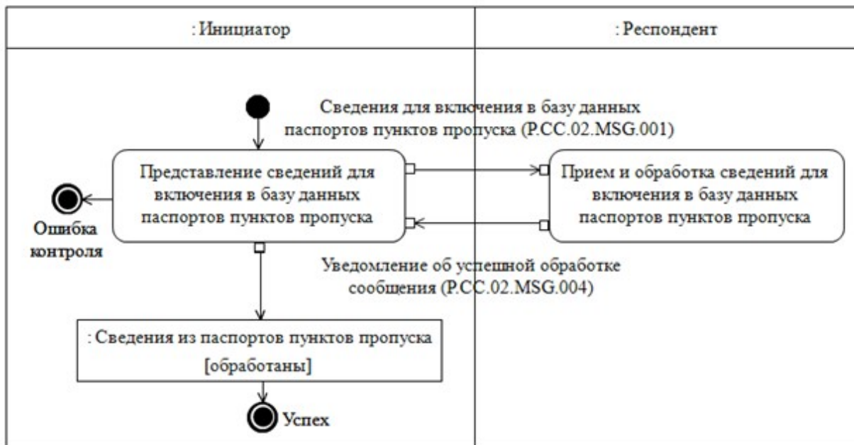
4-сурет. Жалпы процестің "Өткізу пункттері паспорттарының дерекқорына мәліметтер қосу" (P.CC.02.TRN.001) транзакциясының орындалу схемасы 5-кесте
