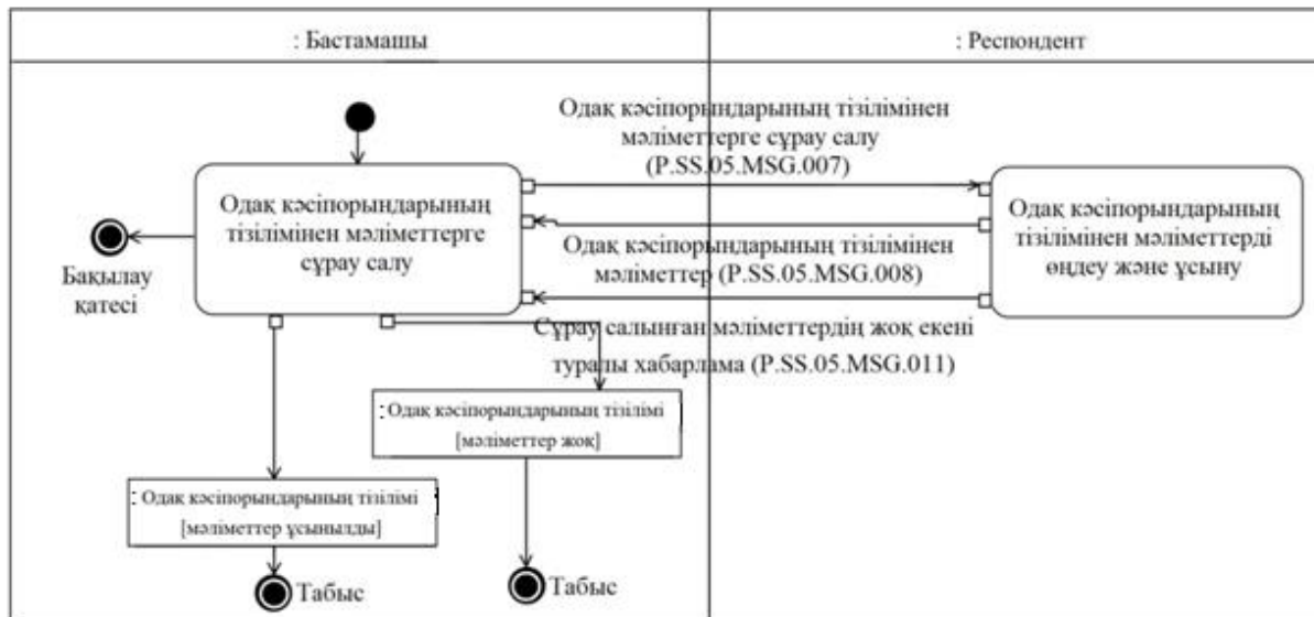
8-сурет. "Одақ кәсіпорындарының тізілімінен мәліметтер алу" (P.SS.05.TRN.005) жалпы процесс транзакциясын орындау схемасы 9-кесте
