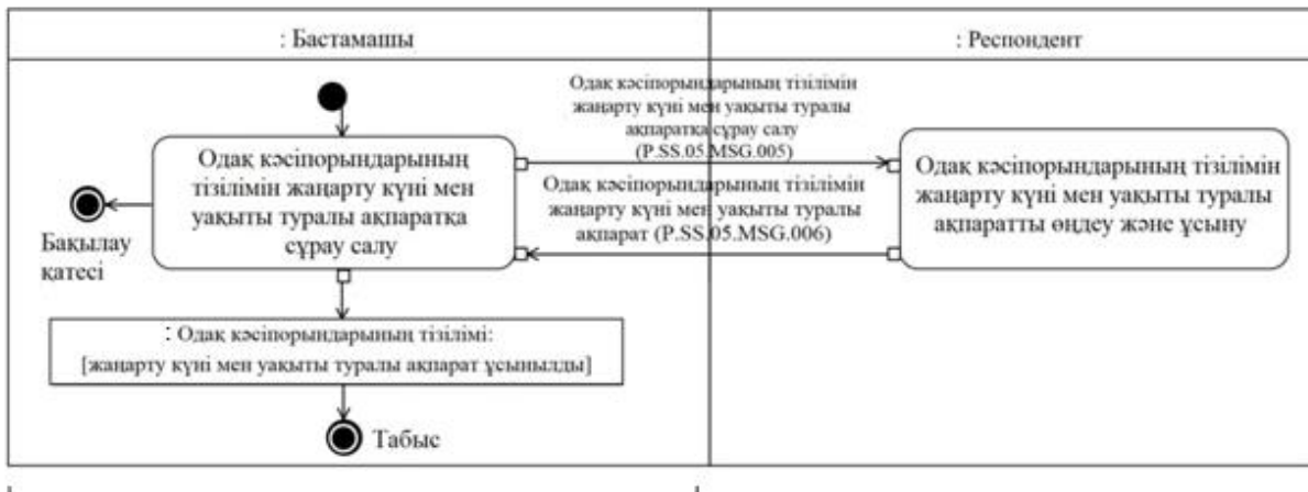
7-сурет. "Одақ кәсіпорындарының тізілімін жаңарту күні мен уақыты туралы ақпарат алу" (P.SS.05.TRN.004) жалпы процесс транзакциясын орындау схемасы 8-кесте
