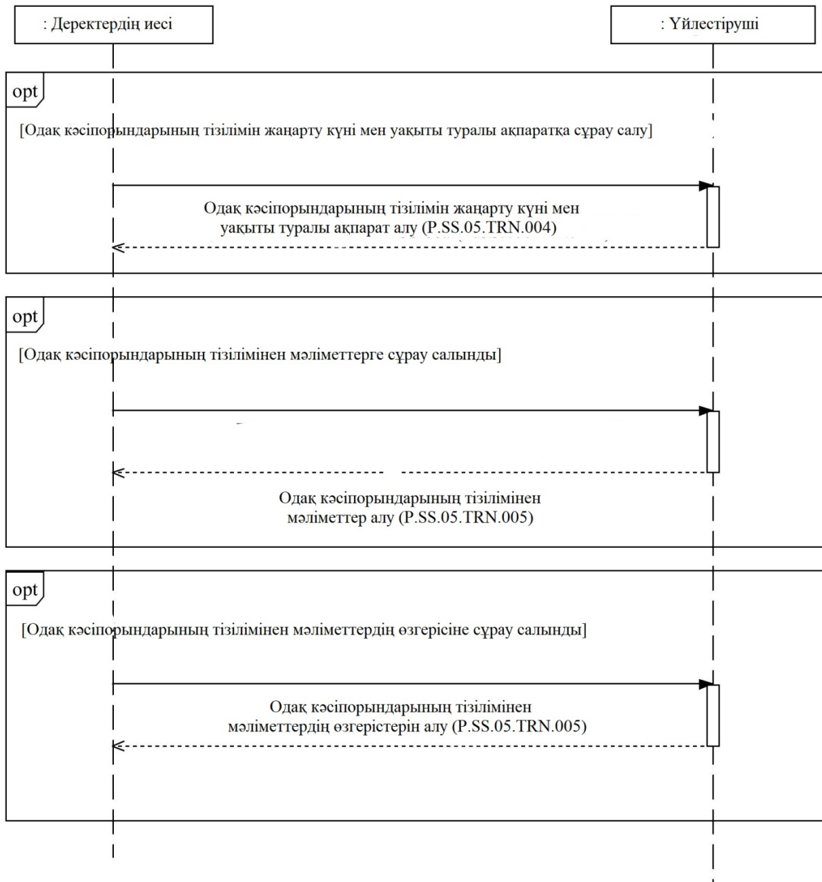
3-сурет. Одақ кәсіпорындарының тізілімінен мәліметтер алу кезінде жалпы процесс транзакцияларын орындау схемасы 3-кесте
