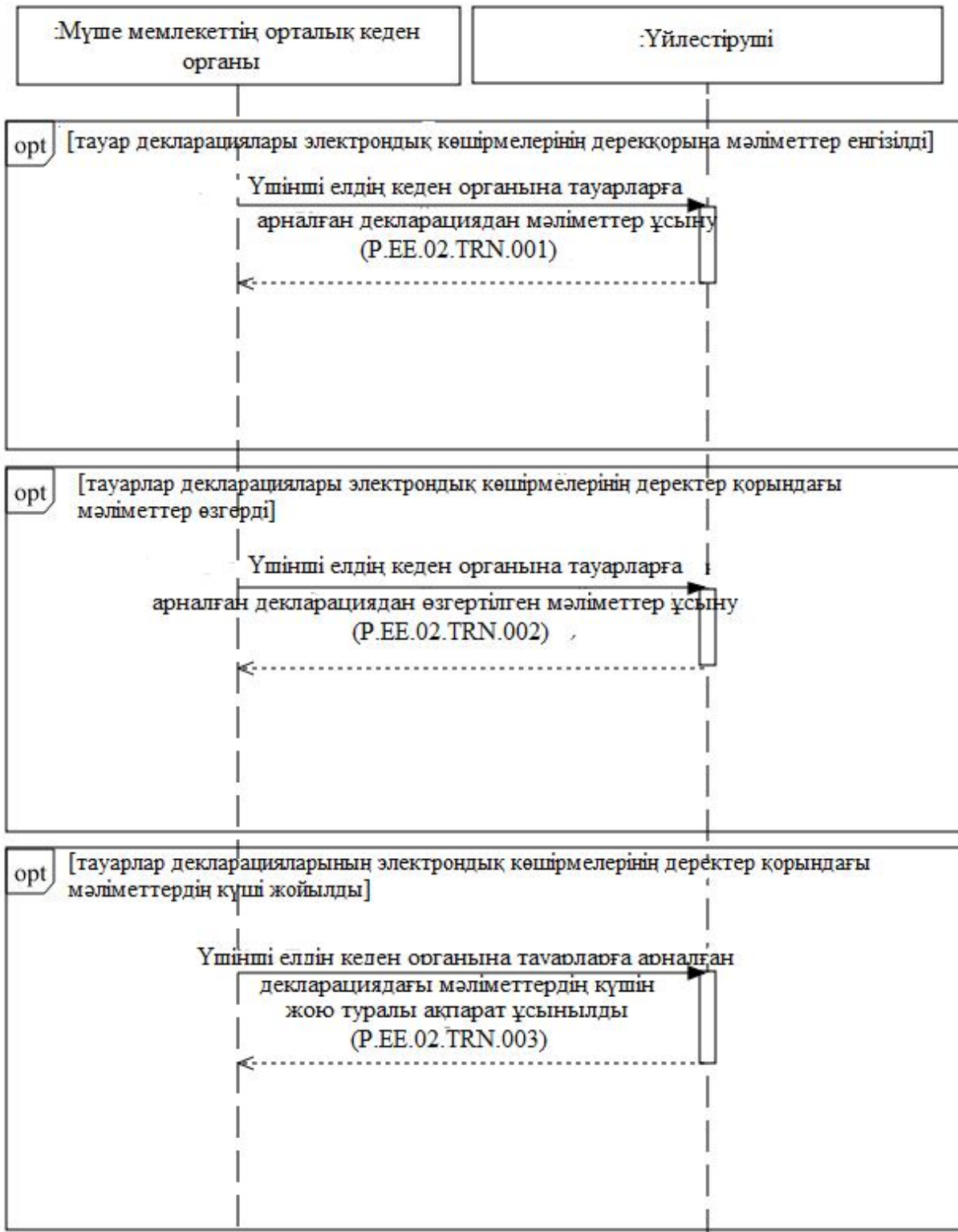
2-сурет. Тауарларға арналған декларациялардан мәліметтер ұсыну кезінде жалпы процестің транзакцияларын орындау схемасы
