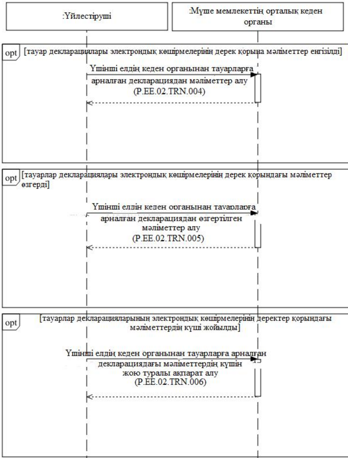
3-сурет. Тауарларға арналған декларациялардан мәліметтер алу кезінде жалпы процестің транзакцияларын орындау схемасы
