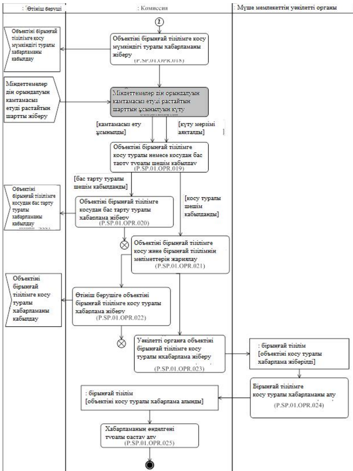
6-сурет. P.SP.01.OPR.018 – P.SP.01.OPR.025 операциялары үшін "Зияткерлік меншік объектілерін бірінғай тізілімге қосу" (P.SP.01.PRC.001) рәсімін орындау схемасы
