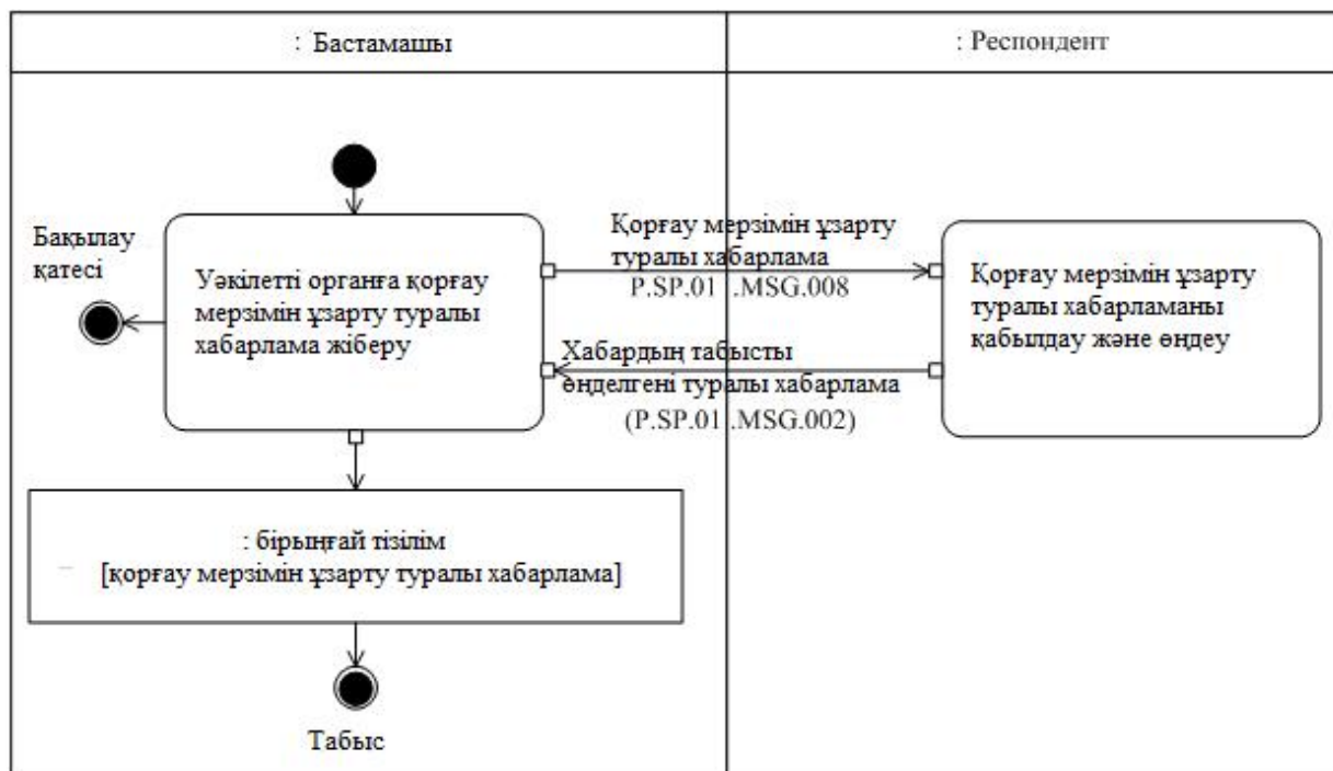
10-сурет. "Қорғау мерзімін ұзарту туралы хабарлама жіберу" (P.SP.01.TRN.007) ортақ процесс транзакциясын орындау схемасы 11-кесте
