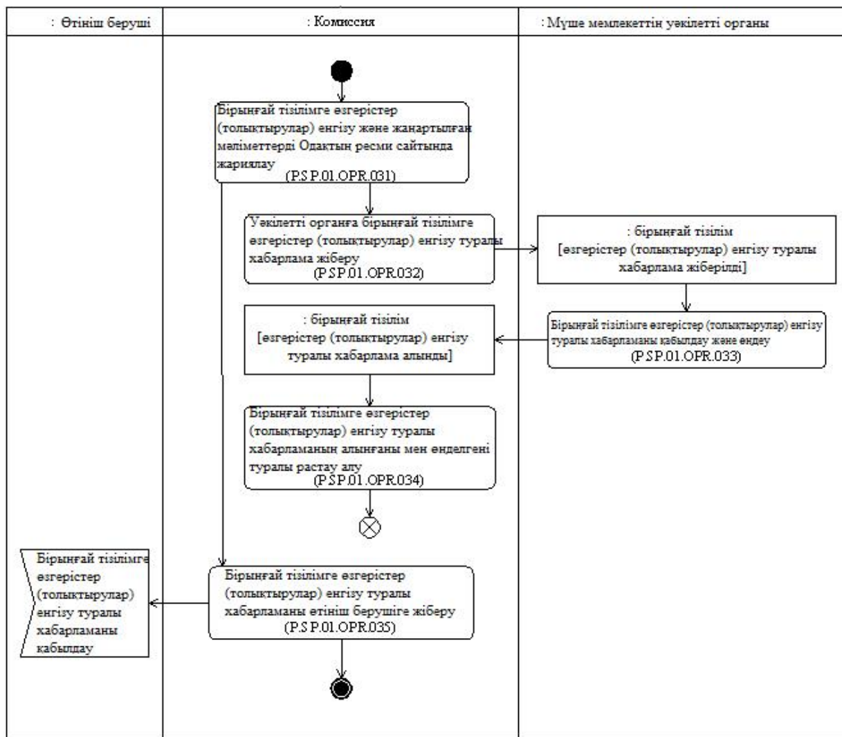
8-сурет. "Бірыңғай тізілімге өзгерістер (толықтырулар) енгізу" (P.SP.01.PRC.003) рәсімін орындау схемасы
