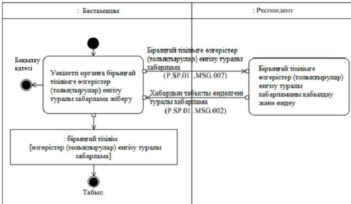
9-сурет. "Бірыңғай тізілімге өзгерістер (толықтырулар) енгізу туралы хабарлама жіберу" (P.SP.01.TRN.006) ортақ процесс транзакциясын орындау схемасы 10-кесте
