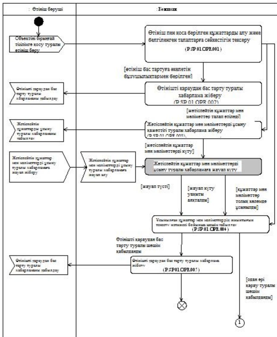
4-сурет. P.SP.01.OPR.001 – P.SP.01.OPR.005 операциялары үшін "Зияткерлік меншік объектілерін бірыңғай тізілімге қосу" (P.SP.01.PRC.001) рәсімін орындау схемасы
