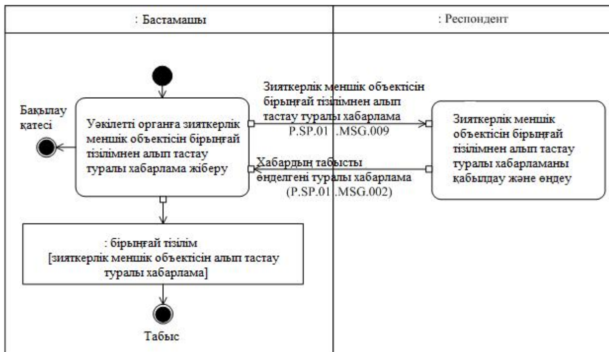
11-сурет. "Объектіні алып тастау туралы хабарлама жіберу" (P.SP.01.TRN.008) ортақ процесс транзакциясын орындау схемасы 12-кесте
