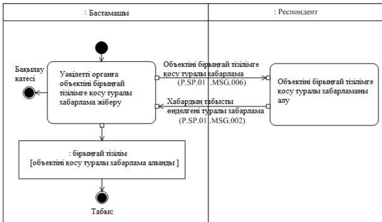
8-сурет. "Объектіні бірыңғай тізілімге қосу туралы хабарлама жіберу" (P.SP.01.TRN.005) ортақ процесс транзакциясын орындау схемасы 9-кесте
