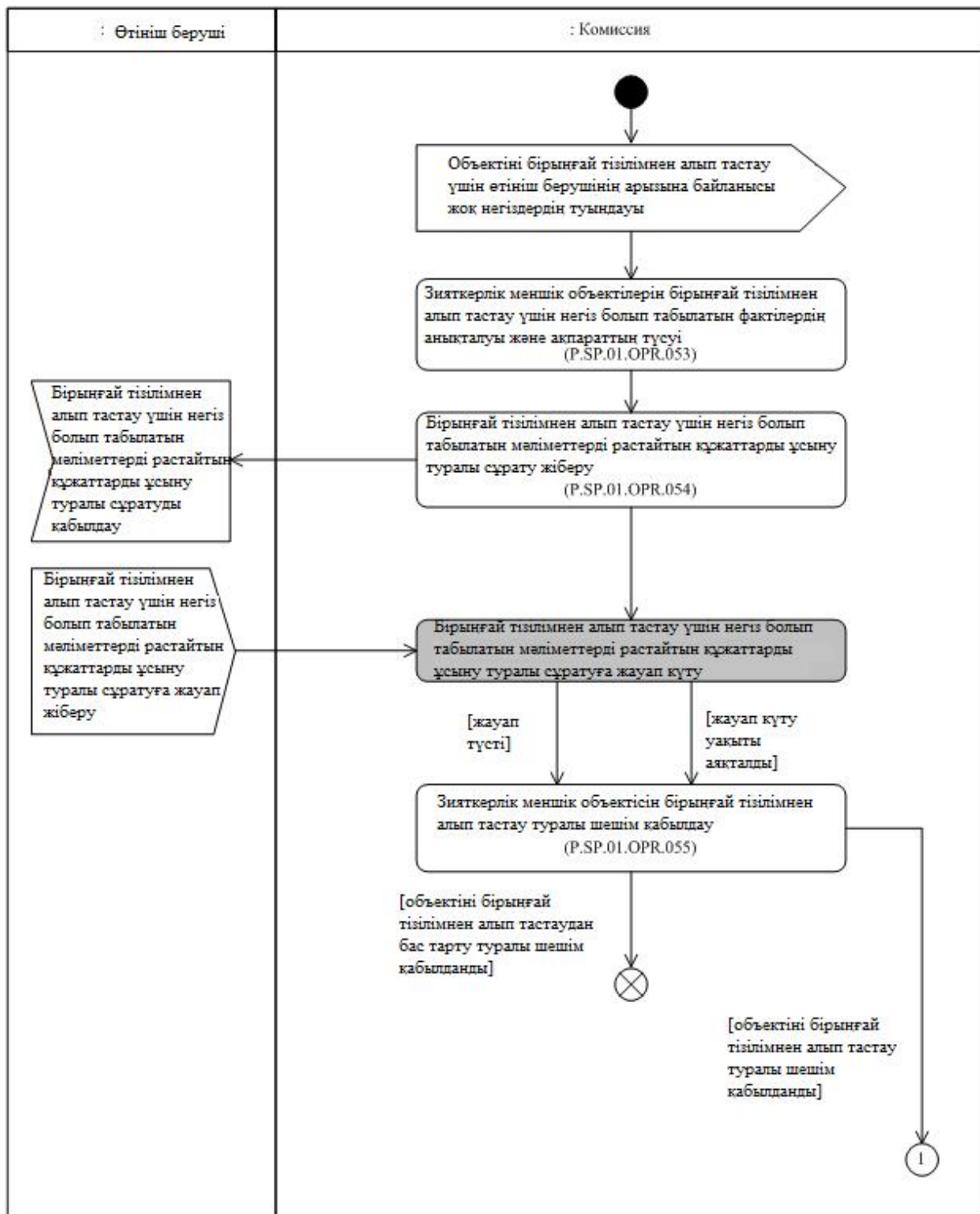
12-сурет. P.SP.01.OPR.053 – P.SP.01.OPR.055 операциялары үшін "Өтініш берушінің арызына байланысы жоқ негіздер туындаған кезде зияткерлік меншік объектілерін бірыңғай тізілімнен алып тастау" (P.SP.01.PRC.006) рәсімін орындау схемасы
