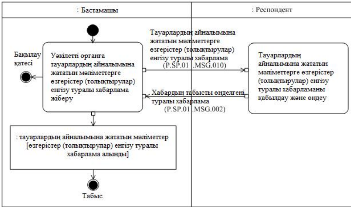
12-сурет. "Тауарлардың айналымына жататын мәліметтерге өзгерістер (толықтырулар) енгізу туралы хабарлама жіберу" (P.SP.01.TRN.009) ортақ процесс транзакциясын орындау схемасы
