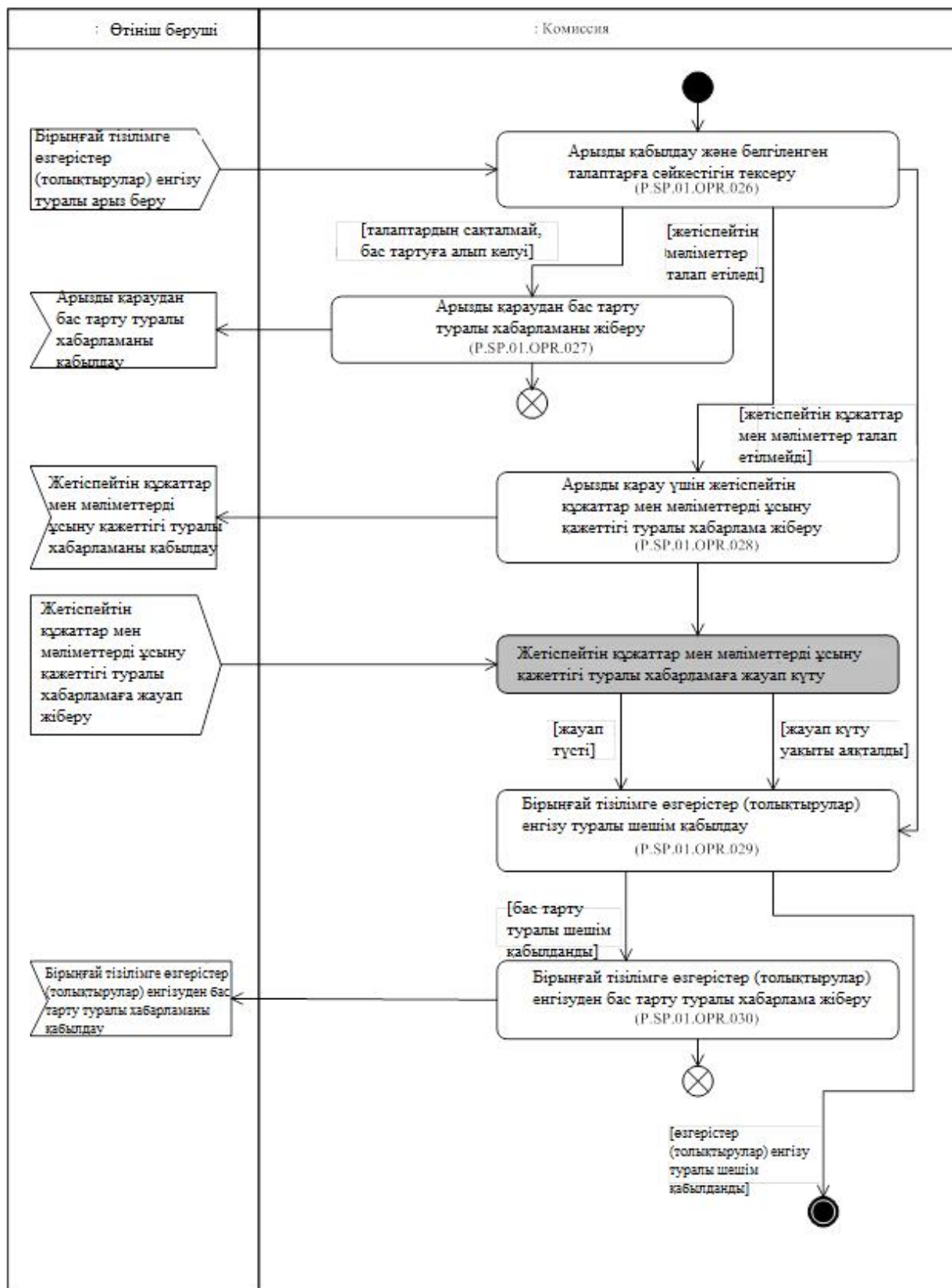
7-сурет. "Өтініш берушінің бірыңғай тізілімге өзгерістер (толықтырулар) енгізу туралы арызын қарау" (P.SP.01.PRC.002) рәсімін орындау схемасы
