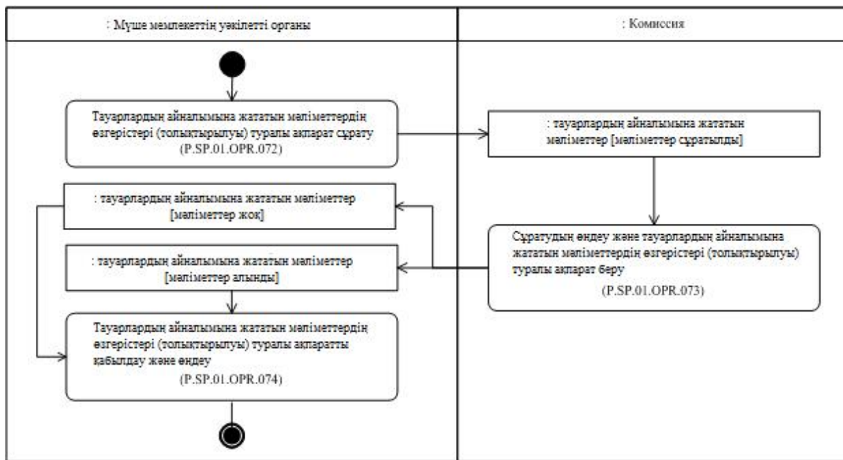
17-сурет. "Тауарлардың айналымына жататын мәліметтердің өзгерістері (толықтырылуы) туралы ақпарат алу" (P.SP.01.PRC.010) рәсімін орындау схемасы
