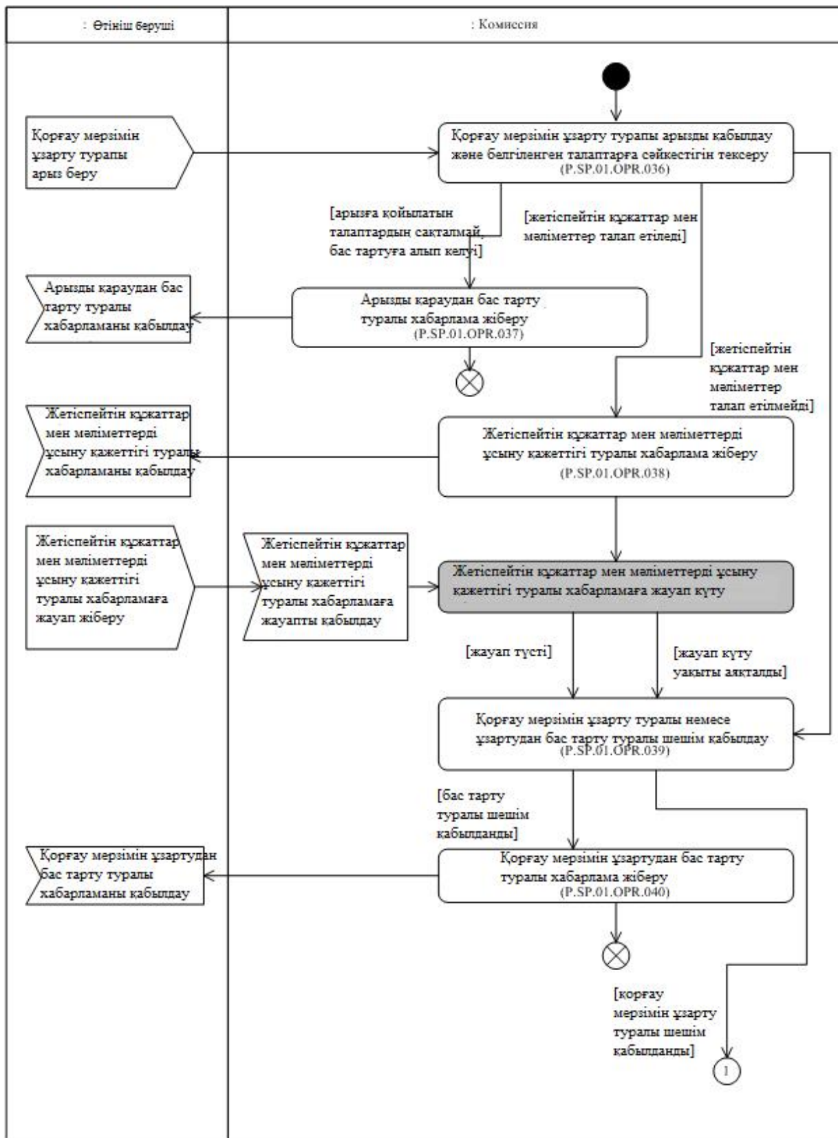
9-сурет. P.SP.01.OPR.036 – P.SP.01.OPR.040 операциялары үшін "Қорғау мерзімін ұзарту" (P.SP.01.PRC.004) рәсімін орындау схемасы
