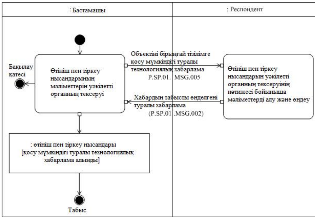
7-сурет. "Зияткерлік меншік объектісін бірыңғай тізілімге қосу мүмкіндігі туралы ақпарат беру" (P.SP.01.TRN.004) ортақ процесс транзакциясын орындау схемасы 8-кесте
