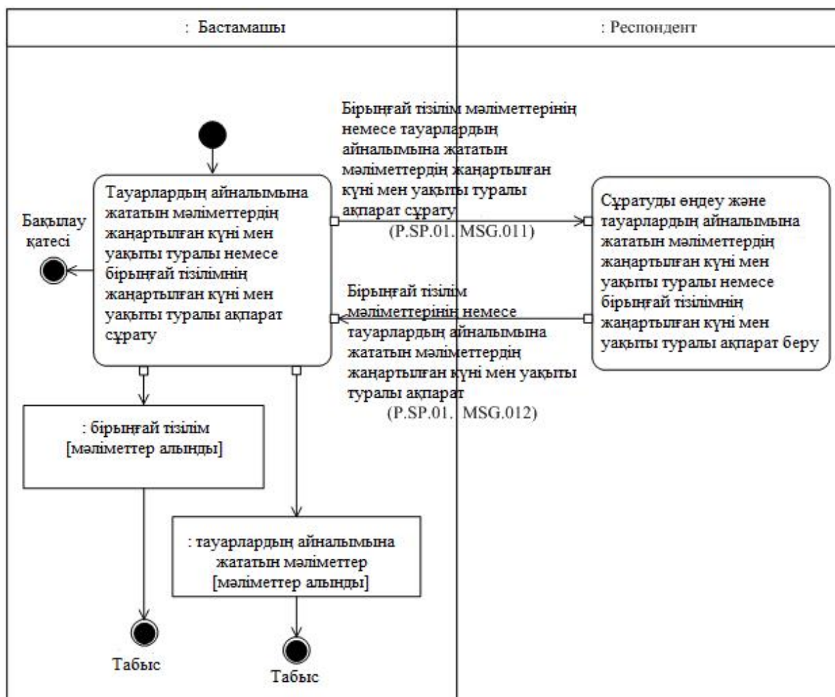
13-сурет. "Тауарлардың айналымына жататын мәліметтердің жаңартылған күні мен уақыты туралы немесе бірыңғай тізілімнің жаңартылған күні мен уақыты туралы ақпарат алу" (P.SP.01.TRN.010) ортақ процесс транзакциясын орындау схемасы 14-кесте
