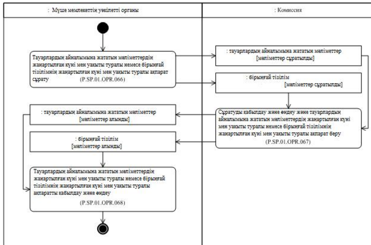
15-сурет. "Тауарлардың айналымына жататын мәліметтердің жаңартылған күні мен уақыты туралы немесе бірыңғай тізілімнің жаңартылған күні мен уақыты туралы ақпарат алу" (P.SP.01.PRC.008) рәсімін орындау схемасы
