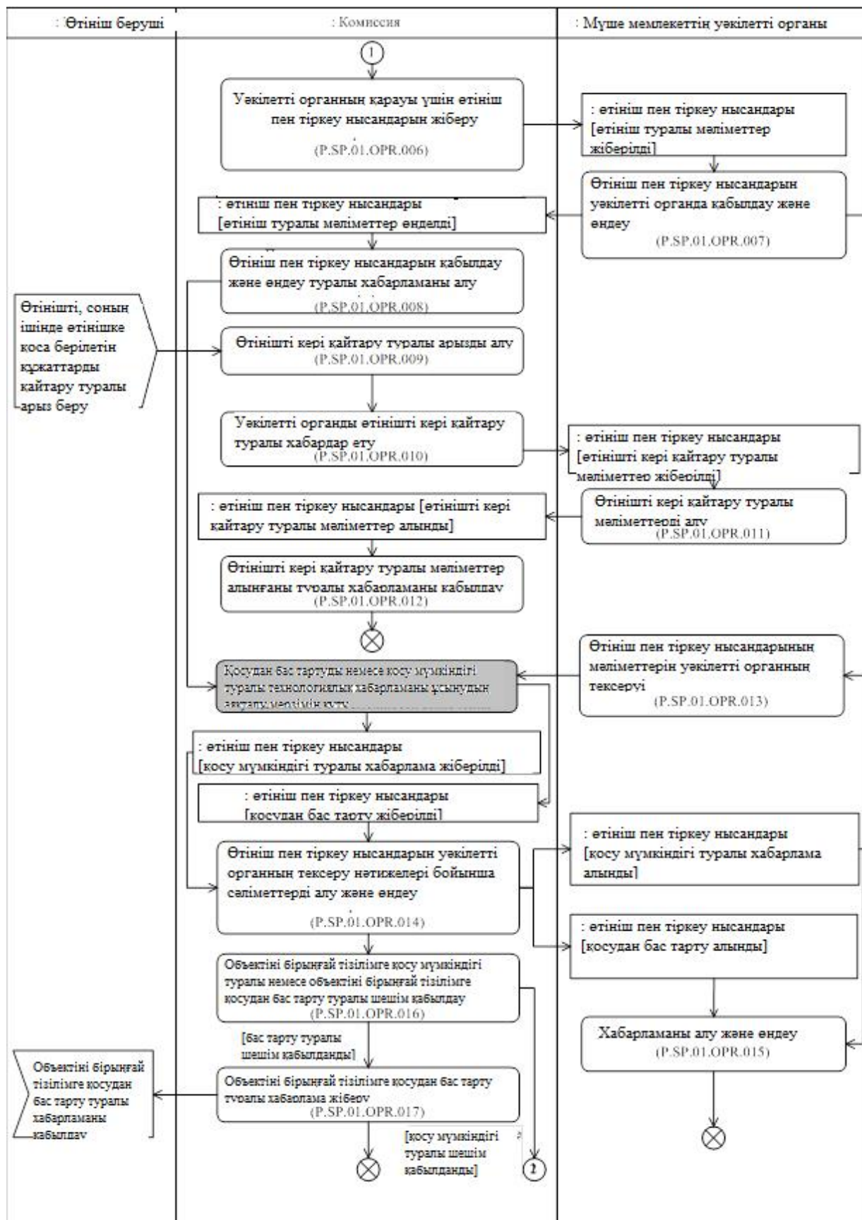
5-сурет. P.SP.01.OPR.006 – P.SP.01.OPR.017 операциялары үшін "Зияткерлік меншік объектілерін бірінғай тізілімге қосу" (P.SP.01.PRC.001) рәсімін орындау схемасы
