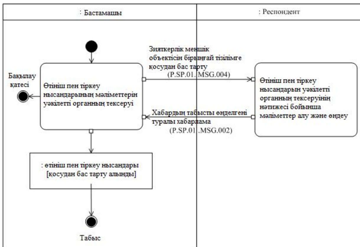
6-сурет. "Зияткерлік меншік объектісін бірыңғай тізілімге қосудан тас тарту туралы ақпарат беру" (P.SP.01.TRN.003) ортақ процесс транзакциясын орындау схемасы 7-кесте
