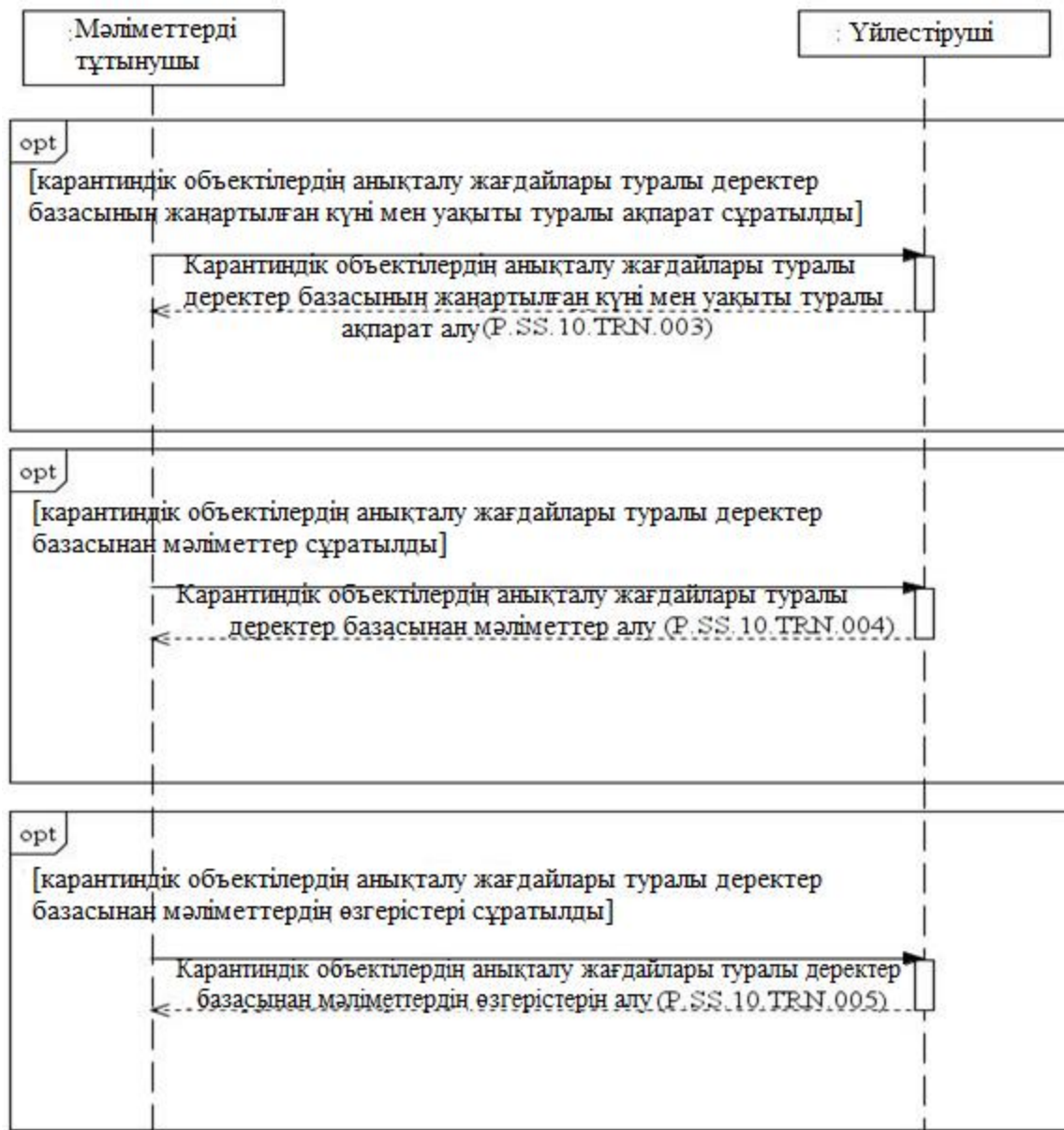
3-сурет. Карантиндік объектілердің анықталу жағдайлары туралы деректер базасынан мәліметтер алу кезінде ортақ процесс транзакцияларын орындау схемасы 3-кесте
