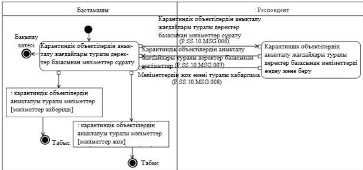
8-сурет. "Карантиндік объектілердің анықталу жағдайлары туралы деректер базасынан мәліметтер алу" (P.SS.10.TRN.004) ортақ процесс транзакциясын орындау схемасы
