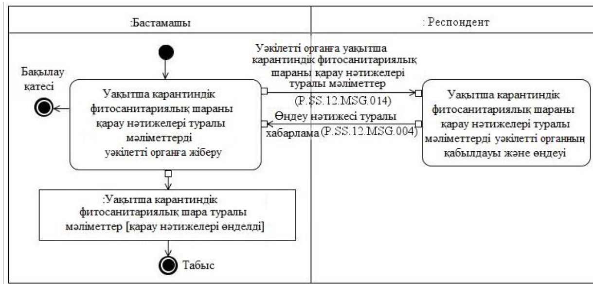
8-сурет. "Уақытша карантиндік фитосанитариялық шараны қарау нәтижелері туралы мәліметтерді уәкілетті органға ұсыну" жалпы процестің транзакциясын орындаудың схемасы (P.SS.12.TRN.011)
