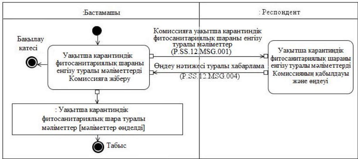
6-сурет. "Уақытша карантиндік фитосанитариялық шараны енгізу туралы мәліметтерді Комиссияға ұсыну" жалпы процестің транзакциясын орындаудың схемасы (P.SS.12.TRN.001)
