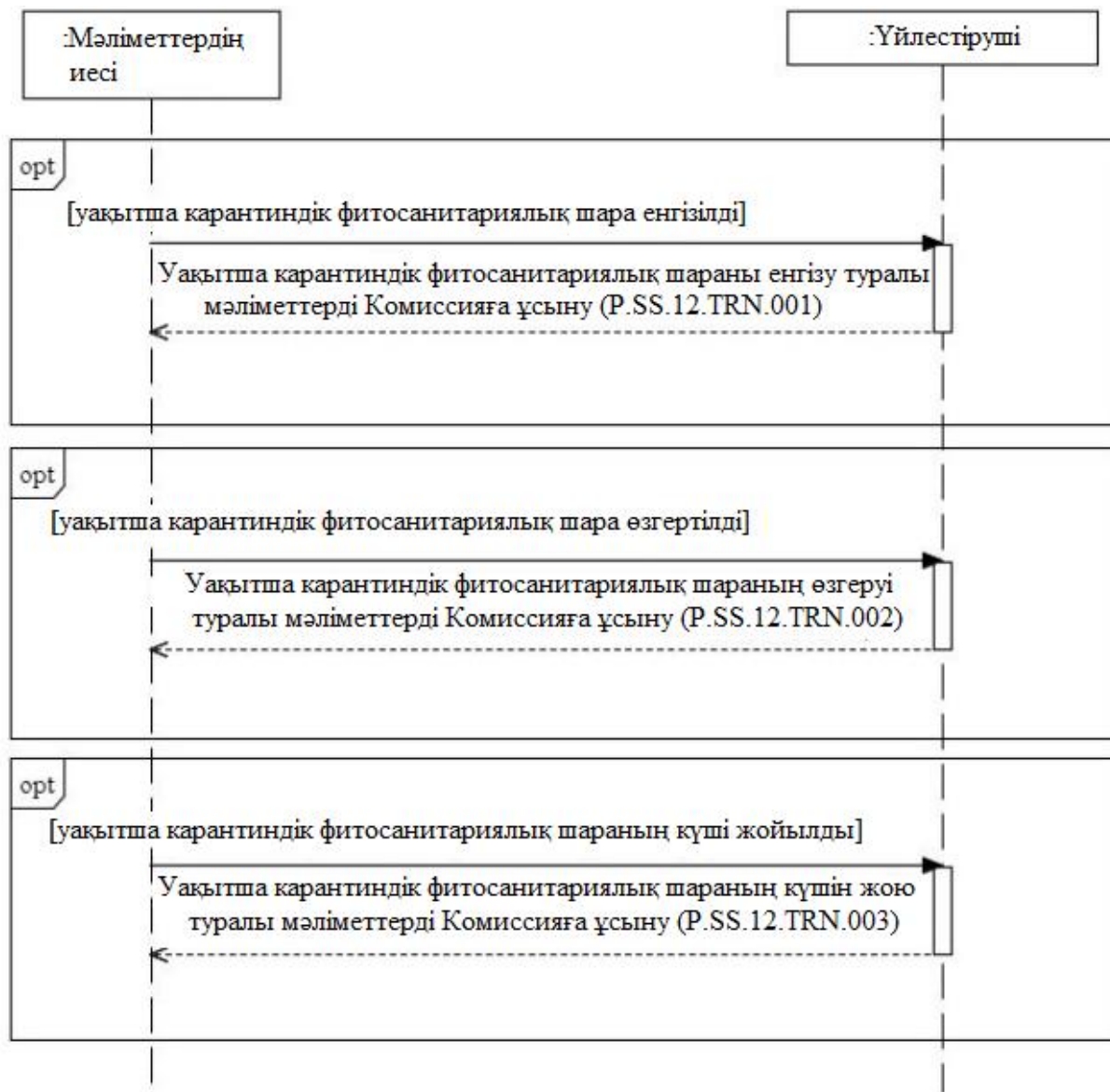
2-сурет. Уақытша карантиндік фитосанитариялық шара туралы мәліметтерді Комиссияға ұсыну кезіндегі жалпы процесс транзакциясын орындаудың схемасы 2-кесте
