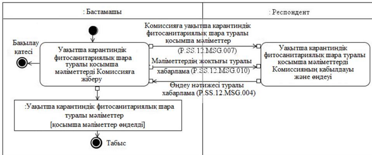
11-сурет. "Уақытша карантиндік фитосанитариялық шара туралы қосымша мәліметтерді Комиссияға беру" жалпы процесс транзакциясын орындаудың схемасы ( P.SS.12.TRN.006)
