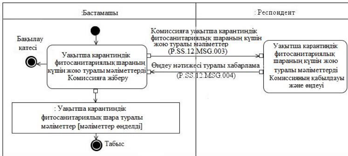
8-сурет. "Уақытша карантиндік фитосанитариялық шараның күшін жою туралы мәліметтерді Комиссияға ұсыну" жалпы процесс транзакциясын орындаудың схемасы ( P.SS.12.TRN.003)
