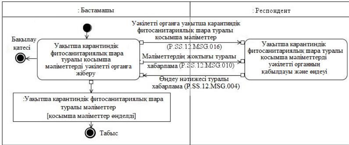
10-сурет. "Уақытша карантиндік фитосанитариялық шара туралы қосымша мәліметтерді уәкілетті органға беру" жалпы процесс транзакциясын орындаудың схемасы (P.SS.12.TRN.013)
