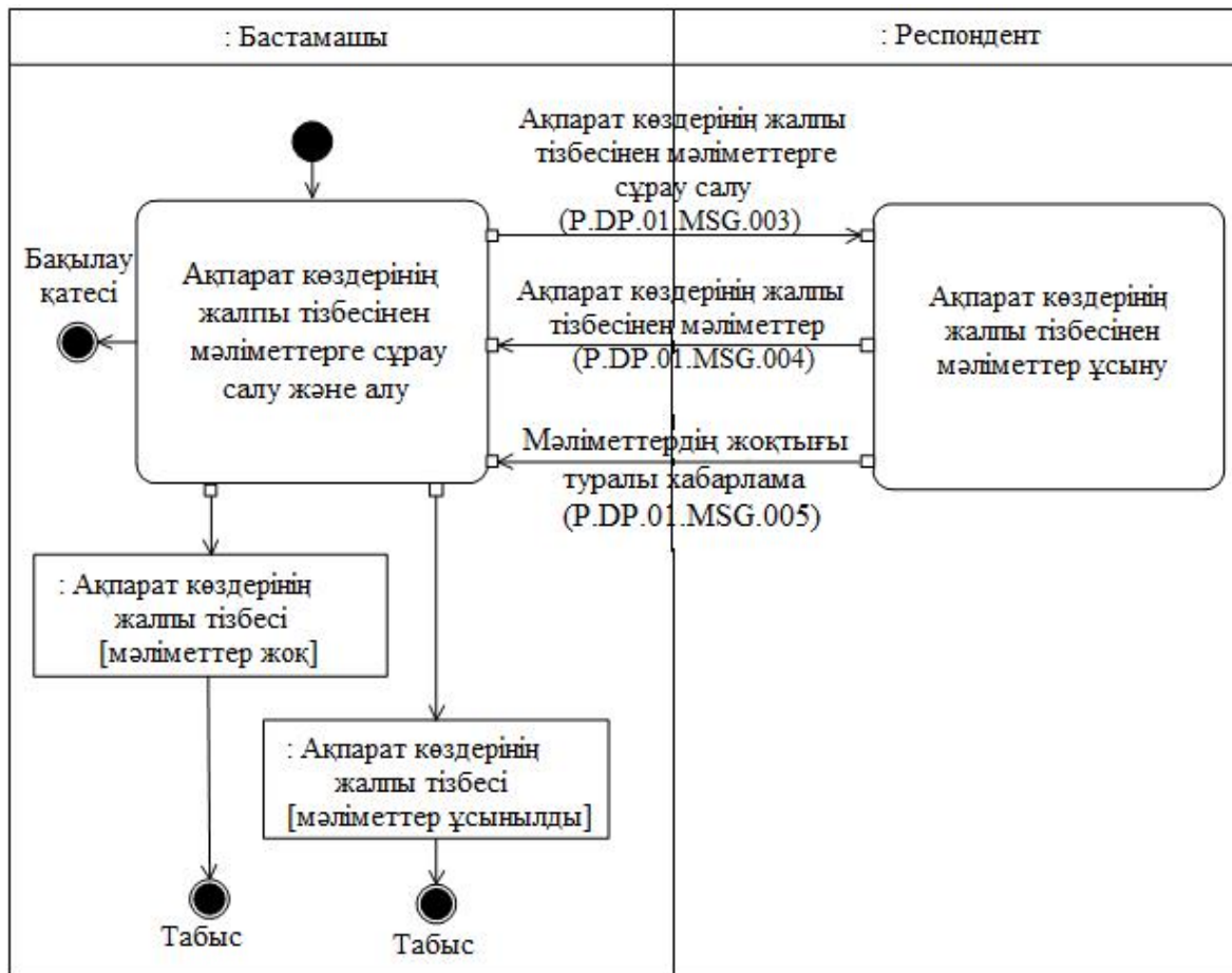
5-сурет. "Ақпарат көздерінің жалпы тізбесінен мәліметтер алу" (P.DP.01.TRN.002) жалпы процесс транзакциясының орындалу схемасы 6-кесте
