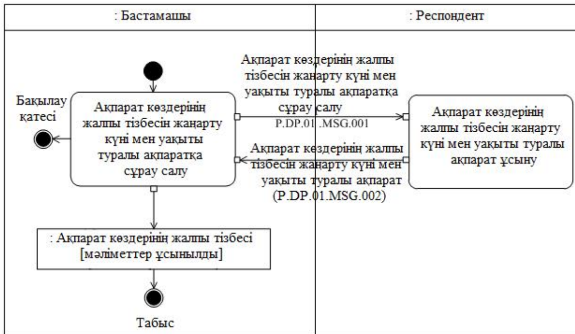
4-сурет. "Ақпарат көздерінің жалпы тізбесін жаңарту күні мен уақыты туралы ақпарат алу" (P.DP.01.TRN.001) жалпы процесс транзакциясының орындалу схемасы 5-кесте
