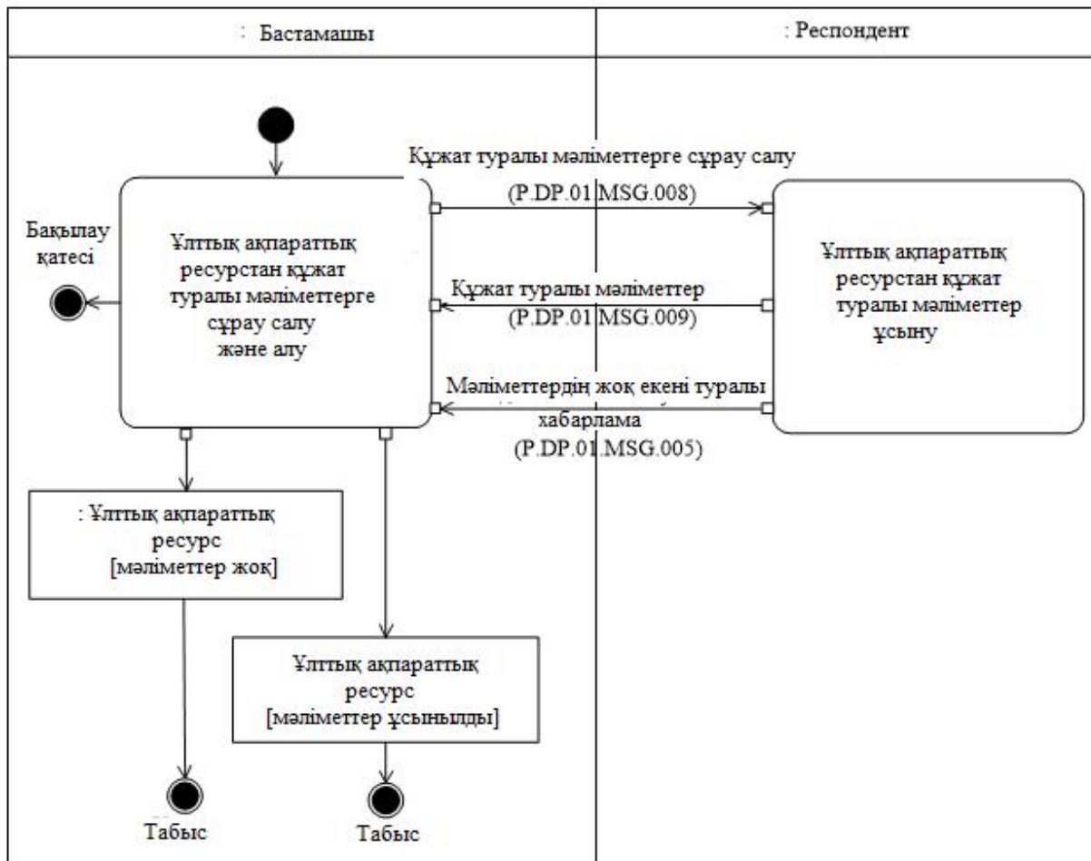
3-сурет. "Ұлттық ақпараттық ресурстан құжат туралы мәліметтер алу" жалпы процесс транзакциясының (P.DP.01.TRN.04) орындалу схемасы 4-кесте
