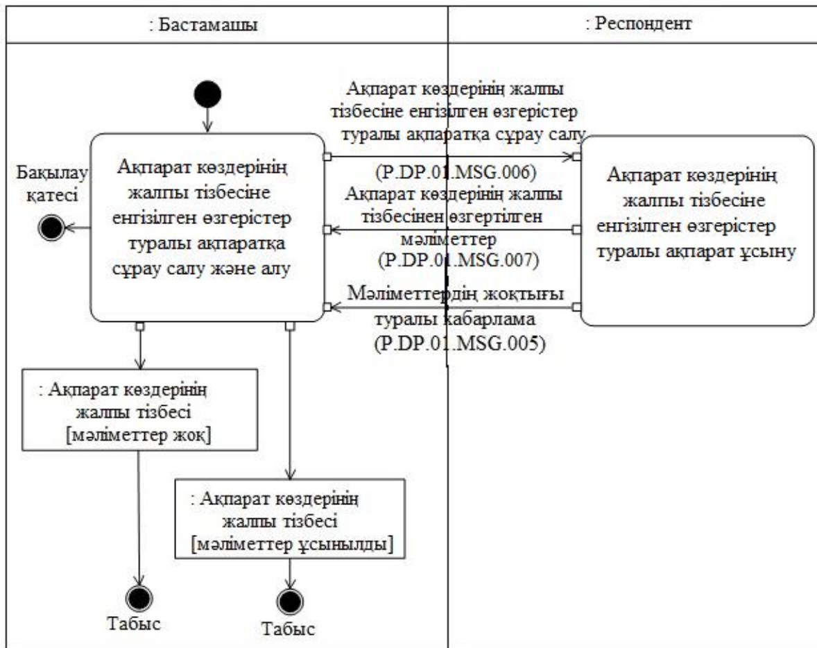
6-сурет. "Ақпарат көздерінің жалпы тізбесіне енгізілген өзгерістер туралы ақпарат алу" (P.DP.01.TRN.003) жалпы процесс транзакциясының орындалу схемасы 7-кесте
