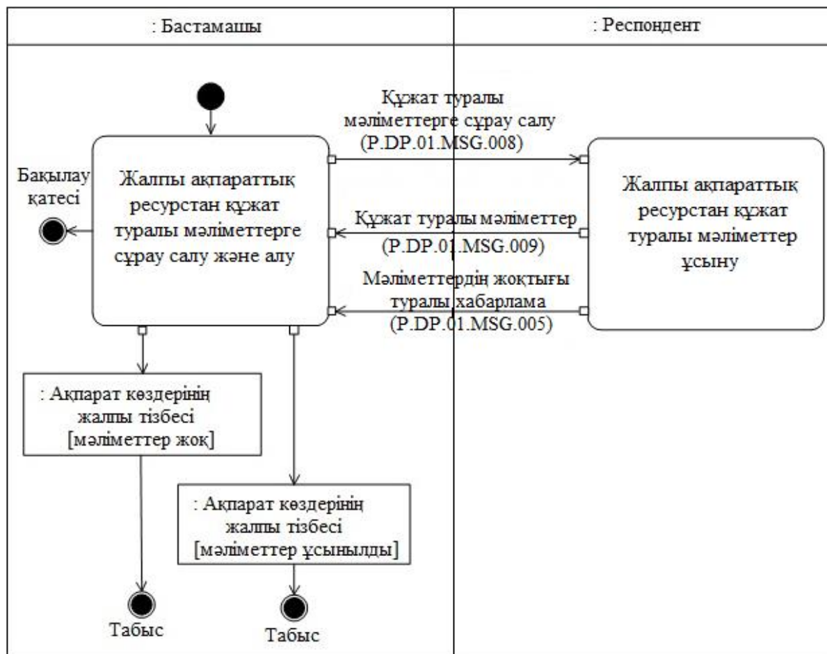
7-сурет. "Жалпы ақпараттық ресурстан құжат туралы мәліметтер алу" (P.DP.01.TRN.005) жалпы процесс транзакциясының орындалу схемасы 8-кесте
