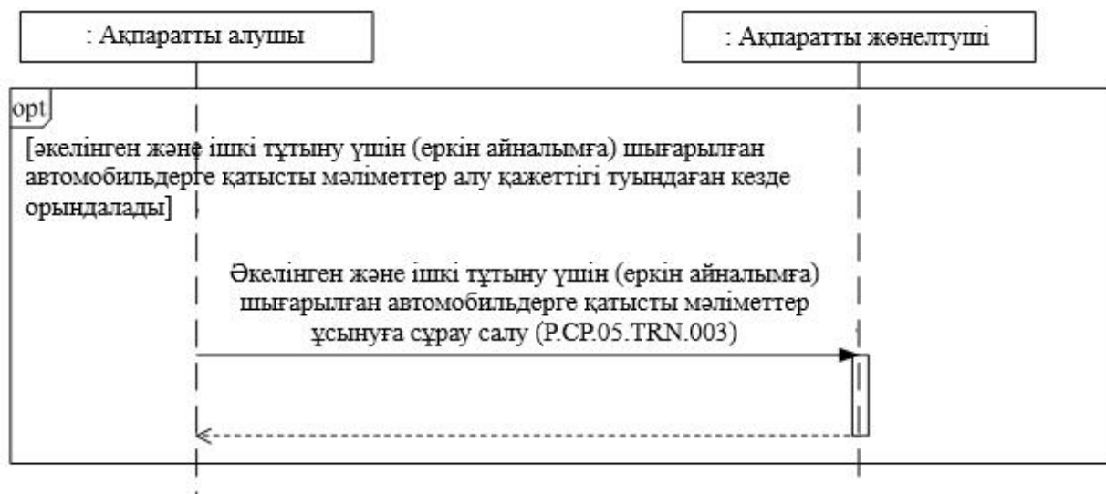
3-сурет. Мәліметтерді алатын уәкілетті органның сұрау салуы бойынша әкелінген және ішкі тұтыну үшін (еркін айналымға) шығарылған автомобильдерге қатысты мәліметтерді ұсыну кезінде жалпы процесс транзакцияларын орындау схемасы 3-кесте
