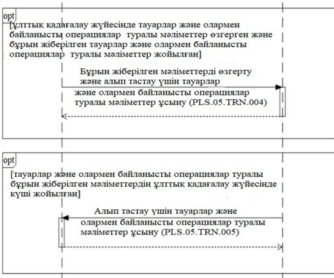
2-сурет. Тауарлар және олармен байланысты операциялар туралы мәліметтер ұсыну кезінде жалпы процесс транзакцияларын орындаудың схемасы 2-кесте
