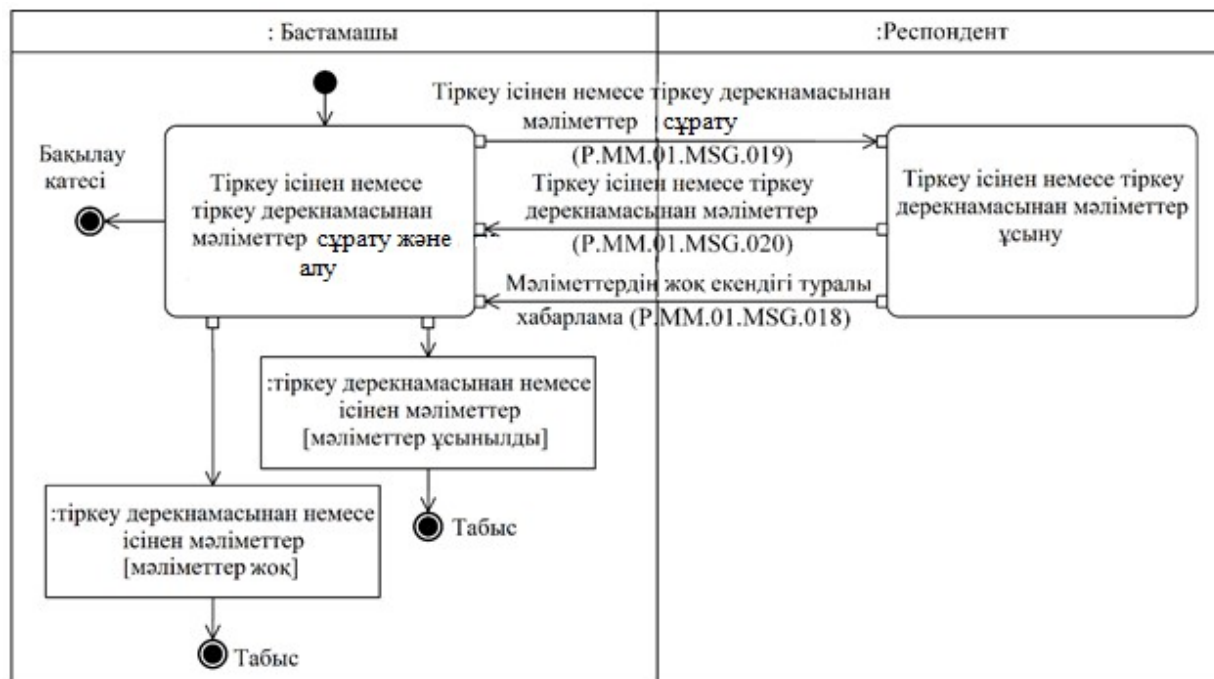
15-сурет. "Комиссияның тіркеу ісінен немесе тіркеу дерекнамасынан мәліметтер алуы" жалпы процесі транзакциясын орындау схемасы (P.MM.01.TRN.008)
