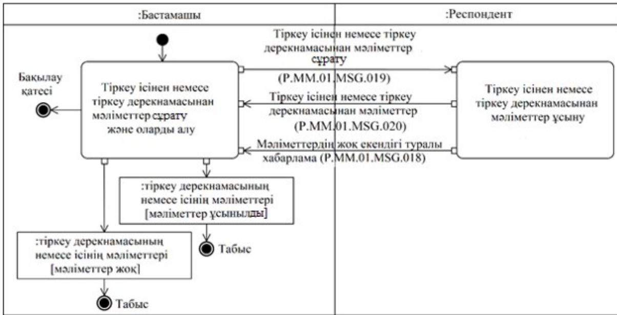
9-сурет. "Тіркеу ісінен немесе тіркеу дерекнамасынан мәліметтер алу" жалпы процесінің транзакциясын (P.MM.01.TRN.012) орындау схемасы 10-кесте
