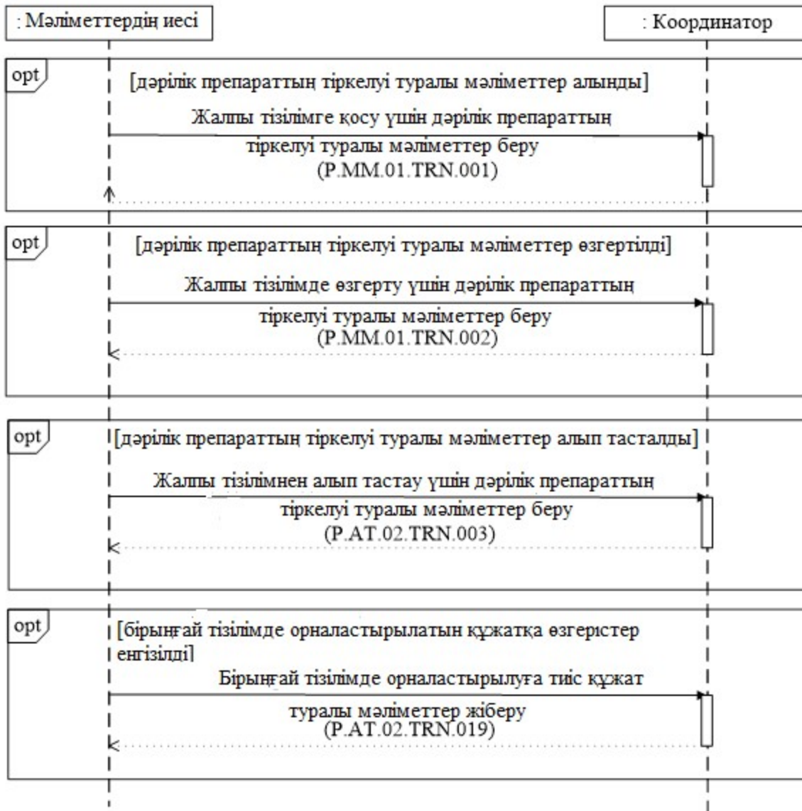
2-сурет. Жалпы тізілімді қалыптастыру және жүргізу кезінде жалпы процесс транзакцияларын орындау схемасы
