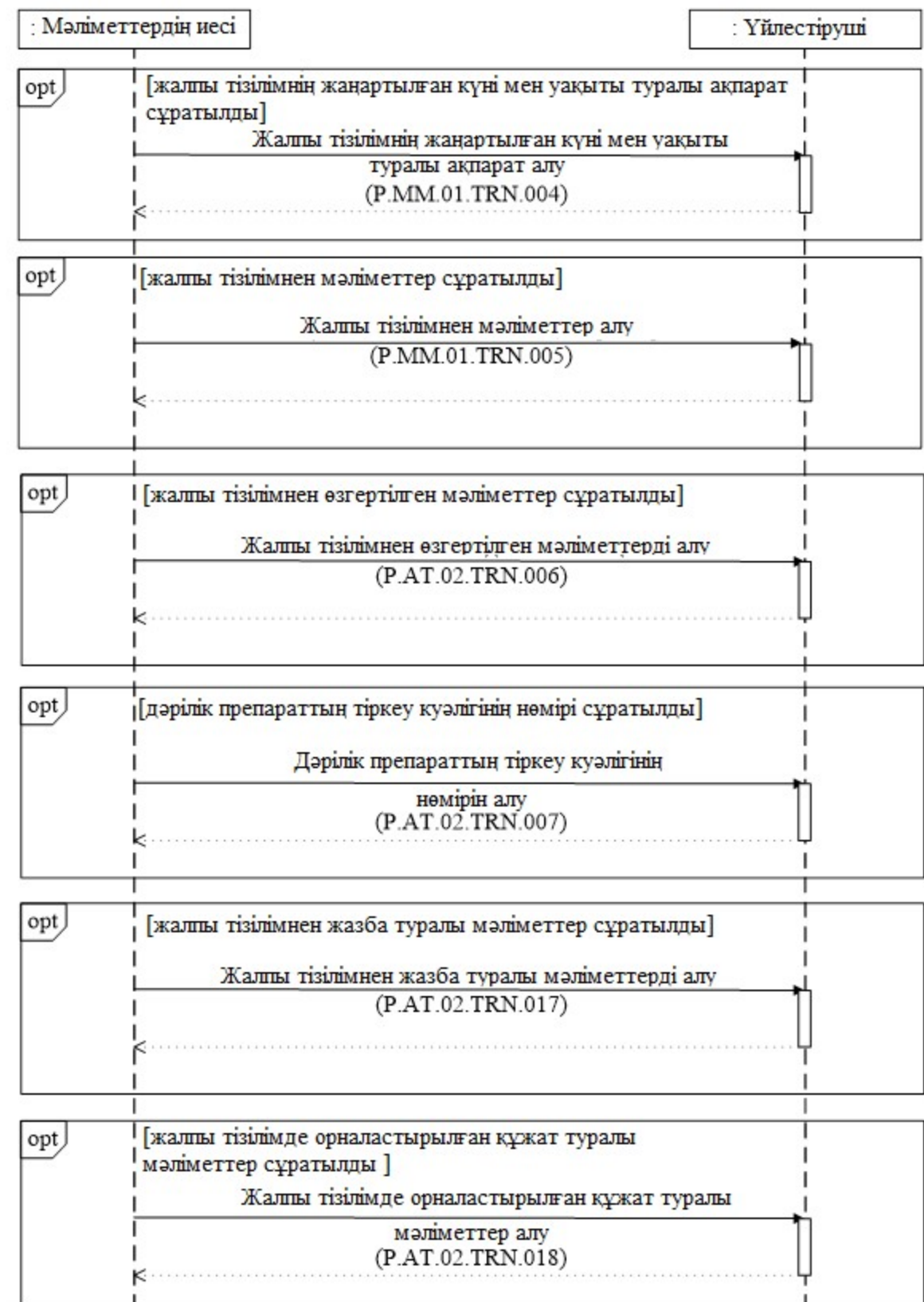
3-сурет. Жалпы тізілімнен мәліметтер алған кезде жалпы процесс транзакцияларын орындау схемасы
