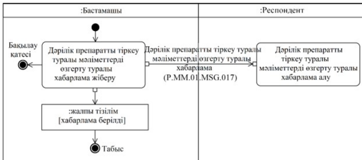
8-сурет. "Дәрілік препаратты тіркеу туралы мәліметтерді өзгерту туралы хабарлау" жалпы процесінің транзакциясын (P.MM.01.TRN.011) орындау схемасы 9-кесте
