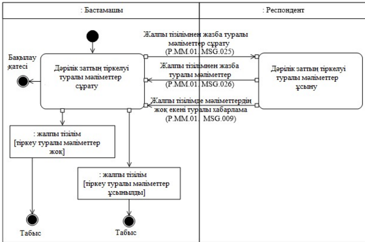
13-сурет. "Жалпы тізілімнен жазба туралы мәліметтер алу" жалпы процесінің транзакциясы (P.MM.01.TRN.017)
