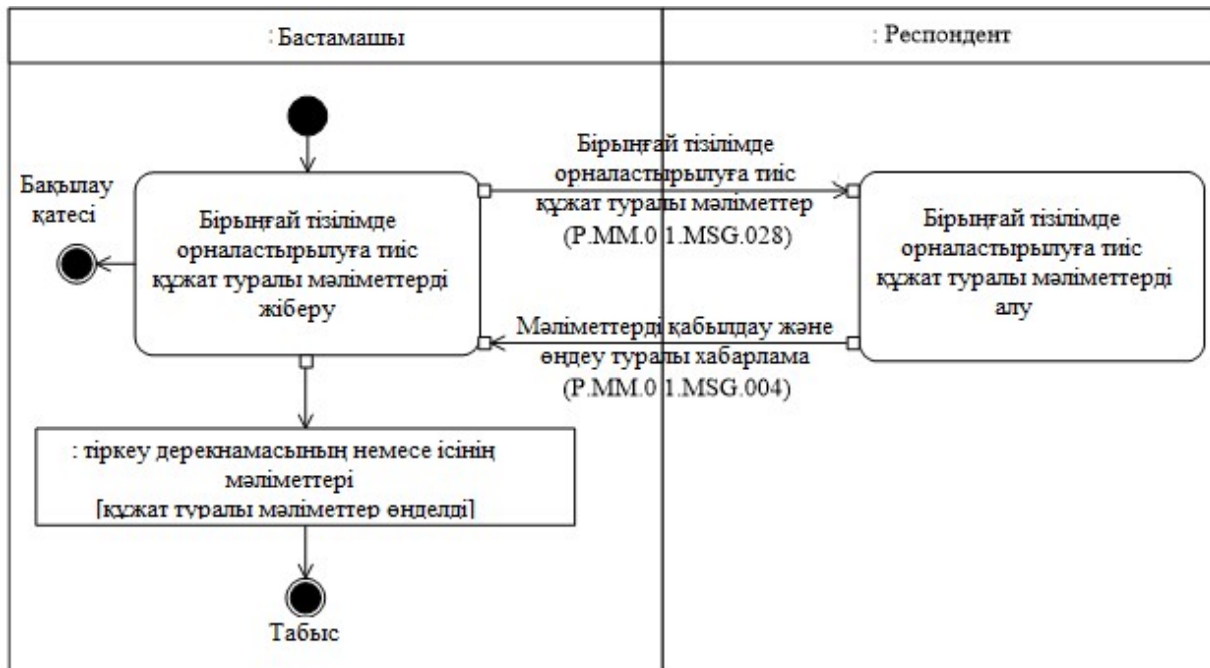
8-сурет. "Бірыңғай тізілімде орналастырылуға тиіс құжат туралы мәліметтерді жіберу" жалпы процесі транзакциясын орындау схемасы (P.MM.01.TRN.019)
