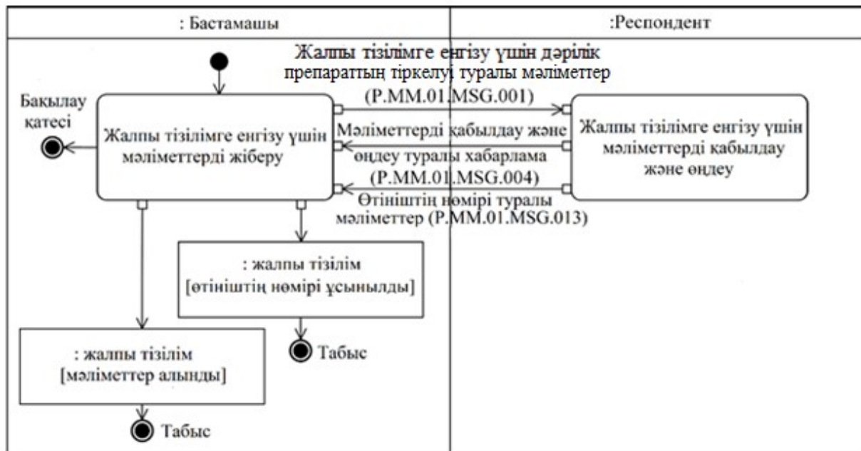
5-сурет. "Жалпы тізілімге енгізу үшін дәрілік препараттың тіркелуі туралы мәліметтер беру" жалпы процесінің транзакциясын орындау схемасы (P.MM.01.TRN.001)
