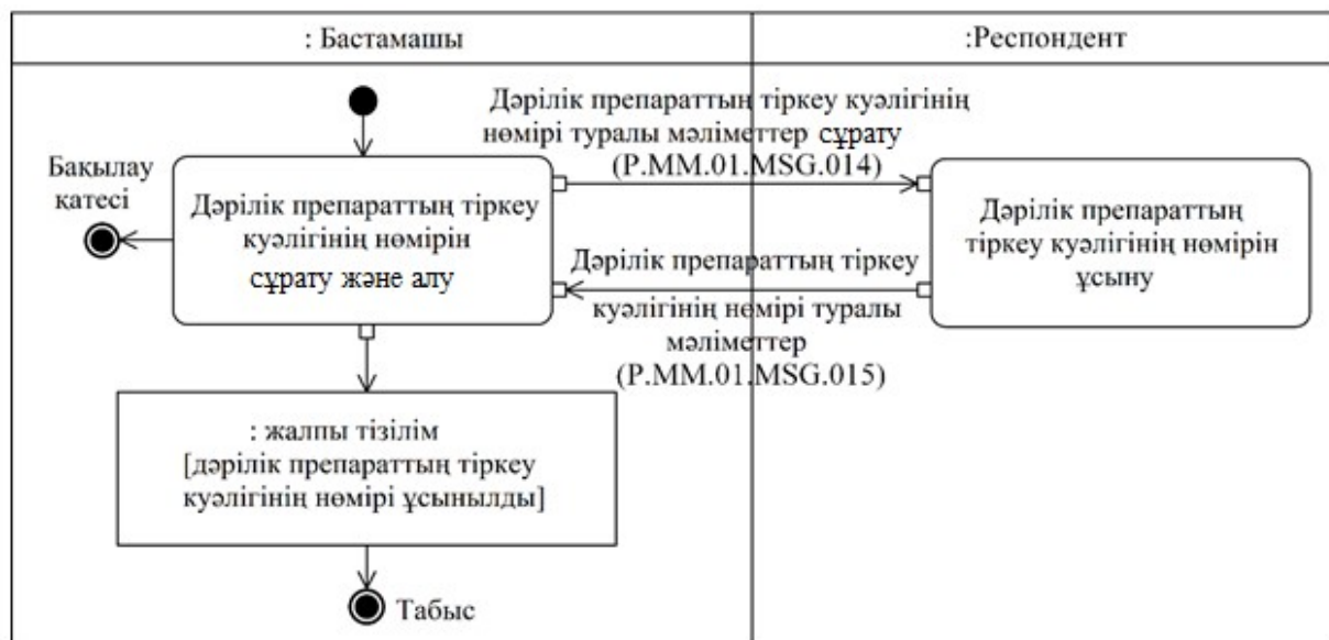
12-сурет. "Дәрілік препараттың тіркеу куәлігінің нөмірін алу" жалпы процесінің транзакциясын орындау схемасы (P.MM.01.TRN.007)
