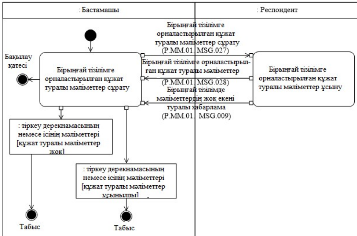
14-сурет. "Бірыңғай тізілімге орналастырылған құжат туралы мәліметтер алу" жалпы процесінің транзакциясын орындау схемасы (P.MM.01.TRN.018)
