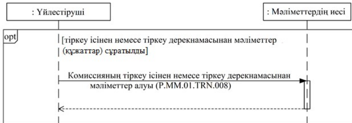
4-сурет. Комиссия тіркеу ісінде немесе тіркеу дерекнамасында бар мәліметтерді алған кездегі жалпы процесс транзакцияларын орындау схемасы 4-кесте
