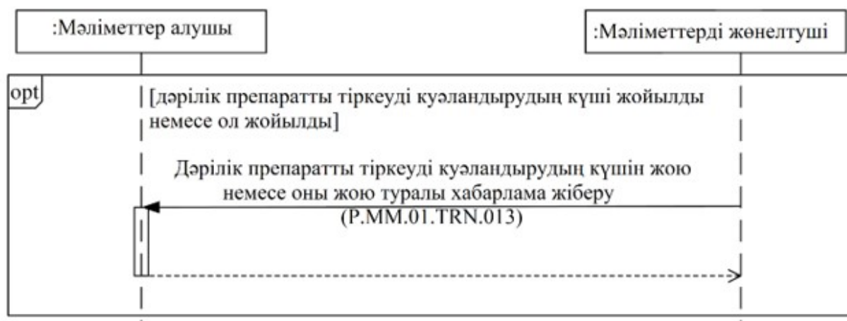
4-сурет. Дәрілік препаратты тіркеуді куәландырудың күшін жою немесе оны жою туралы хабарлаған кезде жалпы процесс транзакцияларын орындау схемасы 4-кесте
