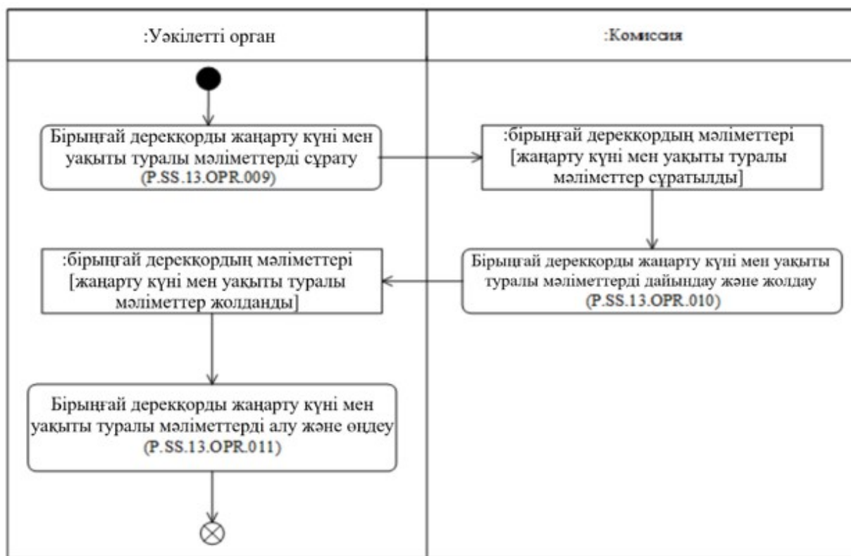
6-сурет. "Бірыңғай дерекқорды жаңарту күні мен уақыты туралы мәліметтер алу" (P.SS.13.PRC.003) рәсiмiн орындау схемасы
