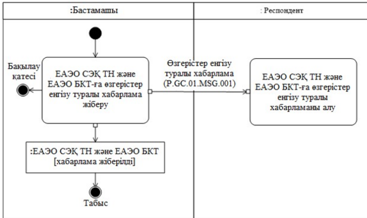
4-сурет. "ЕАЭО СЭҚ ТН және ЕАЭО БКТ-ға өзгерістер енгізу туралы хабарлама" ( P.GC.01.TRN.001) жалпы процесінің транзакциясын орындау схемасы 5-кесте
