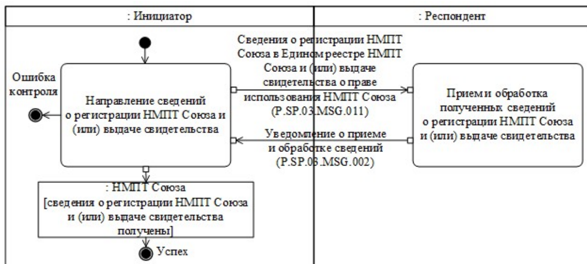
8-сурет. "Одақтың ТШЖА тіркеу және (немесе) Одақтың ТШЖА пайдалану құқығын беру туралы хабарлама" жалпы процесінің транзакциясын орындау схемасы (P.SP.03.TRN.012)
