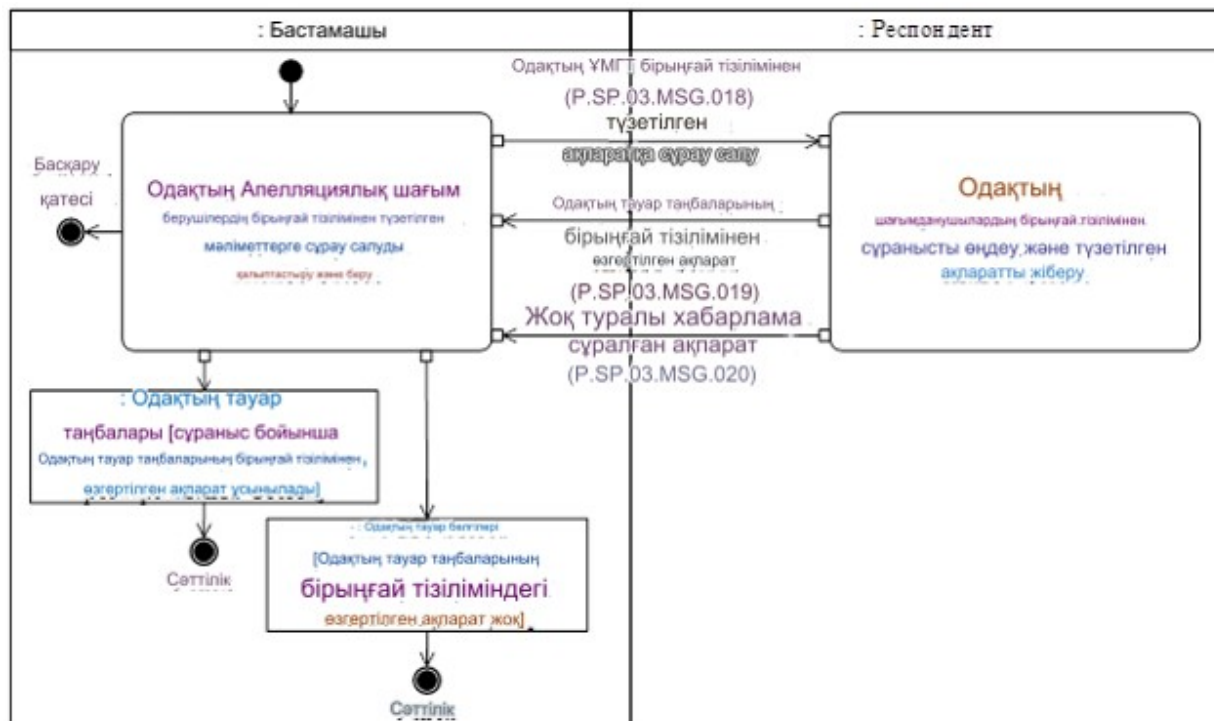
Сурет. 13. "Одақтың ТШЖА бірыңғай тізілімінде өзгертілген мәліметтерді алу" жалпы процесінің транзакциясын орындау схемасы (P. SP.03.TRN.009)
