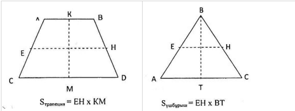
3-сурет. Трапеция мен үшбұрыштың көлемін анықтау
