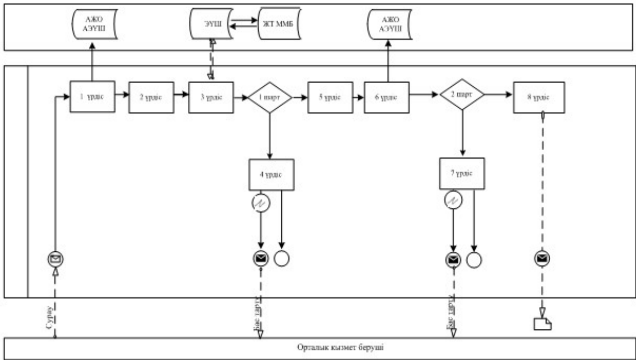
Орталық арқылы электрондық мемлекеттік қызметті көрсету кезінде функционалдық іс-қимылының № 2 диаграммасы
