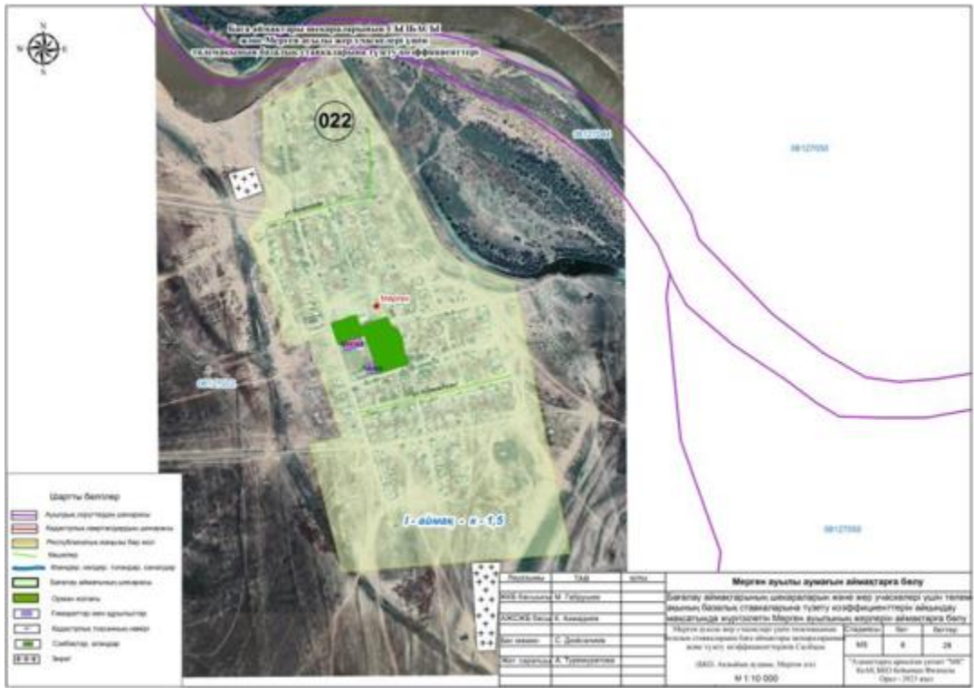
Ақжайық ауданы Мойылды ауылының жерін аймақтарға бөлу жобасы (схемасы)
