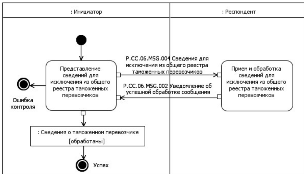
Рис. 6. Схема выполнения транзакции общего процесса "Исключение сведений из общего реестра таможенных перевозчиков" (P.СC.06.ТRN.003) Таблица 7
