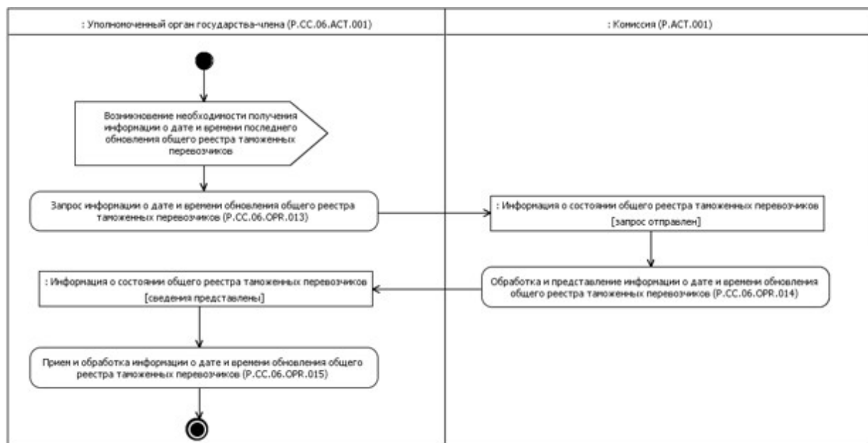
Рис. 8. Схема выполнения процедуры "Получение информации о дате и времени обновления общего реестра таможенных перевозчиков" (P.CC.06.PRC.004)
