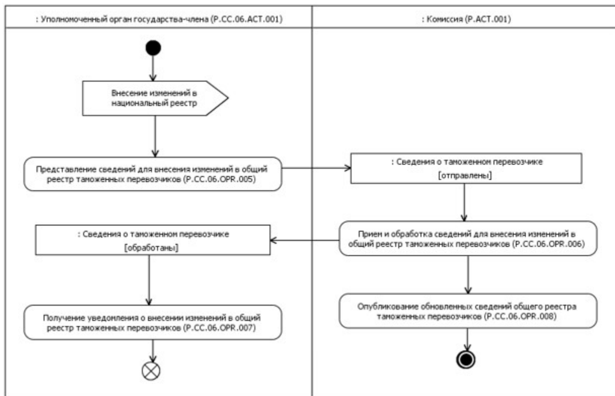
Рис. 6. Схема выполнения процедуры "Изменение сведений,
