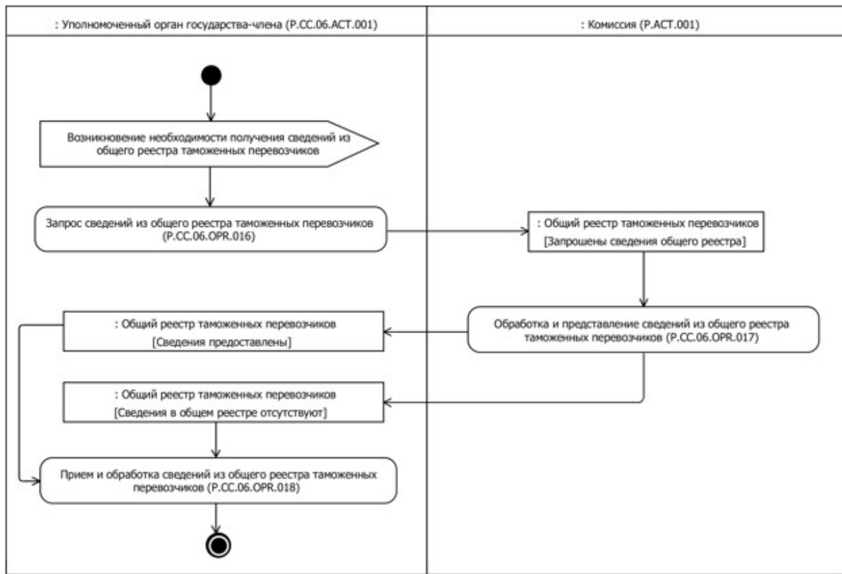
Рис. 9. Схема выполнения процедуры "Получение сведений из общего реестра таможенных перевозчиков" (P.СC.06.PRC.005)
