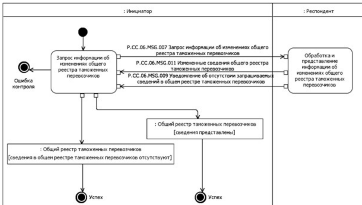
Рис. 9. Схема выполнения транзакции общего процесса "Получение информации об изменениях, внесенных в общий реестр таможенных перевозчиков" (P.СC.06.TRN.006)
