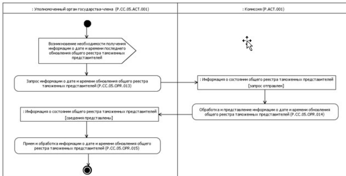
Рис. 8. Схема выполнения процедуры "Получение информации о дате и времени обновления общего реестра таможенных представителей" (P.CC.05.PRC.004)
