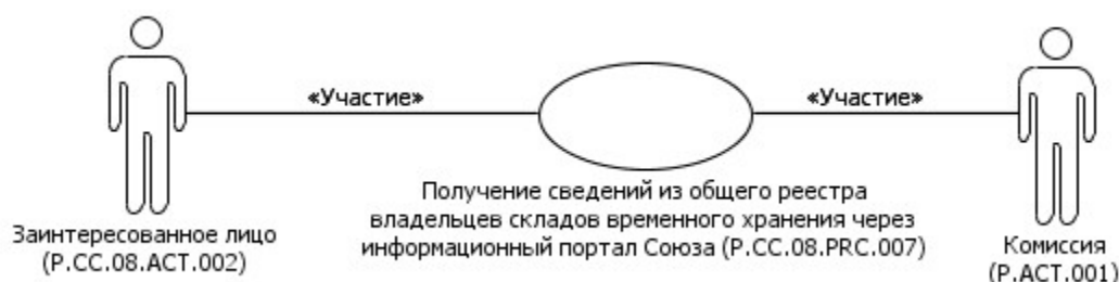
Рис. 4. Общая схема выполнения группы процедур представления заинтересованным лицам сведений, содержащихся в общем реестре владельцев складов временного хранения
