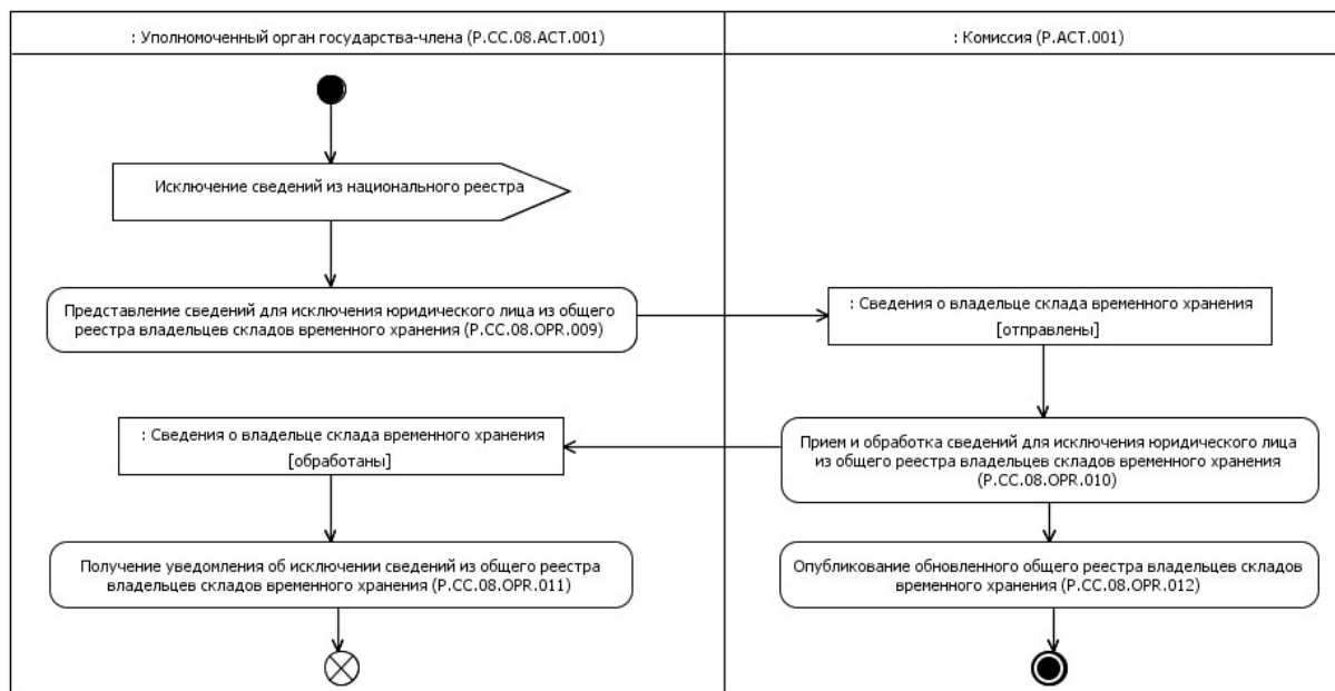
Рис. 7. Схема выполнения процедуры "Исключение сведений из общего реестра владельцев складов временного хранения" (P.СC.08.PRC.003)
