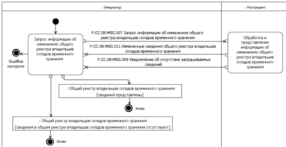
Рис. 9. Схема выполнения транзакции общего процесса "Получение информации об изменениях, внесенных в общий реестр владельцев складов временного хранения" (P.CC.08.TRN.006)
