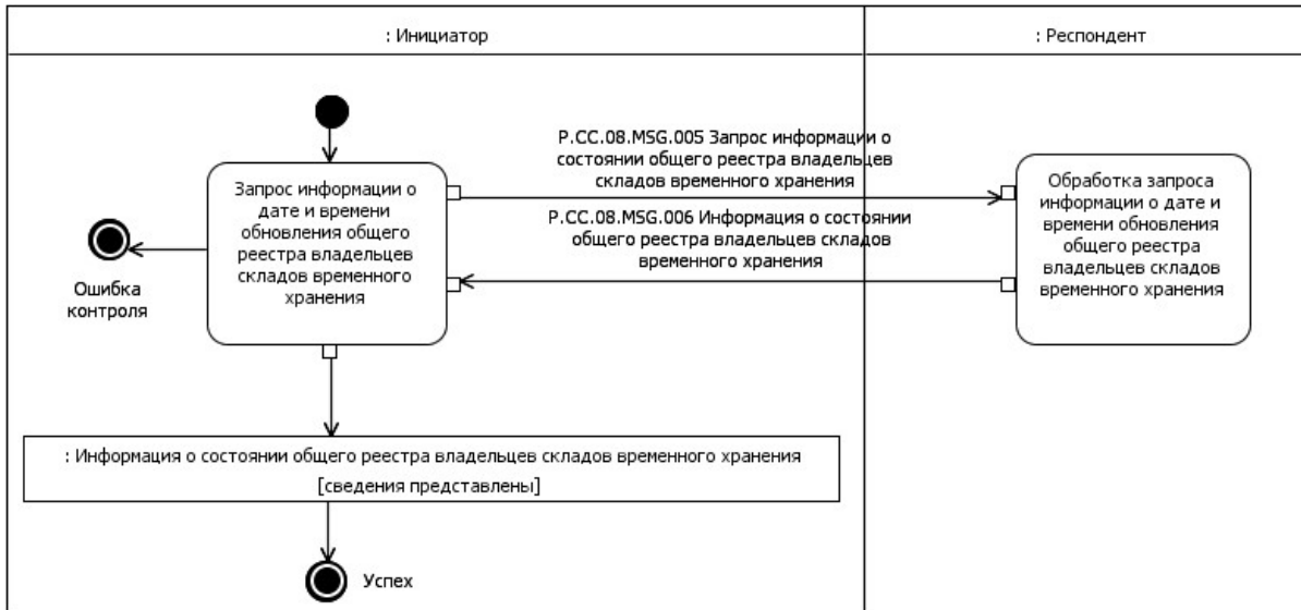
Рис. 7. Схема выполнения транзакции общего процесса "Получение информации о дате и времени обновления общего реестра владельцев складов временного хранения" (P.СC.08.TRN.004) Таблица 8
