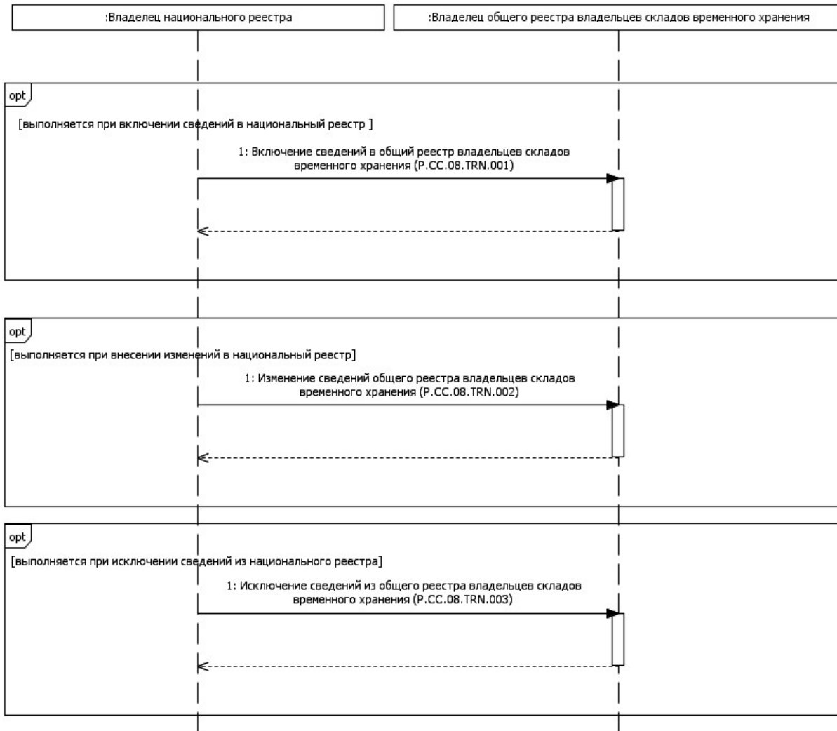
Рис. 2. Схема выполнения транзакций общего процесса при формировании и ведении общего реестра владельцев складов временного хранения
