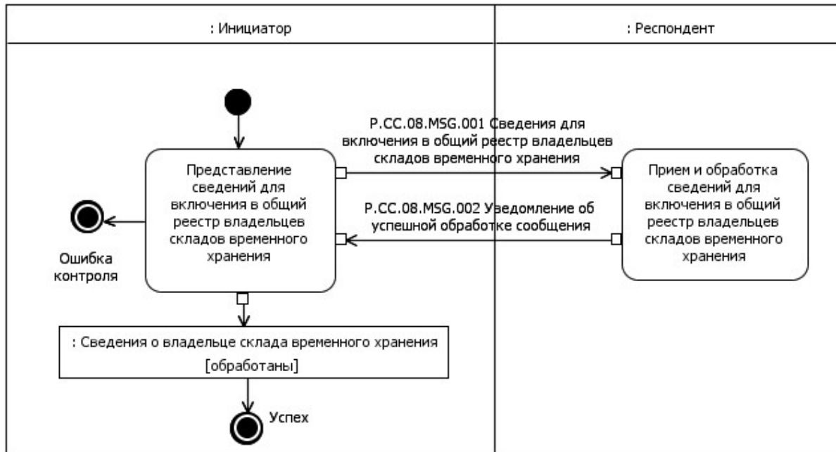
Рис. 4. Схема выполнения транзакции общего процесса "Включение сведений в общий реестр владельцев складов временного хранения" (P.СC.08.TRN.001)
