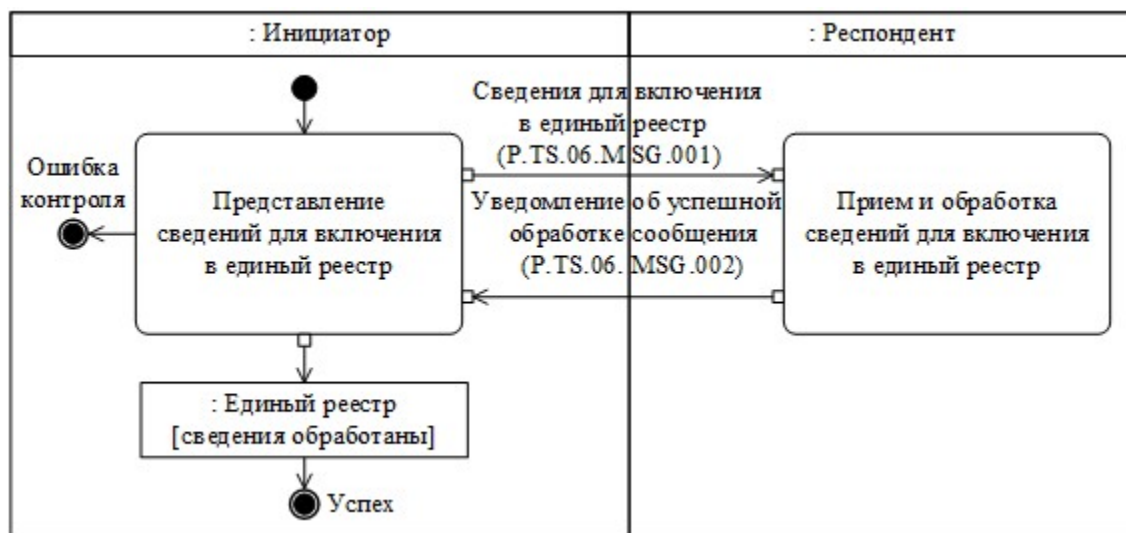
Рис. 4. Схема выполнения транзакции общего процесса "Включение сведений в единый реестр" (P.TS.06.TRN.001)
