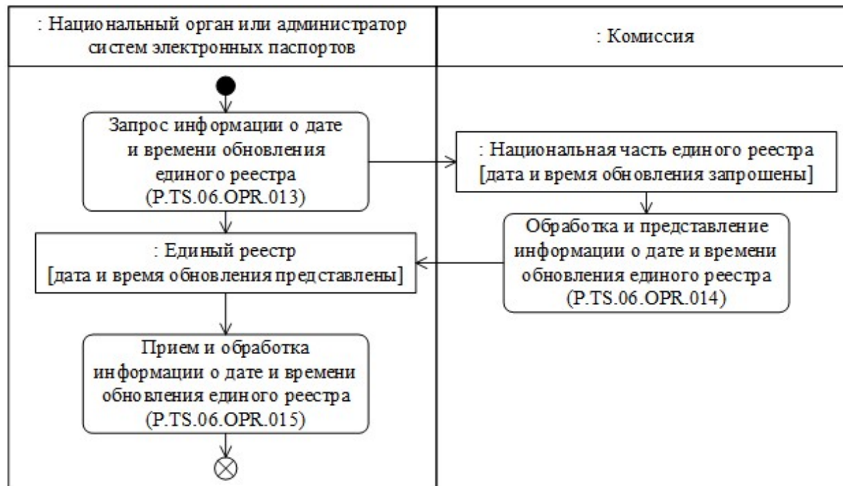
Рис. 8. Схема выполнения процедуры "Получение информации о дате и времени обновления единого реестра" (P.TS.06.PRC.004)
