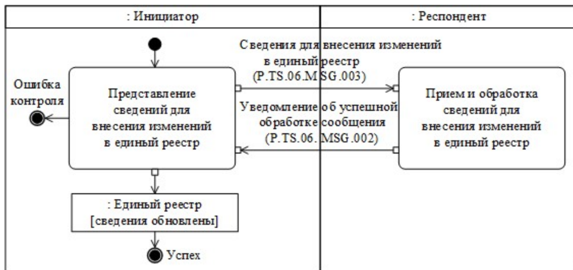
Рис. 5. Схема выполнения транзакции общего процесса "Изменение сведений единого реестра" (P.TS.06.TRN.002)
