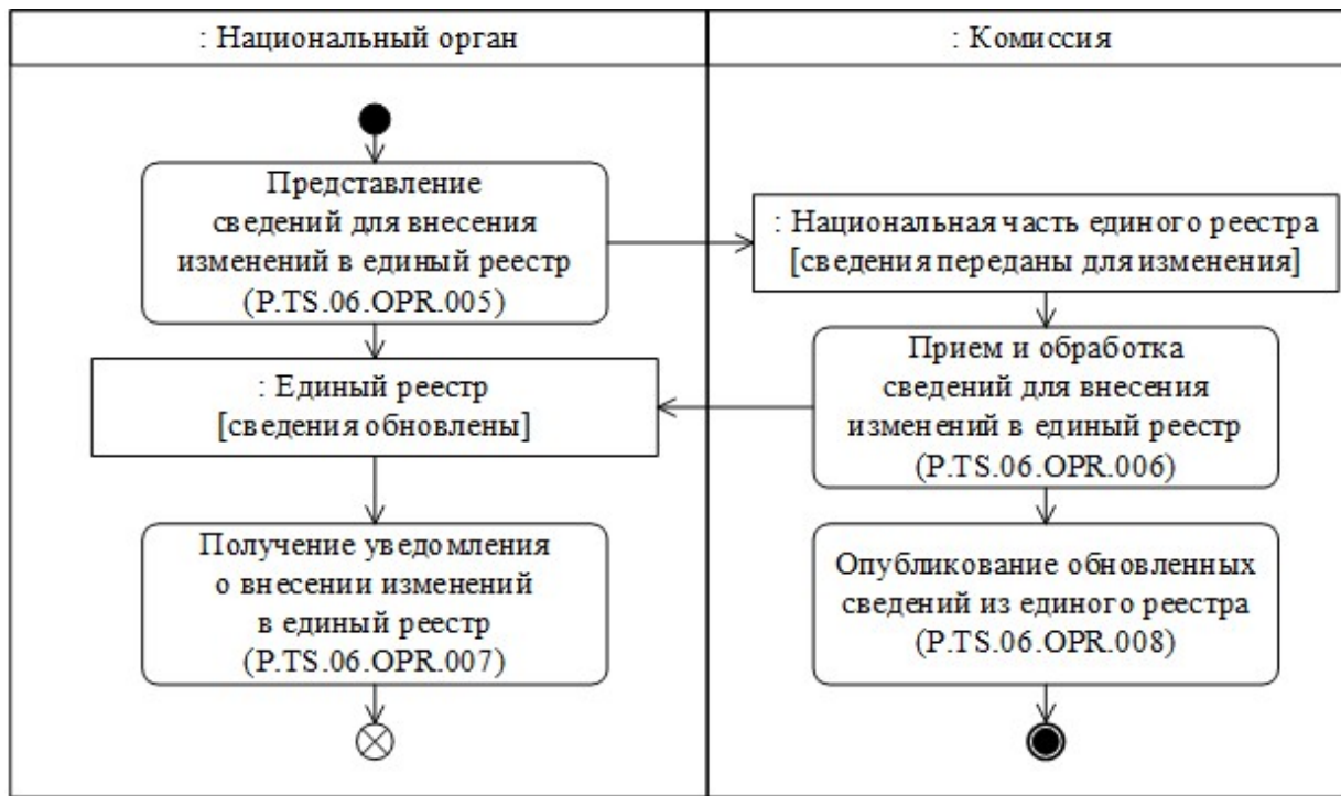
Рис. 6. Схема выполнения процедуры "Изменение сведений, содержащихся в едином реестре" (P.TS.06.PRC.002)
