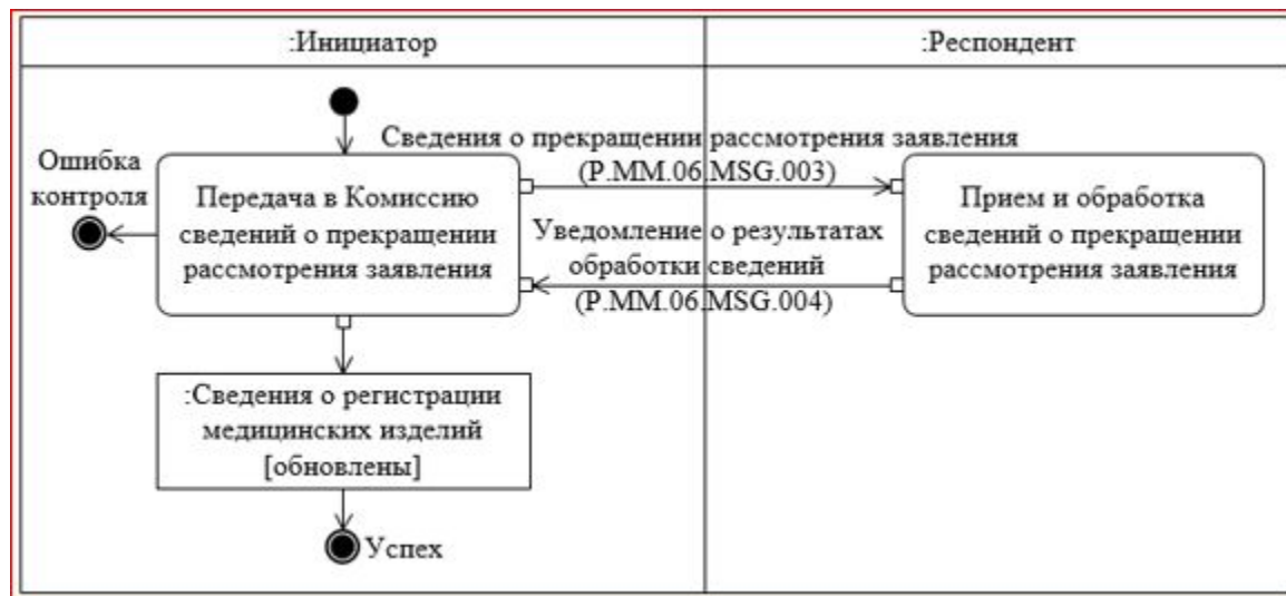
Рис. 6. Схема выполнения транзакции общего процесса "Передача в Комиссию сведений о прекращении рассмотрения заявления" (P.MM.06.TRN.003)
