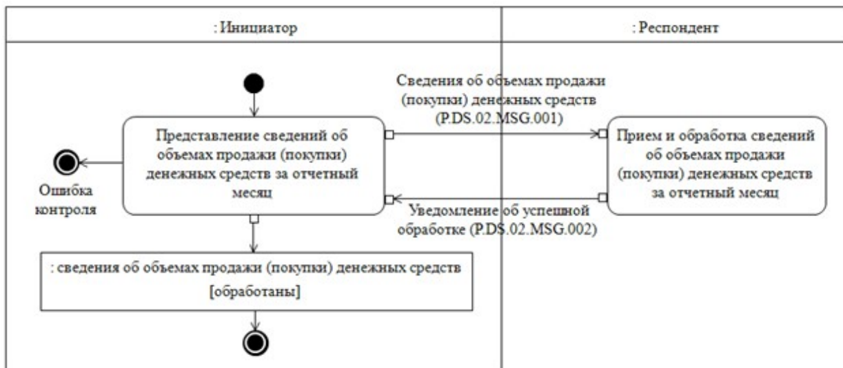
Рис. 3. Схема выполнения транзакции общего процесса «Представление сведений об объемах продажи (покупки) денежных средств за отчетный месяц» (P.DS.02.TRN.001)
