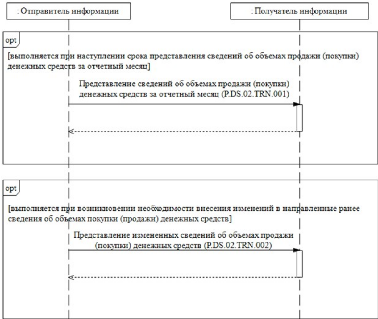
Рис. 2. Схема выполнения транзакций общего процесса при представлении сведений уполномоченными органами государств-членов в Комиссию
