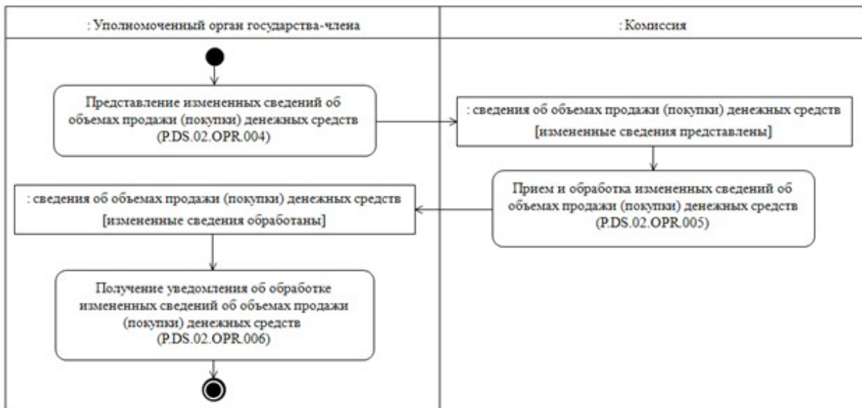
Рис. 3. Схема выполнения процедуры "Представление измененных сведений об объемах продажи (покупки) денежных средств" (P.DS.02.PRC.002)
