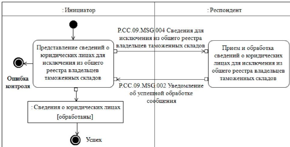
Рис. 6. Схема выполнения транзакции общего процесса "Исключение сведений о юридических лицах из общего реестра владельцев таможенных складов" (P.CC.09.TRN.003)
