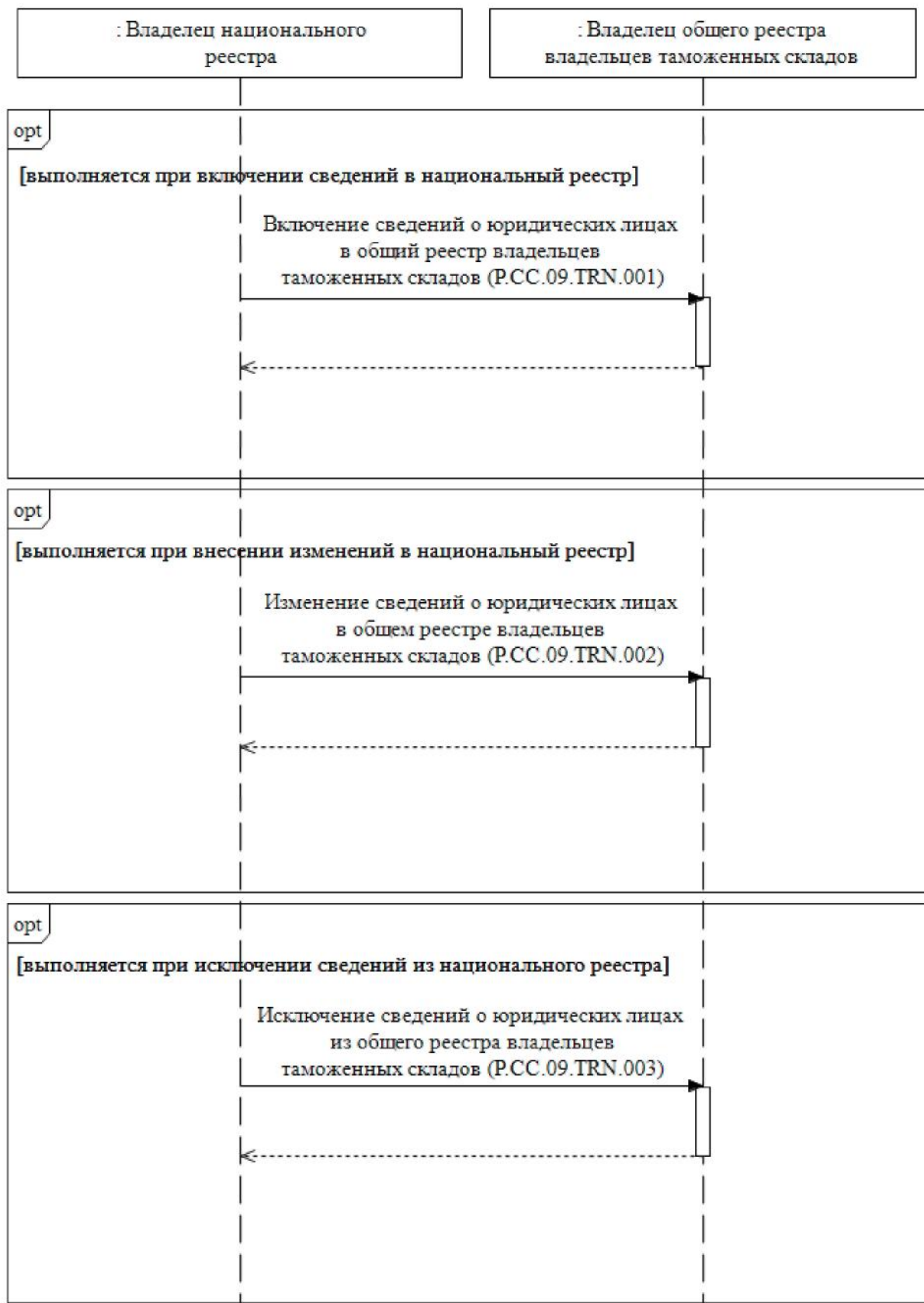
Рис. 2. Схема выполнения транзакций общего процесса при формировании и ведении общего реестра владельцев таможенных складов
