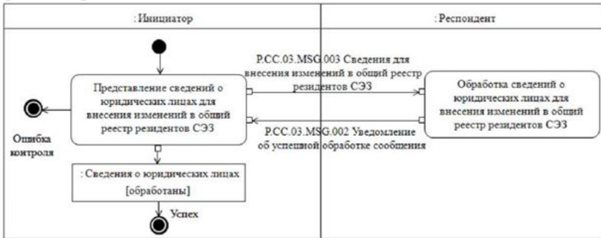
Рис. 5. Схема выполнения транзакции общего процесса «Изменение сведений о юридических лицах общего реестра резидентов СЭЗ» (P.CC.03.TRN.002)
