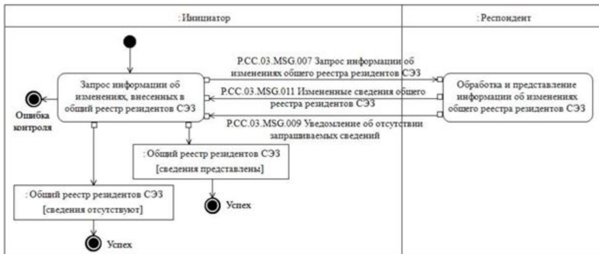
Рис. 5. Схема выполнения транзакции общего процесса «Получение информации об изменениях, внесенных в общий реестр резидентов СЭЗ» (P.CC.03.TRN.006)
