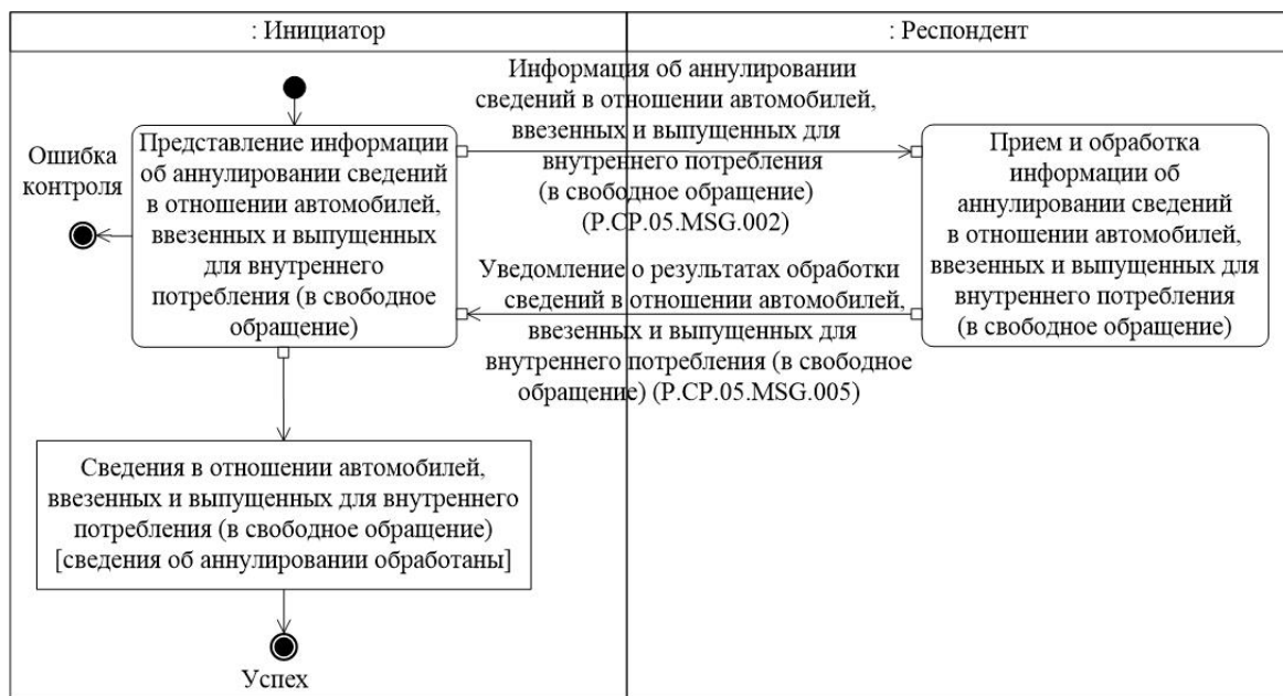
Рис. 5. Схема выполнения транзакции общего процесса "Аннулирование сведений в отношении автомобилей, ввезенных и выпущенных для внутреннего потребления (в свободное обращение)" (P.SP.05.TRN.002)
