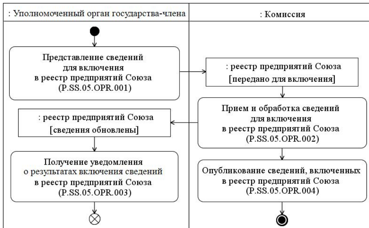
Рис. 4. Схема выполнения процедуры "Включение сведений в реестр предприятий Союза" (P.SS.05.PRC.001)
