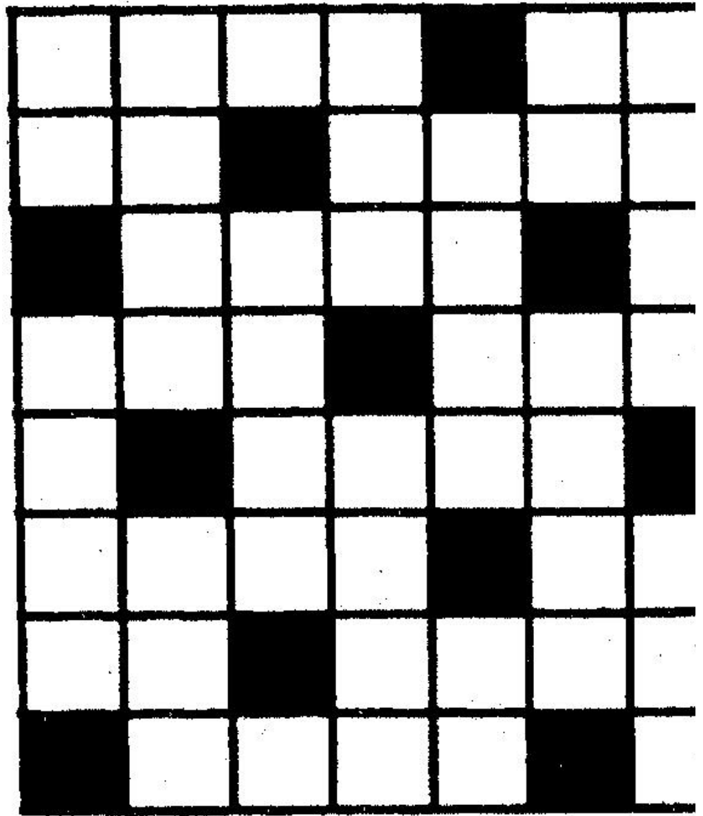
Атласное переплетение
