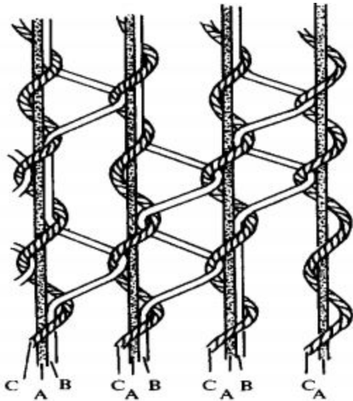
Рис. 3 БОБИННЫЙ ПЮЛЬ А – основная нить; В – нить, образующая рисунок; С – перевивочная нить.
