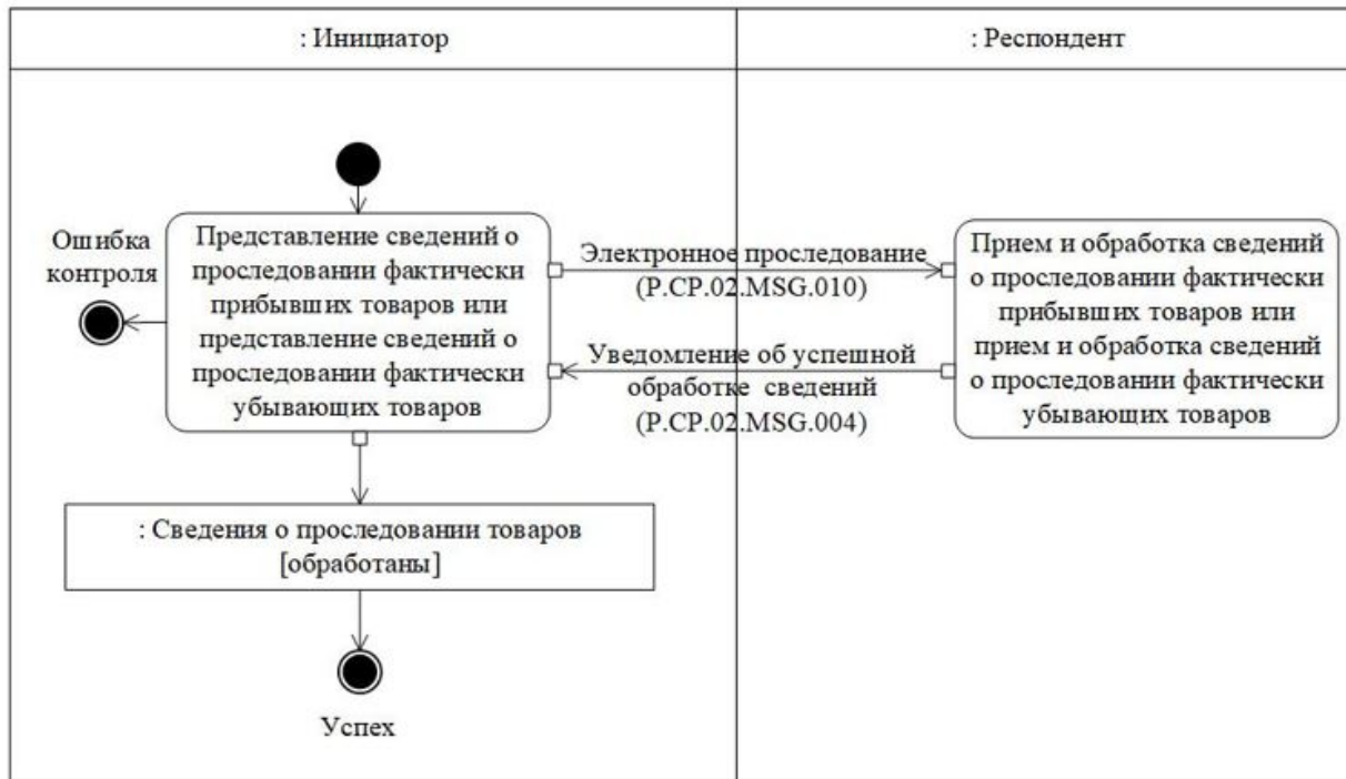
Рис. 13. Схема выполнения транзакции общего процесса "Оповещение о проследовании товаров" (P.SP.02.TRN.006)
