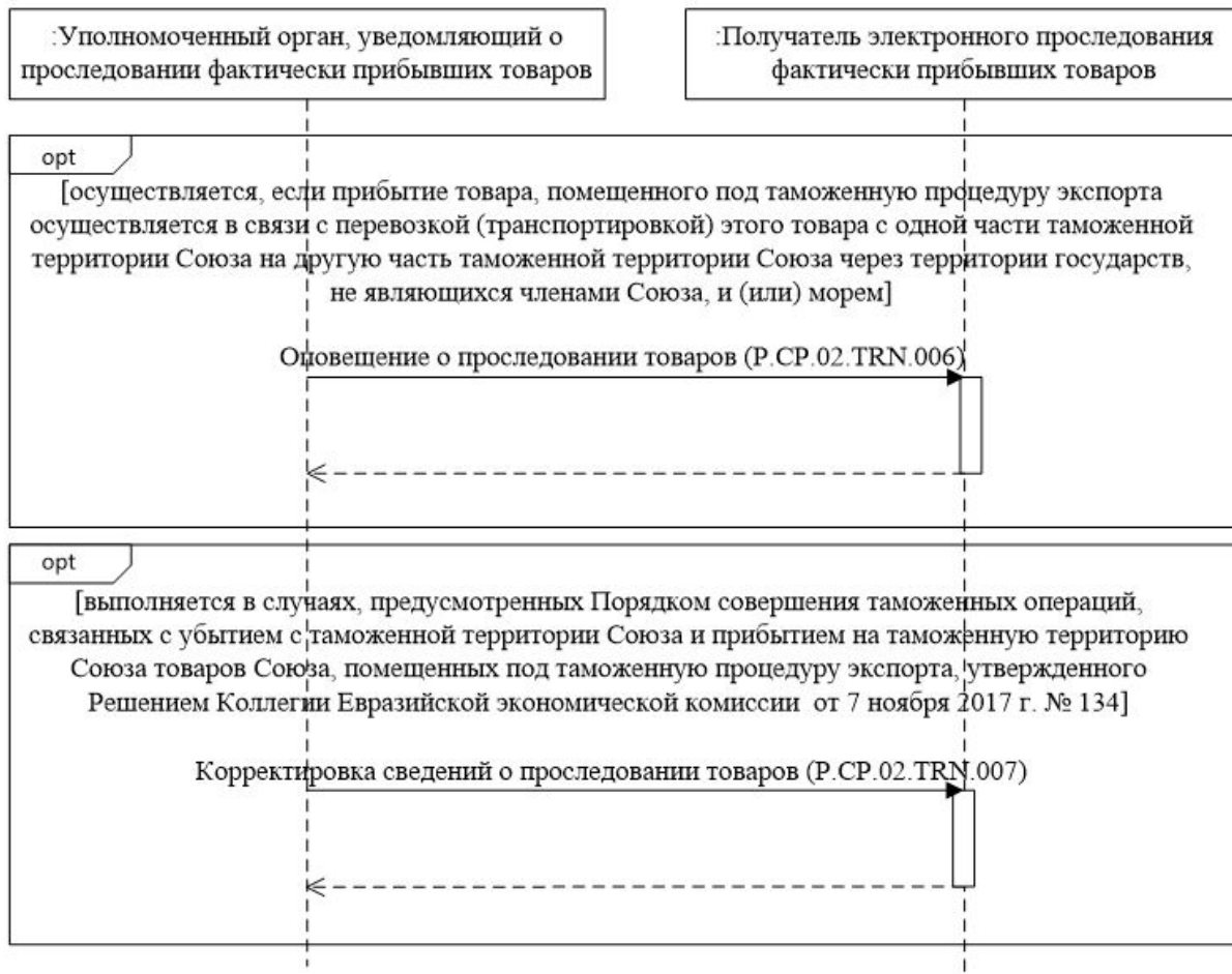
Рис. 5. Схема выполнения транзакций общего процесса при оповещении о проследовании товаров через территории государств, не являющихся членами Союза
