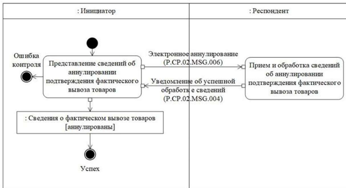
Рис. 10. Схема выполнения транзакции общего процесса "Аннулирование сведений о фактическом вывозе товаров" (P.SP.02.TRN.003)
