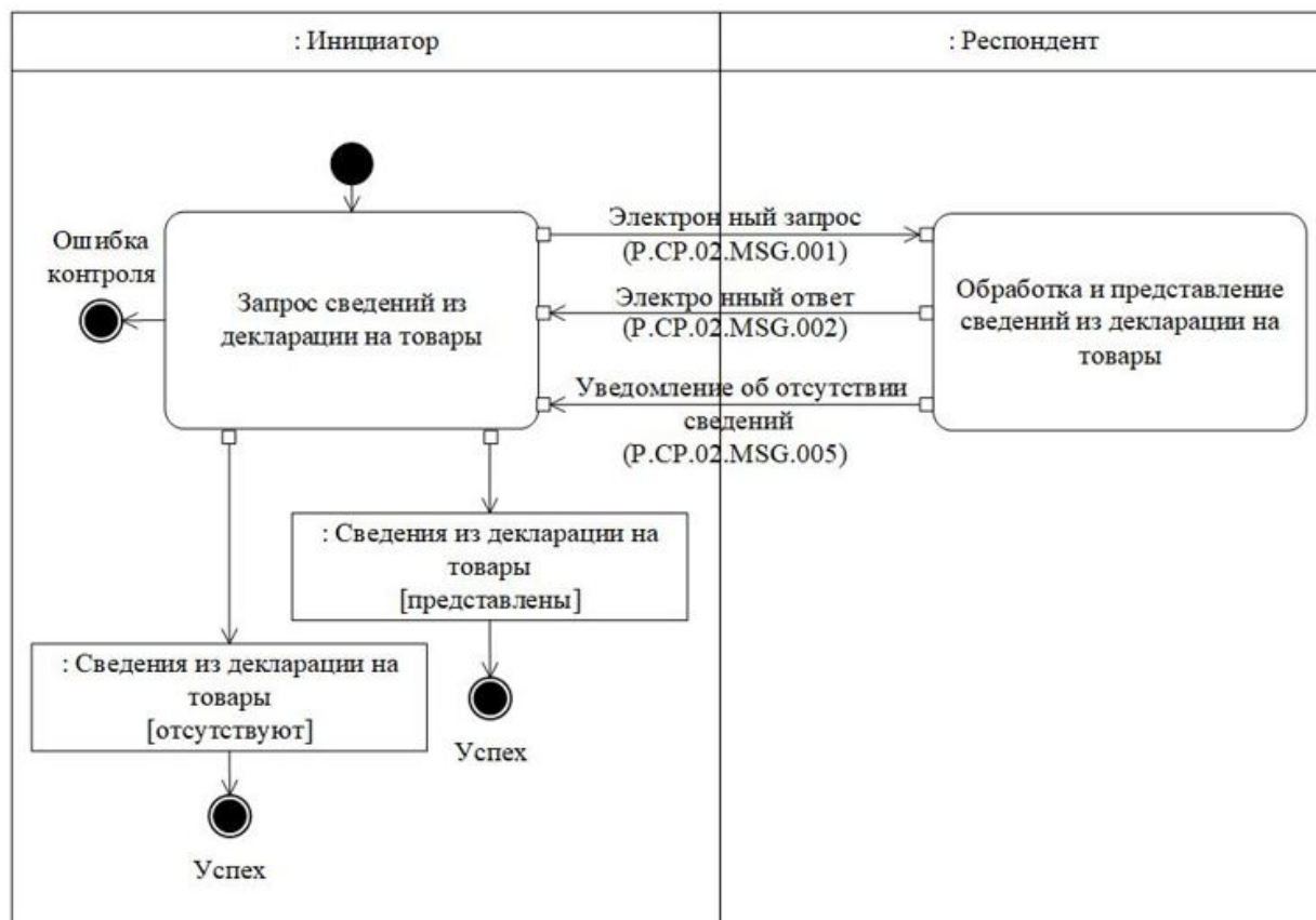
Рис. 8. Схема выполнения транзакции общего процесса "Получение сведений из декларации на товары" (P.CP.02.TRN.001)
