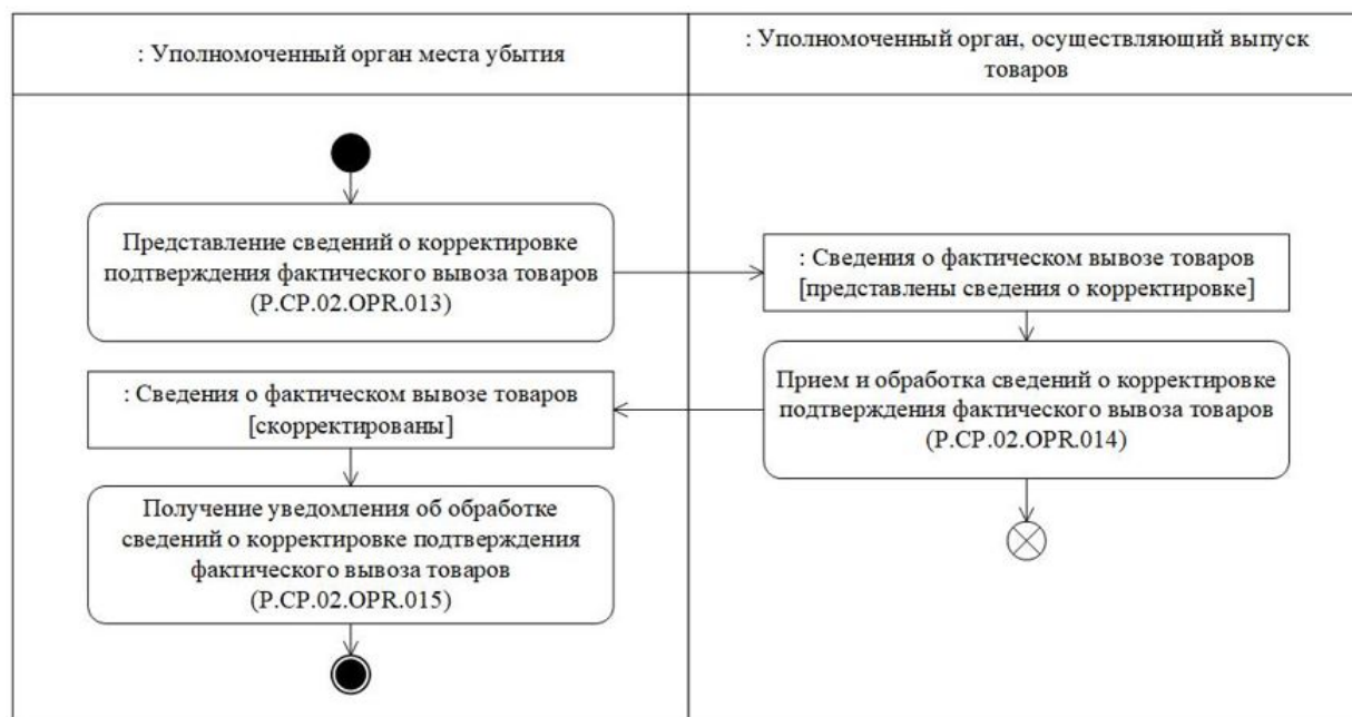
Рис. 8. Схема выполнения процедуры "Корректировка сведений о фактическом вывозе товаров" (P.SP.02.PRC.005)
