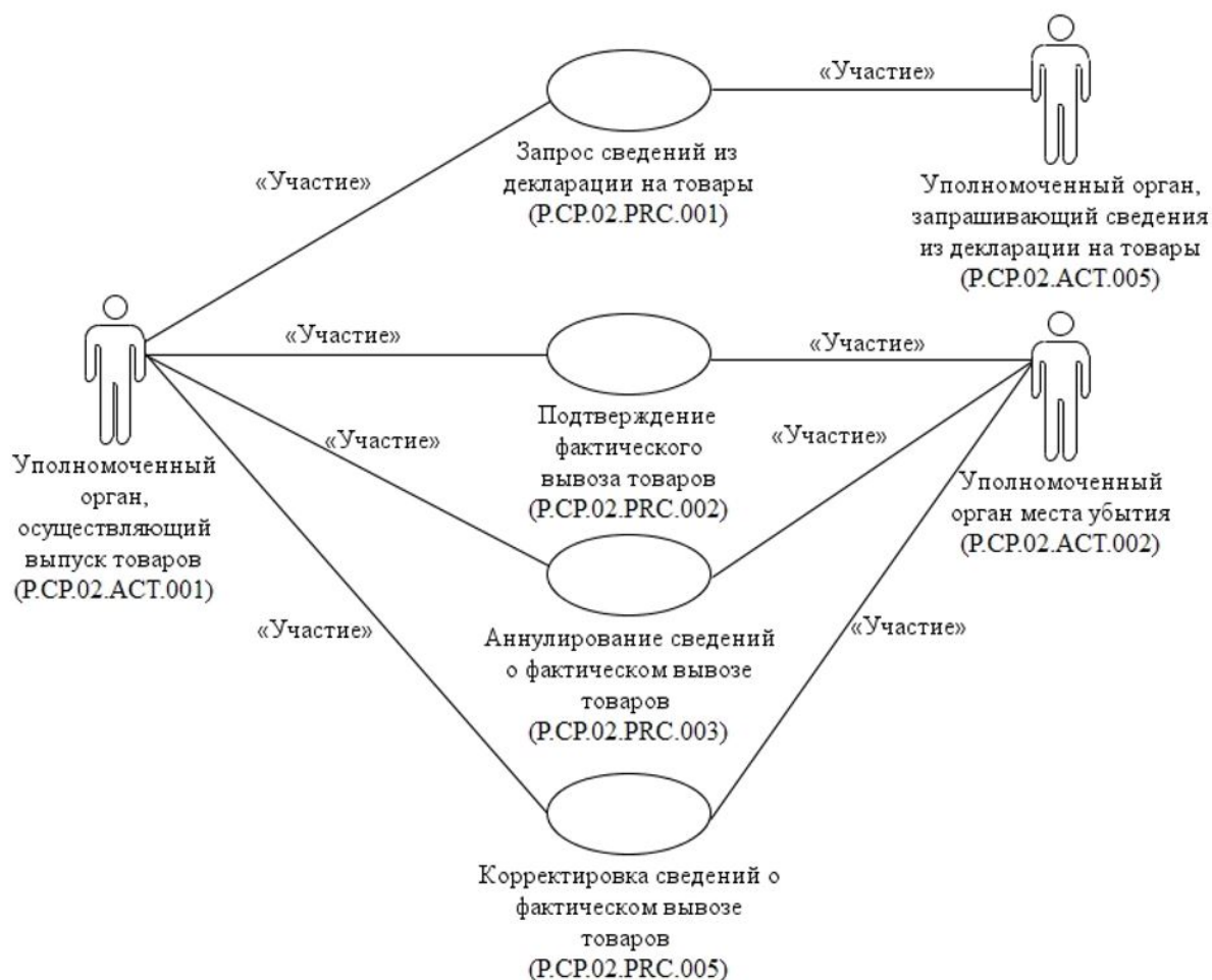
Рис. 2. Общая схема группы процедур информационного обеспечения контроля за фактическим вывозом товаров в процессе их убытия с таможенной территории Союза
