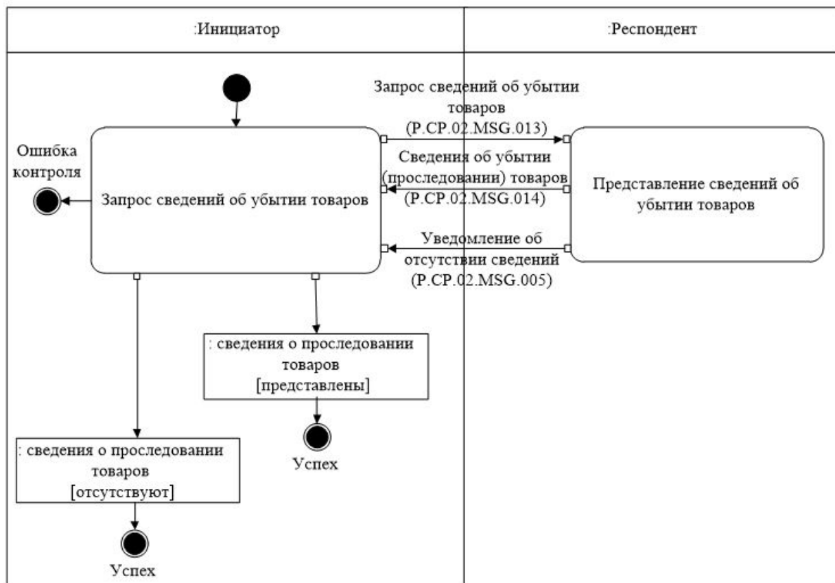
Рис. 16. Схема выполнения транзакции общего процесса "Запрос сведений об убытии товаров" (P.SP.02.TRN.009)
