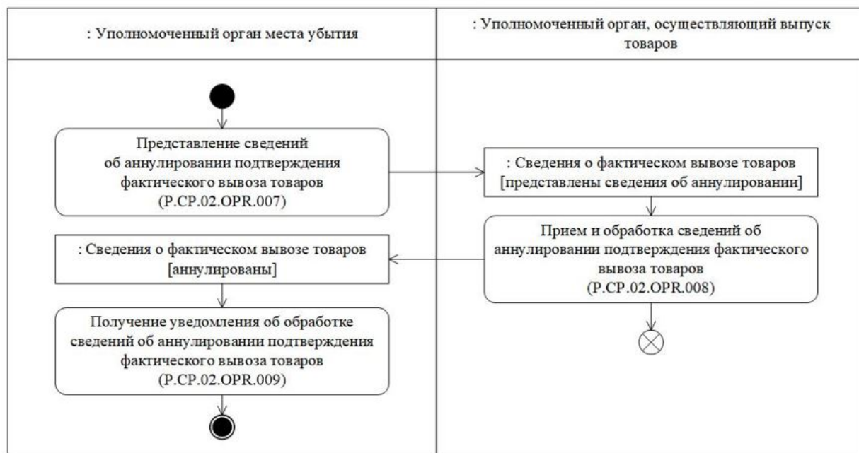
Рис. 7. Схема выполнения процедуры "Аннулирование сведений о фактическом вывозе товаров" (P.CP.02.PRC.003)
