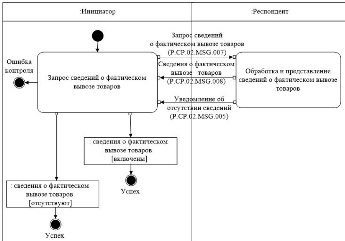
Рис. 11. Схема выполнения транзакции общего процесса "Запрос сведений о фактическом вывозе товаров" (P.SP.02.TRN.004)
