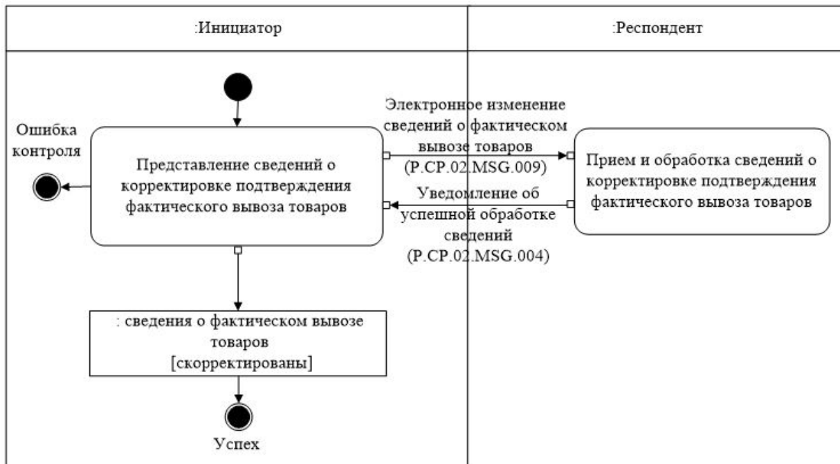
Рис. 12. Схема выполнения транзакции общего процесса "Корректировка сведений о фактическом вывозе товаров" (P.SP.02.TRN.005)
