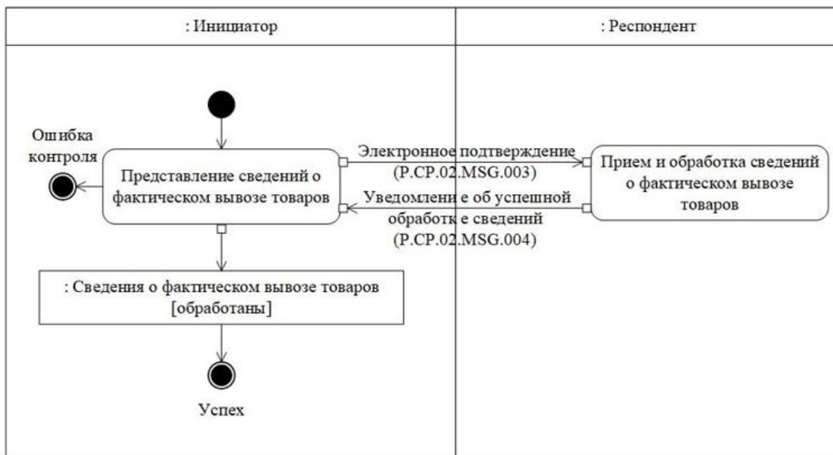
Рис. 9. Схема выполнения транзакции общего процесса "Подтверждение фактического вывоза товаров" (P.SP.02.TRN.002)
