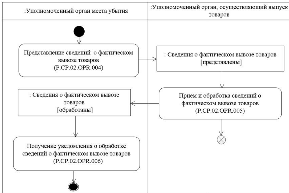
Рис. 6. Схема выполнения процедуры "Подтверждение фактического вывоза товаров" (P.SP.02.PRC.002)
