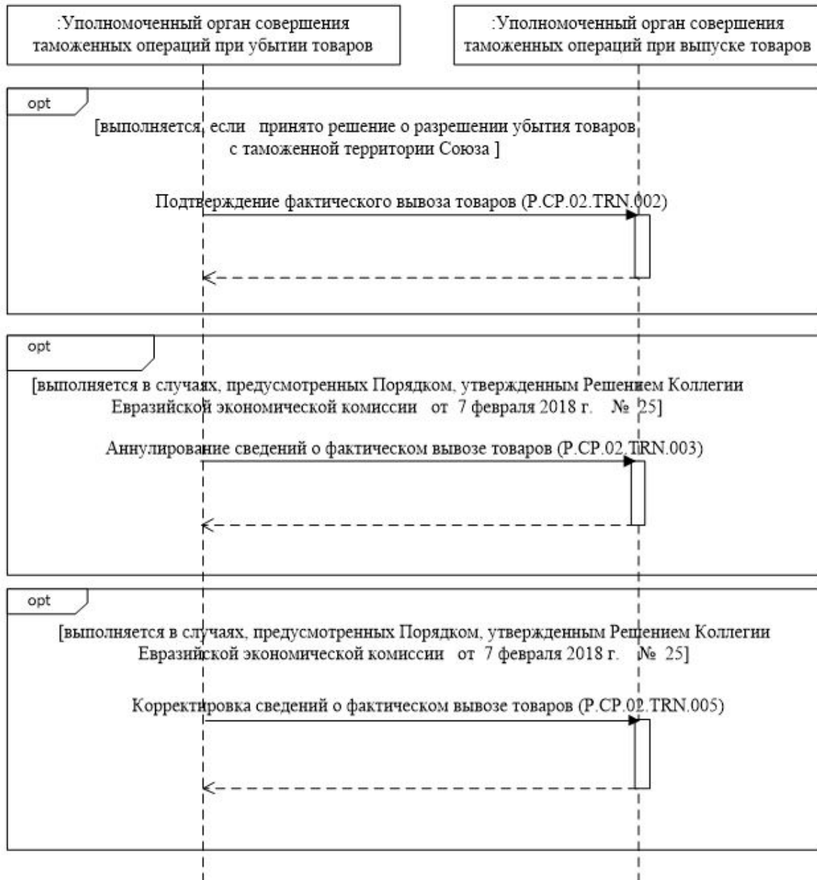
Рис. 3. Схема выполнения транзакций общего процесса при обеспечении контроля за фактическим вывозом товаров в процессе их убытия с таможенной территории Союза
