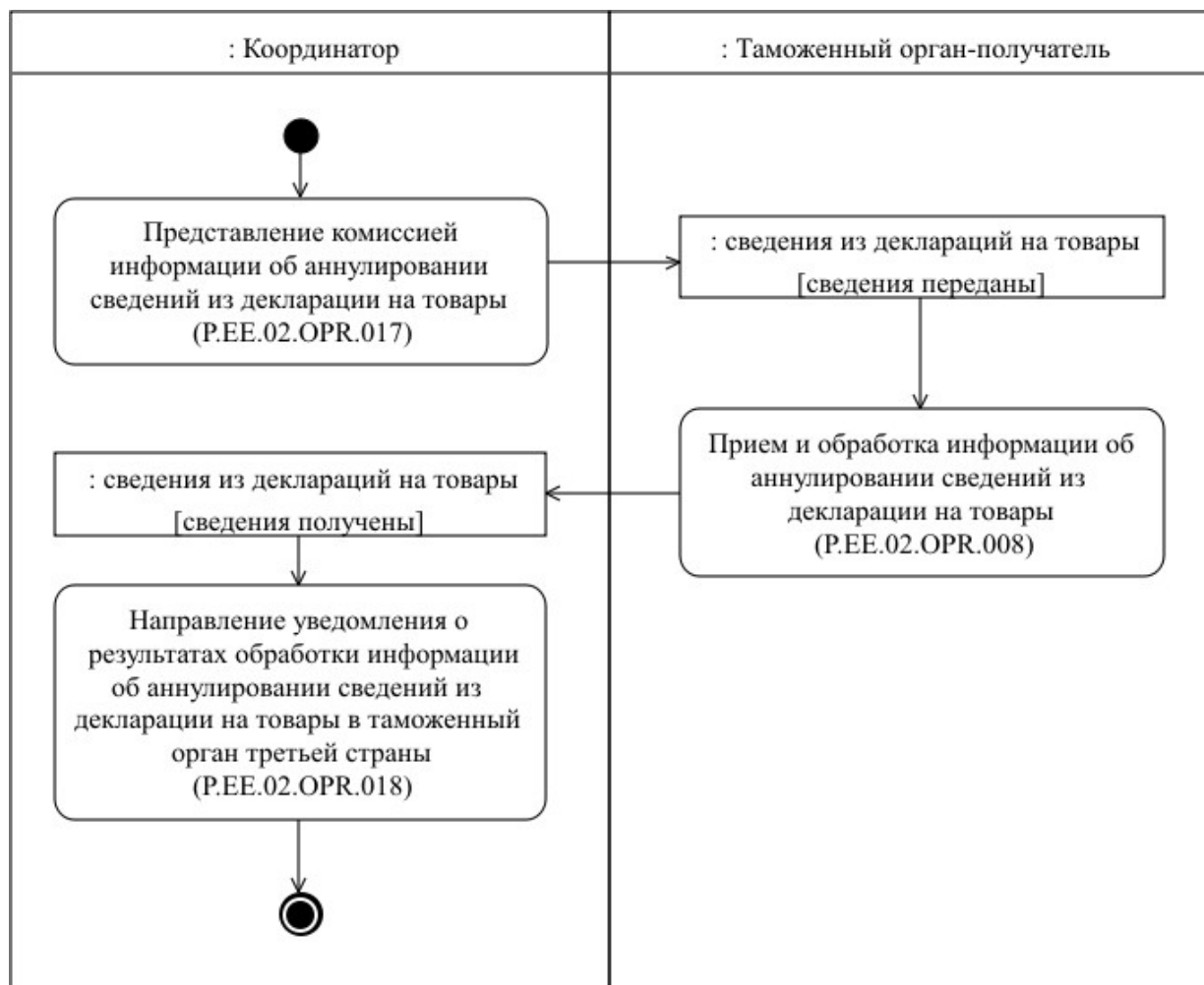
Рис. 9. Схема выполнения процедуры "Получение информации об аннулировании сведений из декларации на товары" (P.EE.02.PRC.006)
