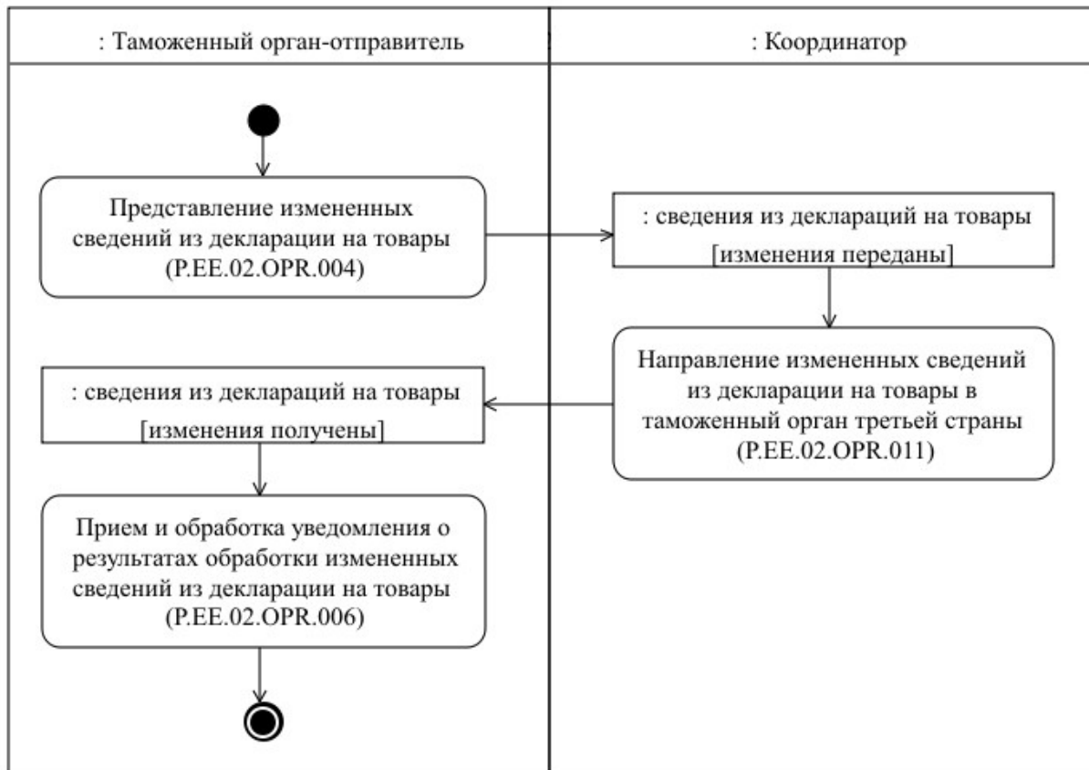
Рис. 5. Схема выполнения процедуры "Внесение изменений в сведения, представленные ранее из базы данных электронных копий деклараций на товары" (P.EE.02.PRC.002)
