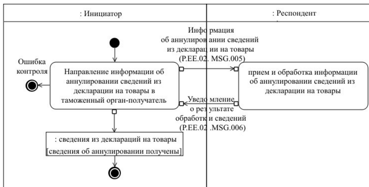
Рис. 9. Схема выполнения транзакции общего процесса "Получение информации об аннулировании сведений из декларации на товары от таможенного органа третьей страны" (P.EE.02.TRN.006)
