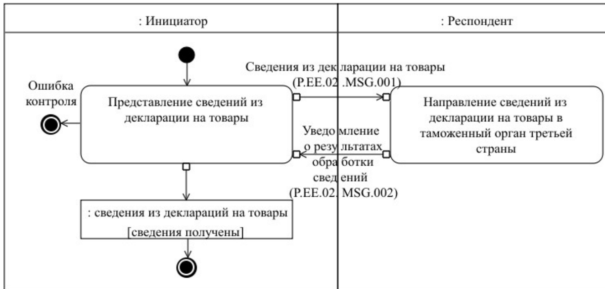
Рис. 4. Схема выполнения транзакции общего процесса "Представление сведений из декларации на товары в таможенный орган третьей страны" (P.EE.02.TRN.001)
