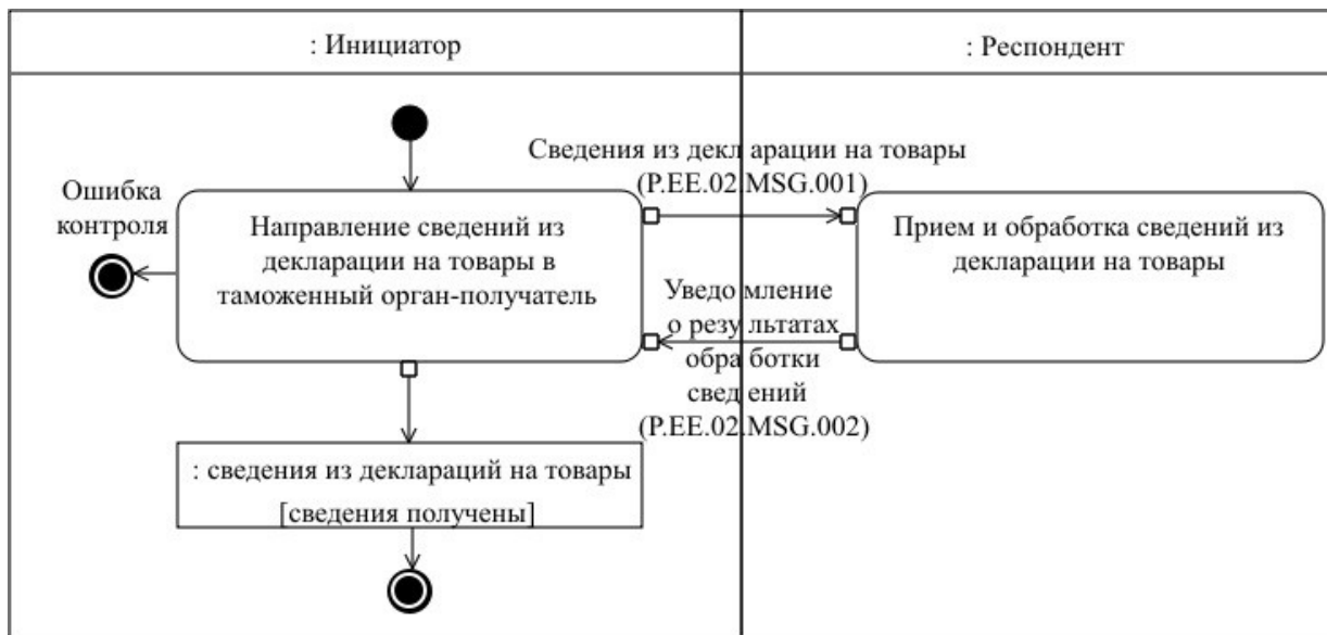
Рис. 7. Схема выполнения транзакции общего процесса "Получение сведений из деклараций на товары от таможенного органа третьей страны" (P.EE.02.TRN.004)
