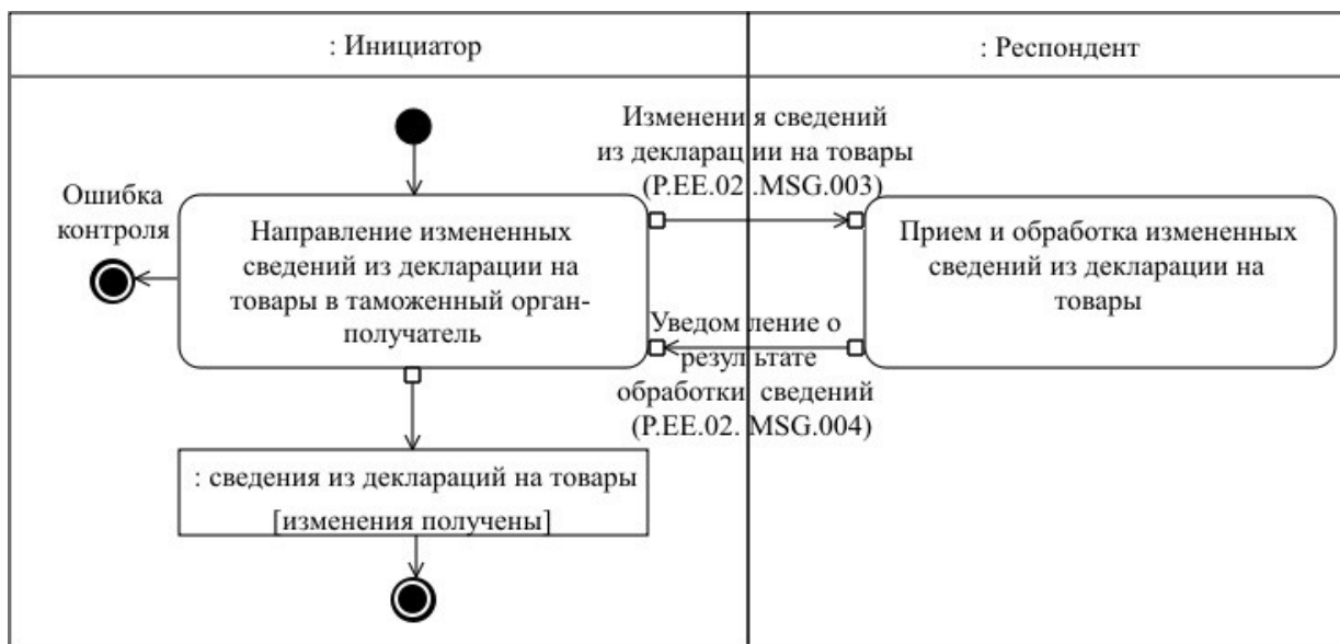
Рис. 8. Схема выполнения транзакции общего процесса "Получение измененных сведений из деклараций на товары от таможенного органа третьей страны" (P.EE.02.TRN.005)
