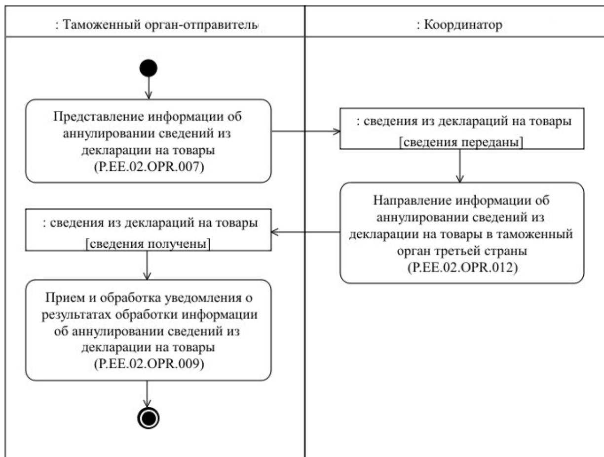
Рис. 6. Схема выполнения процедуры "Аннулирование сведений, представленных ранее из базы данных электронных копий деклараций на товары" (P.EE.02.PRC.003)
