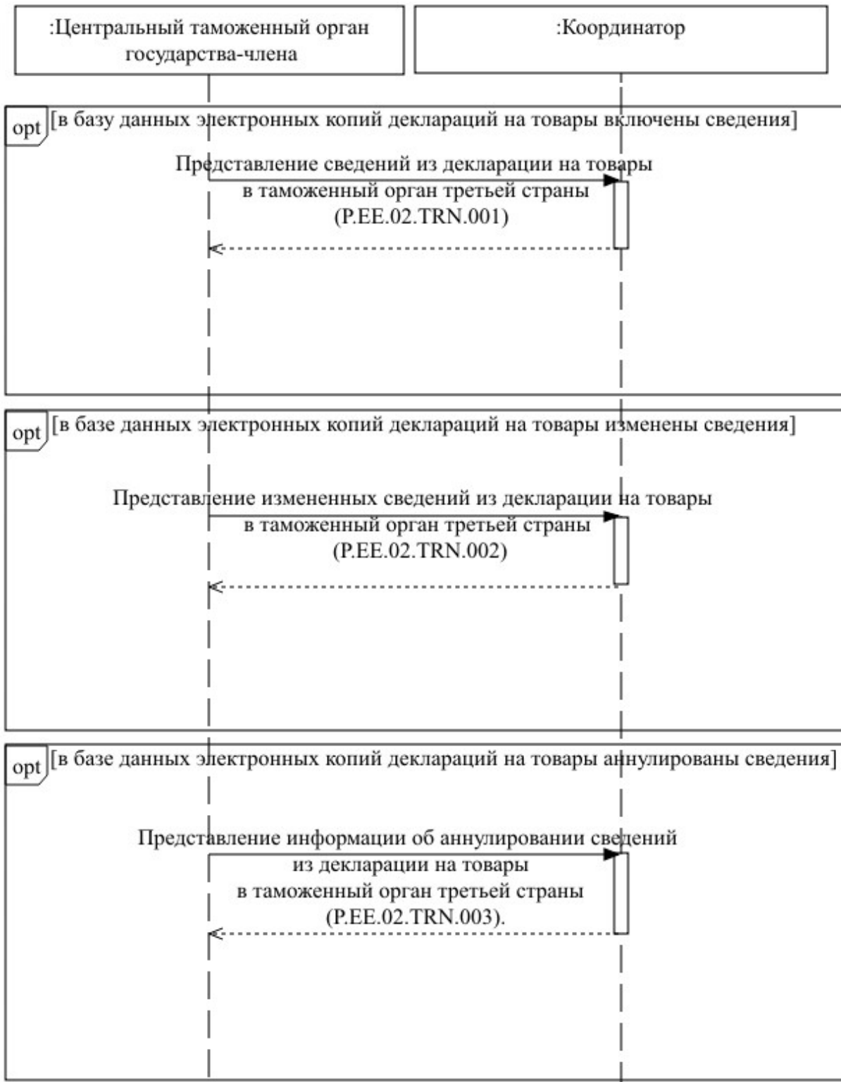
Рис. 2. Схема выполнения транзакций общего процесса при представлении сведений из деклараций на товары
