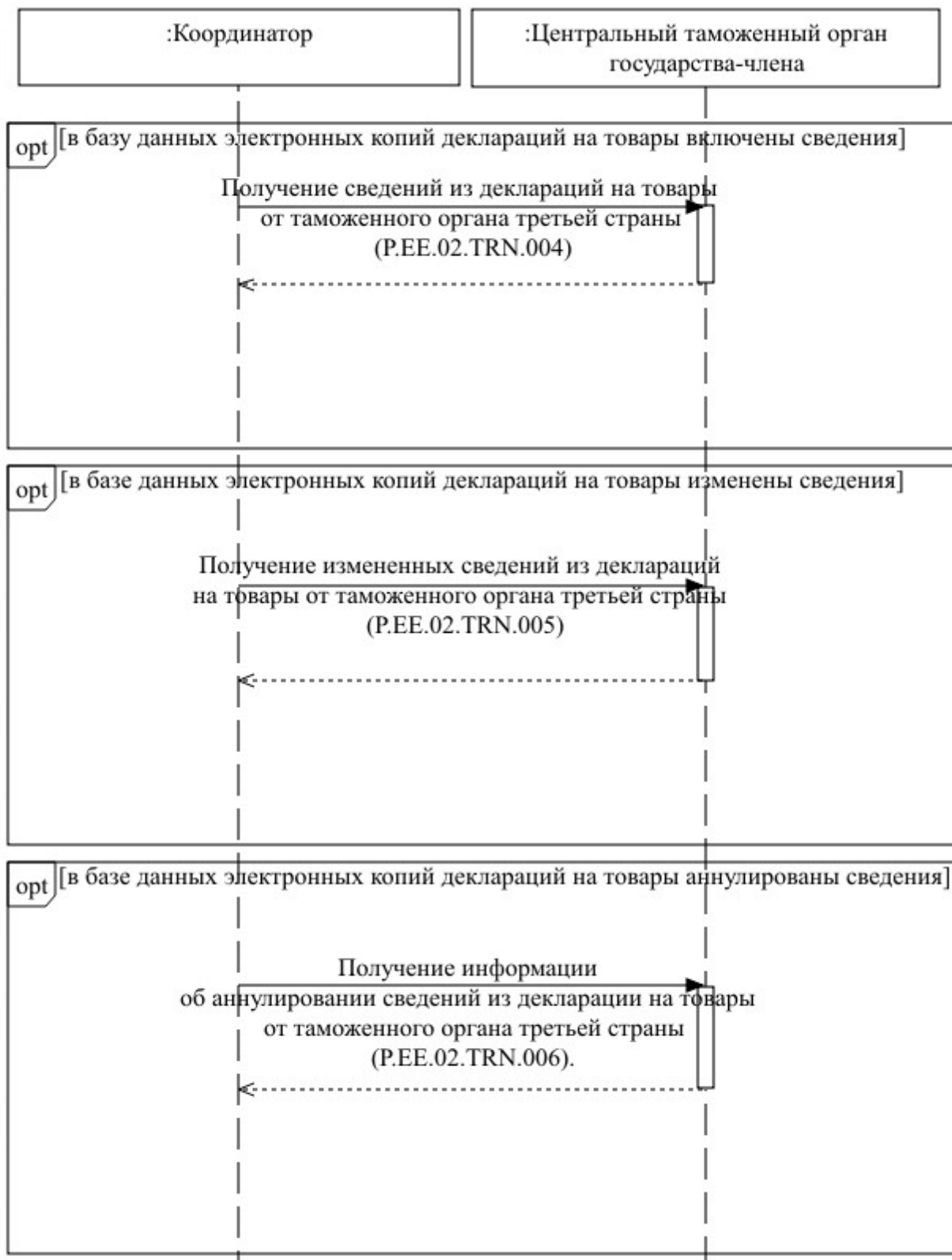
Рис. 3. Схема выполнения транзакций общего процесса при получении сведений из деклараций на товары
