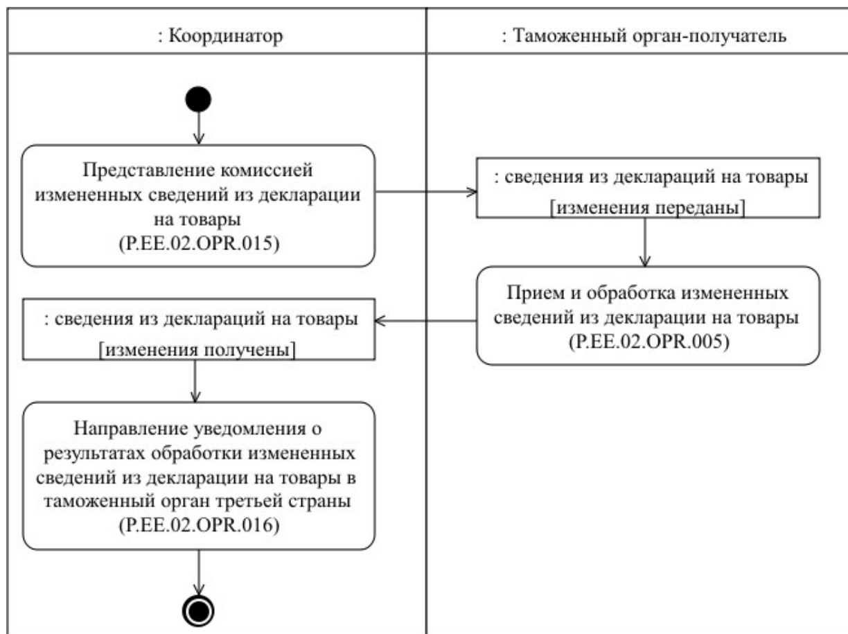
Рис. 8. Схема выполнения процедуры "Получение изменений в сведения, представленные ранее из базы данных электронных копий деклараций на товары" (P.EE.02.PRC.005)
