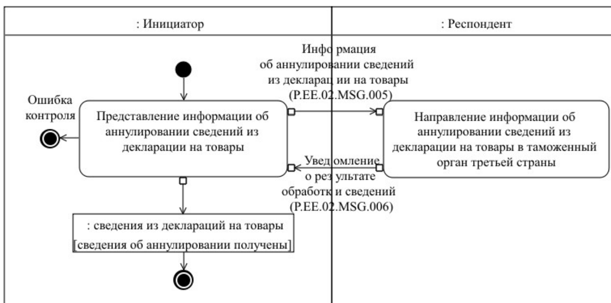
Рис. 6. Схема выполнения транзакции общего процесса "Представление информации об аннулировании сведений из декларации на товары в таможенный орган третьей страны" (P.EE.02.TRN.003)
