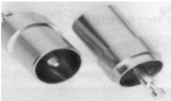
Рис. 1. Коаксиальная штепсельная вилка
