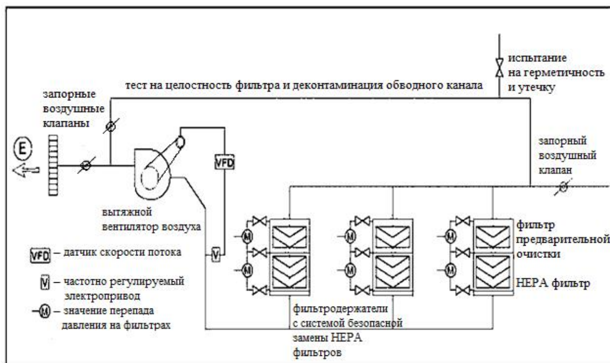
Рис. 2. Схема системы фильтрации с обводным каналом и системой безопасной замены фильтров
