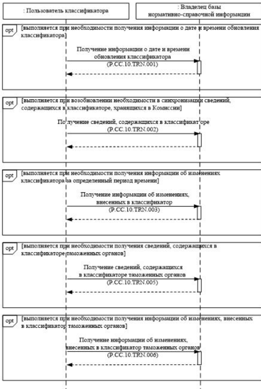
Рис. 2. Схема выполнения транзакций общего процесса при представлении уполномоченным органам государств-членов сведений, содержащихся в классификаторе, используемом для заполнения таможенных документов, или сведений, содержащихся в классификаторе таможенных органов
