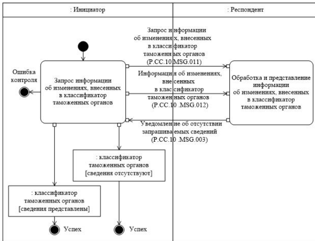
Рис. 10. Схема выполнения транзакции общего процесса "Получение информации об изменениях, внесенных в классификатор таможенных органов" (P.CC.10.TRN.006)
