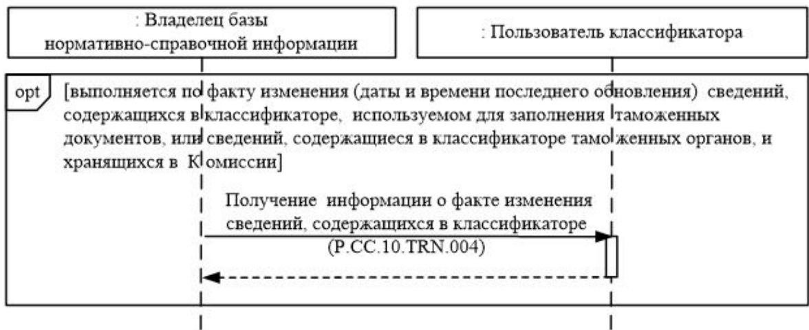
Рис. 3. Схема выполнения транзакций общего процесса при информировании уполномоченных органов государств-членов о факте изменения сведений, содержащихся в классификаторе, используемом для заполнения таможенных документов, или сведений, содержащихся в классификаторе таможенных органов
