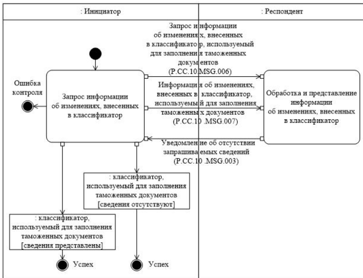
Рис. 7. Схема выполнения транзакции общего процесса "Получение информации об изменениях, внесенных в классификатор" (P.CC.10.TRN.003)
