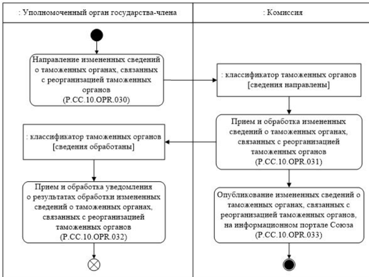
Рис. 15. Схема выполнения процедуры "Представление измененных сведений о таможенных органах, связанных с реорганизацией таможенных органов" (P.CC.10.PRC.011)
