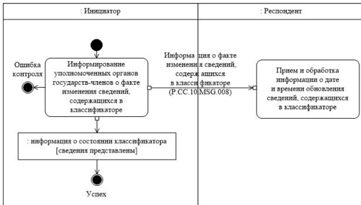
Рис. 8. Схема выполнения транзакции общего процесса "Получение информации о факте изменения сведений, содержащихся в классификаторе" (P.CC.10.TRN.004)
