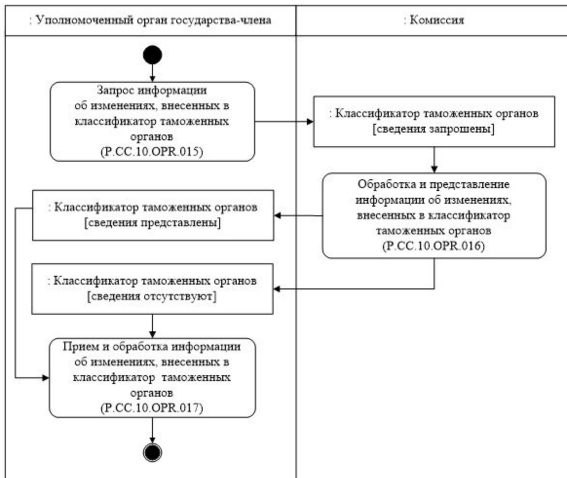
Рис. 10. Схема выполнения процедуры "Получение информации об изменениях, внесенных в классификатор таможенных органов" (P.СC.10.PRC.007)
