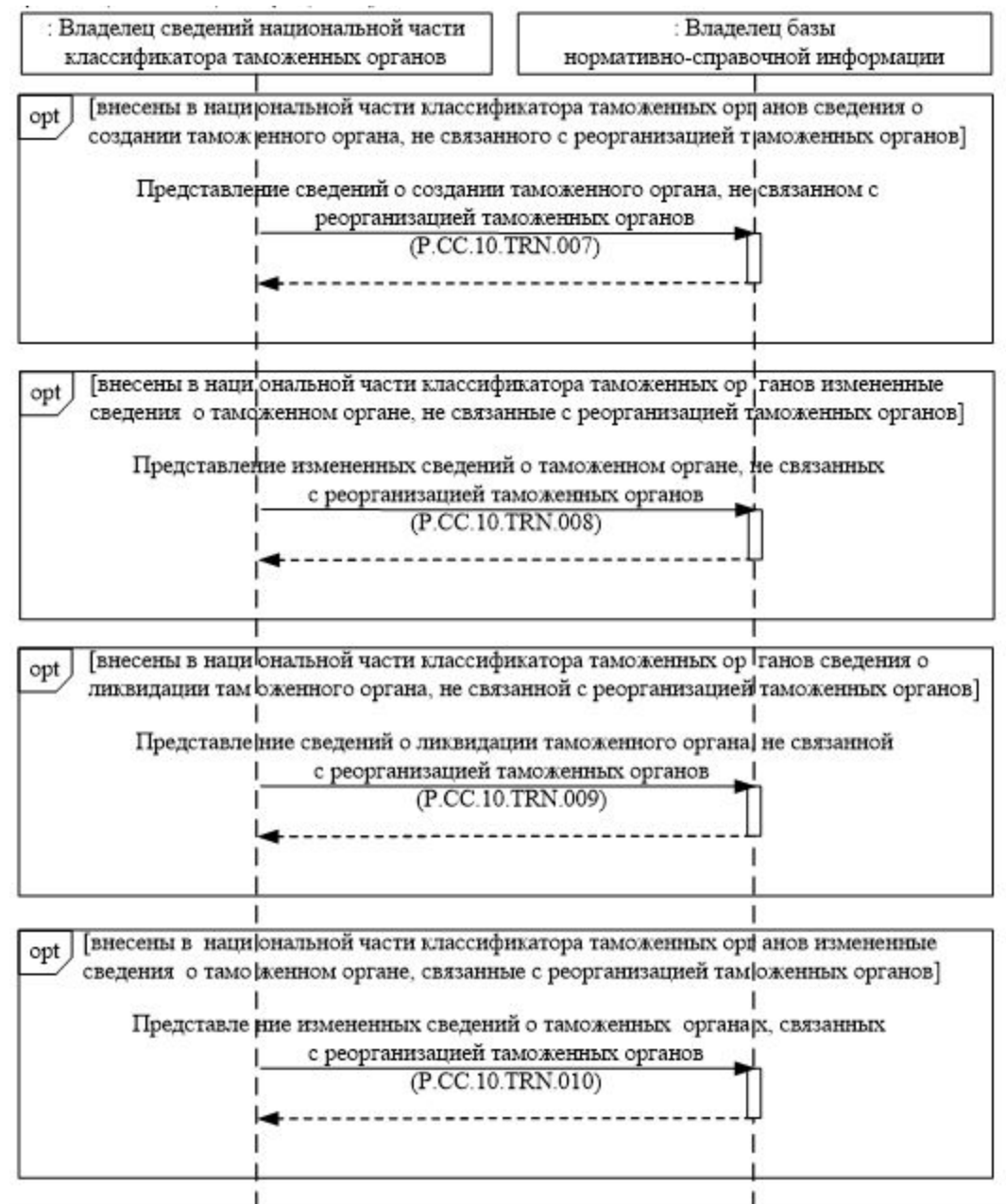
Рис. 4. Схема выполнения транзакций общего процесса при формировании классификатора таможенных органов
