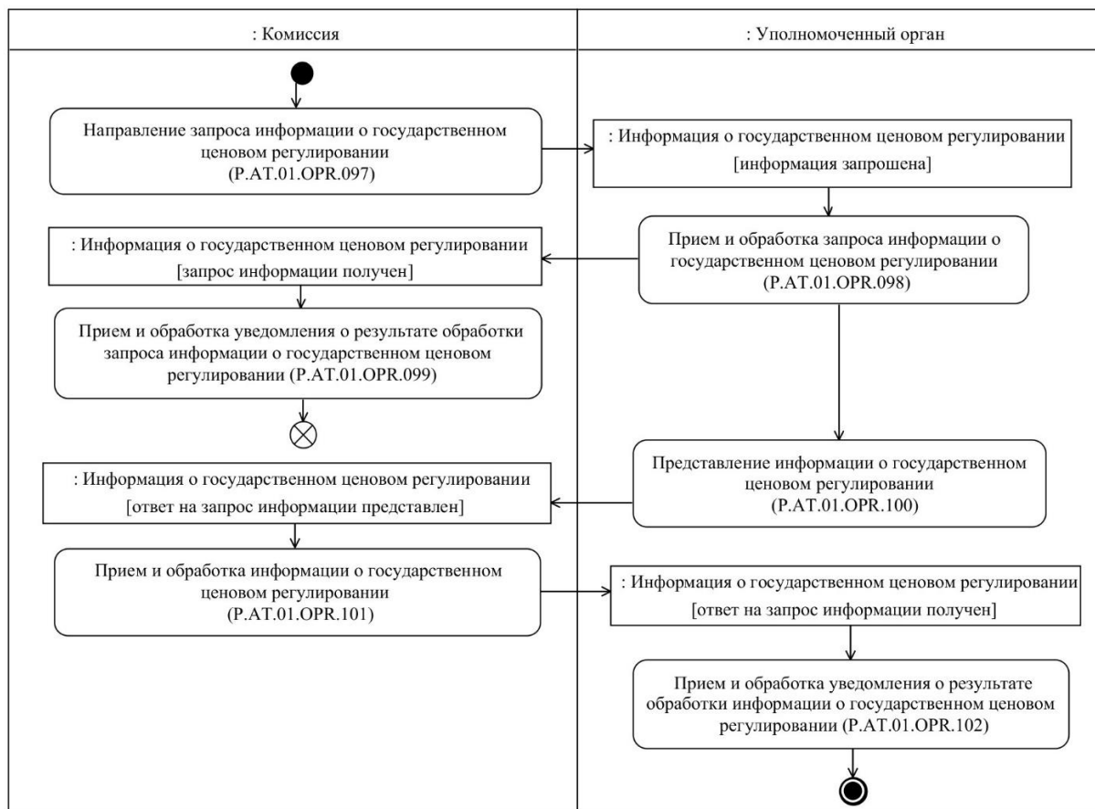
Рис. 7. Схема выполнения процедуры "Получение информации при рассмотрении обращения" (P.AT.01.PRC.028)
