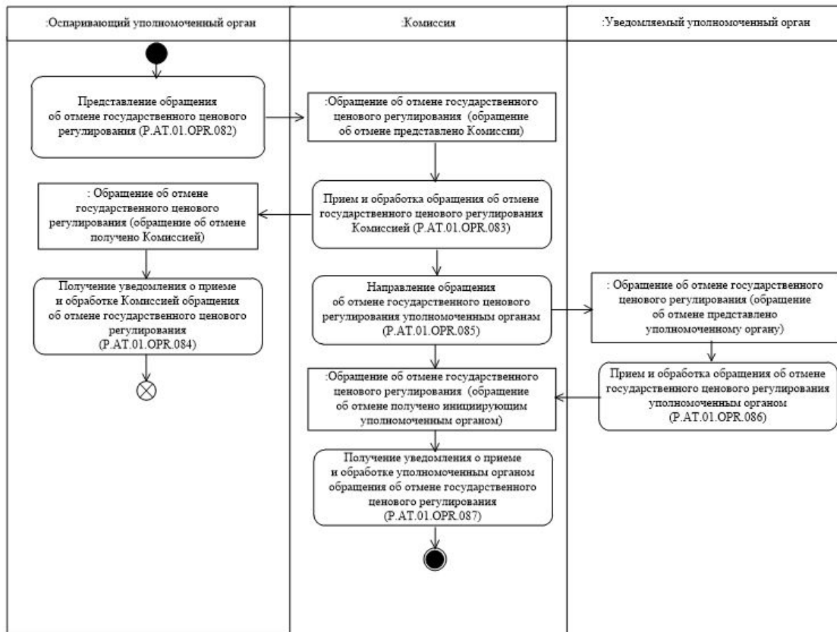
Рис. 4. Схема выполнения процедуры "Обращение об отмене государственного ценового регулирования" (P.AT.01.PRC.025)
