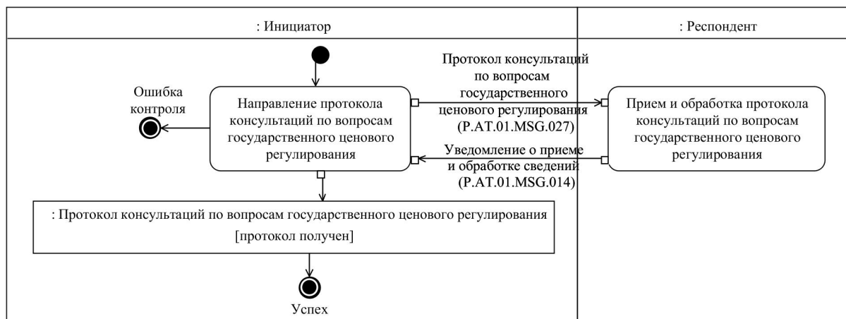
Рис. 9. Схема выполнения транзакции общего процесса "Направление протокола консультаций по вопросам государственного ценового регулирования" (P.AT.01.TRN.027)
