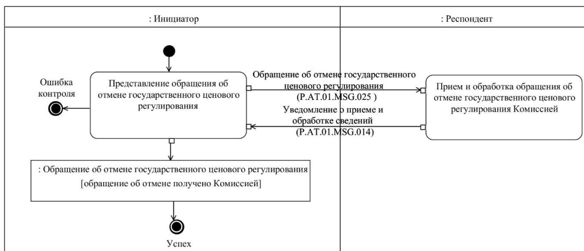
Рис. 5. Схема выполнения транзакции общего процесса "Направление обращения об отмене государственного ценового регулирования в Комиссию" (P.AT.01.TRN.023)
