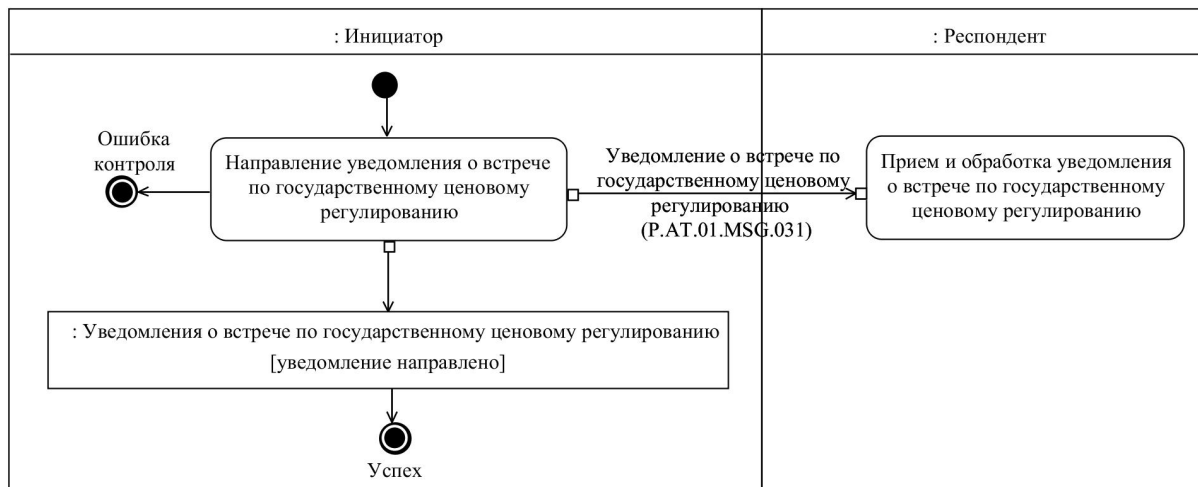
Рис. 13. Схема выполнения транзакции общего процесса "Направление уведомления о встрече по государственному ценовому регулированию" (P.AT.01.TRN.031)
