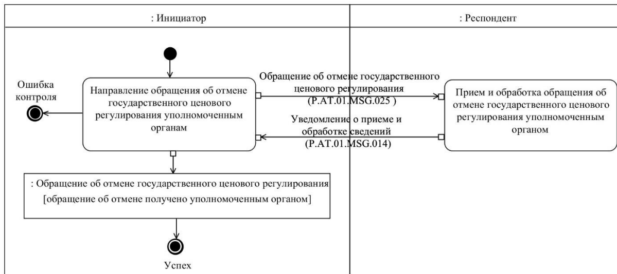
Рис. 6. Схема выполнения транзакции общего процесса "Направление обращения об отмене государственного ценового регулирования в уполномоченные органы" (P.AT.01.TRN.024)
