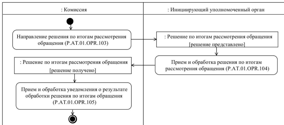
Рис. 8. Схема выполнения процедуры "Направление решения по итогам рассмотрения обращения" (P.AT.01.PRC.029)
