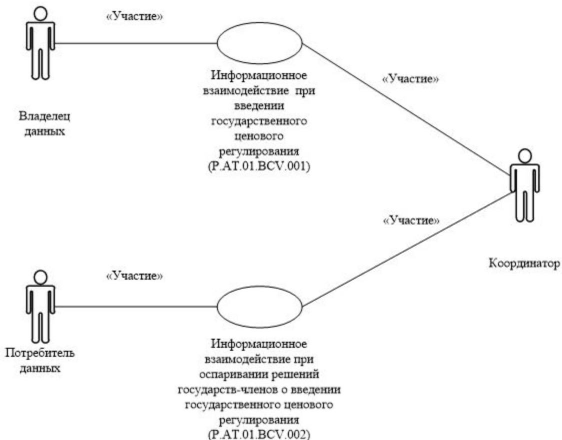
Рис. 1. Структура информационного взаимодействия между государствами-членами и Комиссией
