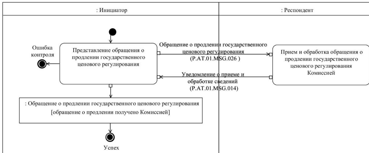
Рис. 7. Схема выполнения транзакции общего процесса "Направление обращения о продлении государственного ценового регулирования в Комиссию" (P.AT.01.TRN.025)
