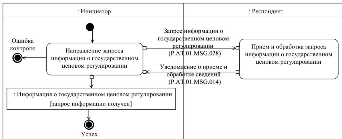
Рис. 10. Схема выполнения транзакции общего процесса "Запрос информации при рассмотрении обращения" (P.AT.01.TRN.028)
