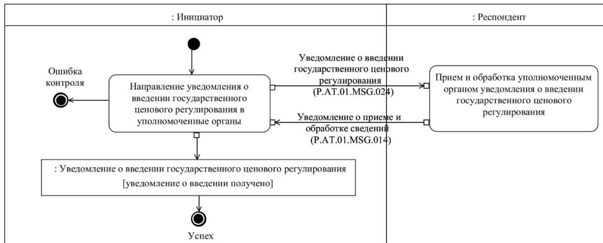
Рис. 3. Схема выполнения транзакции общего процесса "Уведомление о введении государственного ценового регулирования уполномоченных органов" (P.AT.01.TRN.022)
