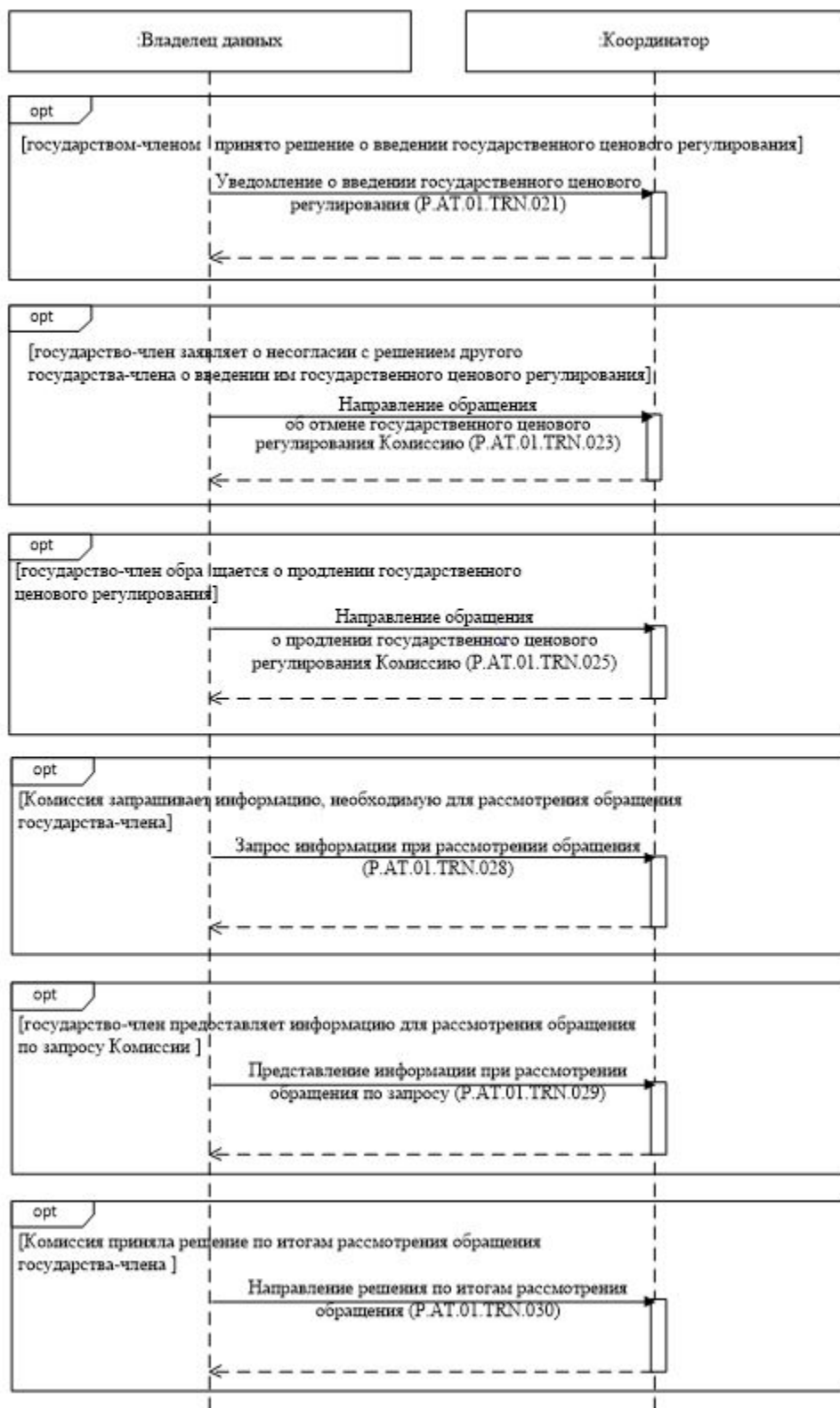
Рис. 2. Схема выполнения транзакций общего процесса при введении государственного ценового регулирования
