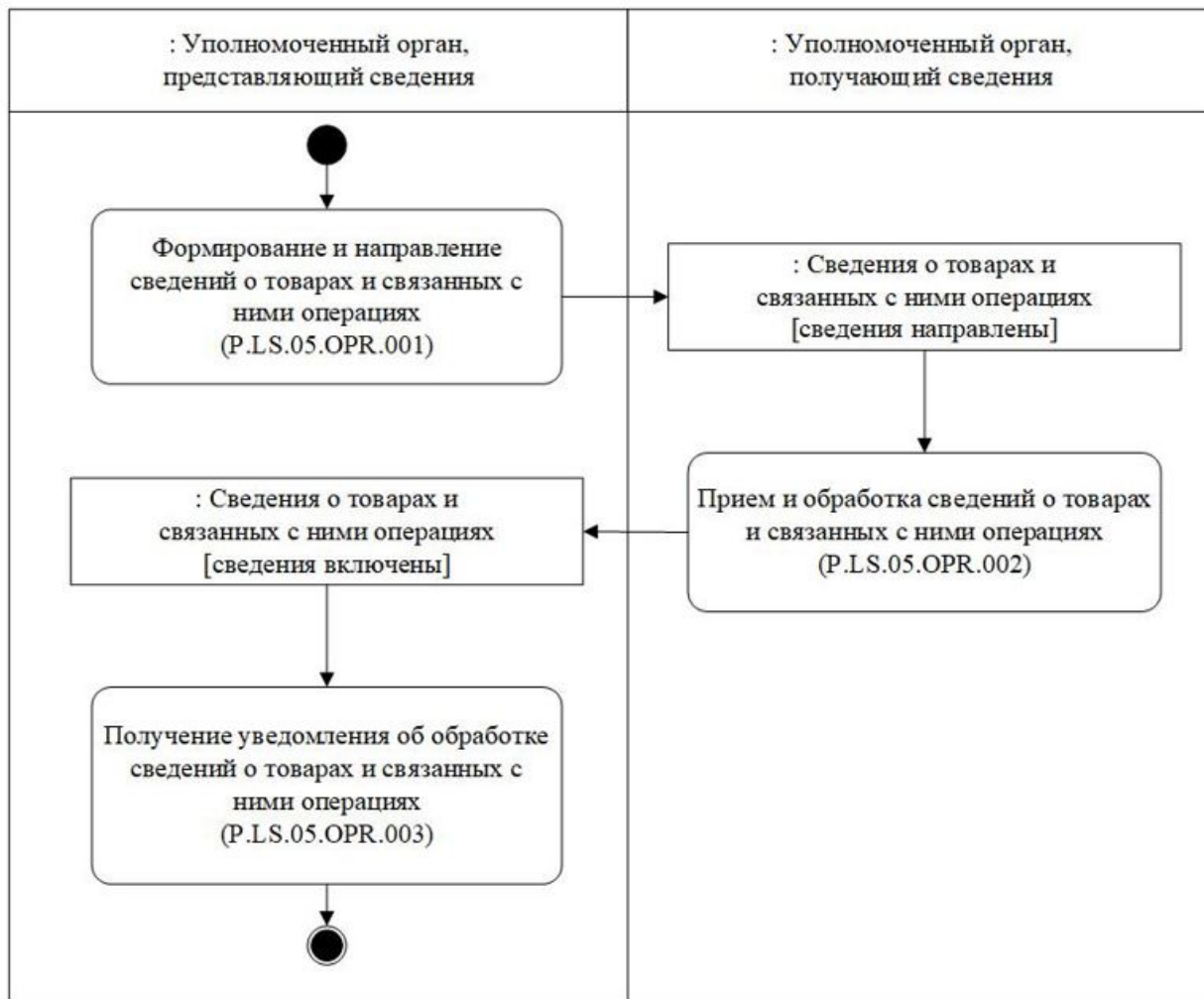
Рис. 5. Схема выполнения процедуры "Представление сведений о товарах и связанных с ними операциях" (P.LS.05.PRC.001)
