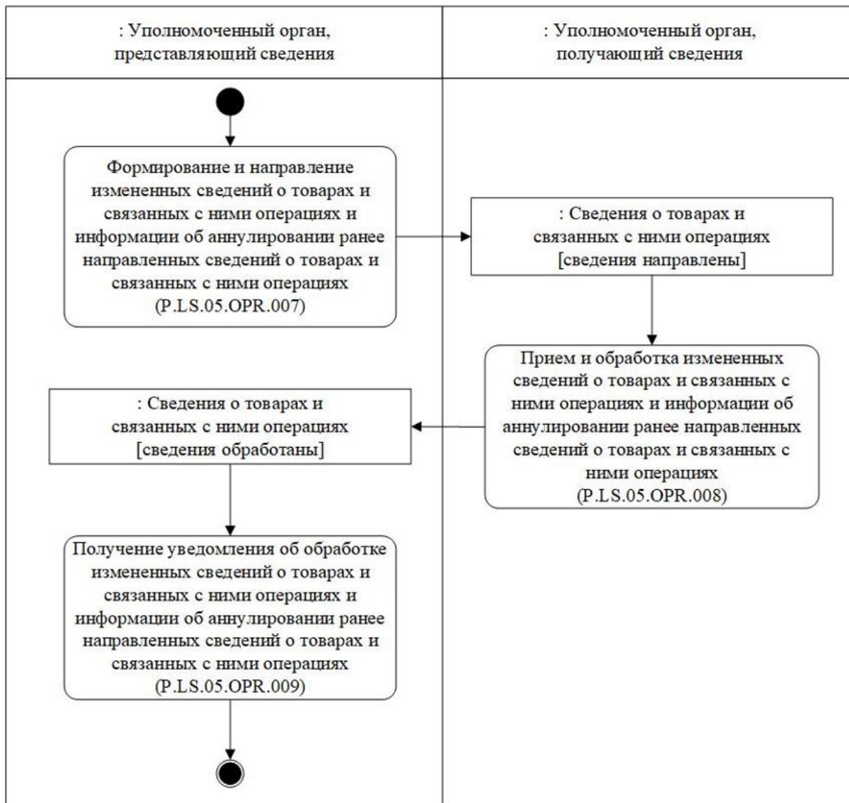
Рис. 7. Схема выполнения процедуры "Представление измененных сведений о товарах и связанных с ними операциях и информации об аннулировании ранее направленных сведений о товарах и связанных с ними операциях" (P.L.S.05.PRC.003)
