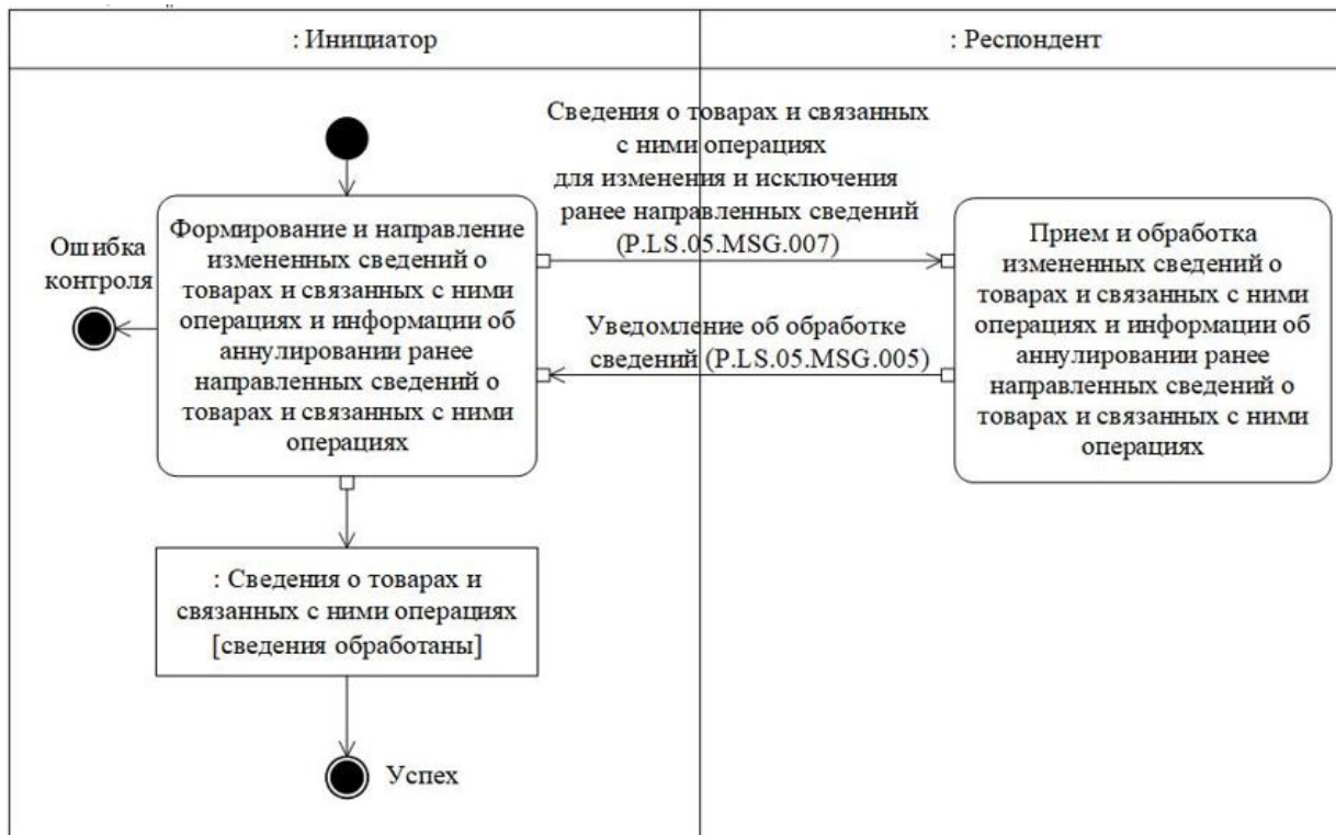
Рис. 6. Схема выполнения транзакции общего процесса "Представление сведений о товарах и связанных с ними операциях для изменения и исключения ранее направленных сведений" (P.LS.05.TRN.004)
