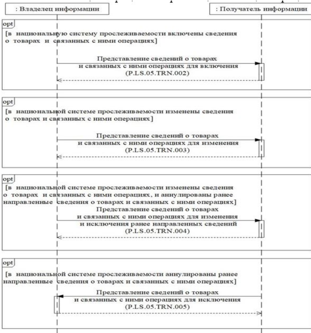
Рис. 2. Схема выполнения транзакций общего процесса при представлении сведений о товарах, подлежащих прослеживаемости, и связанных с оборотом таких товаров операциях
