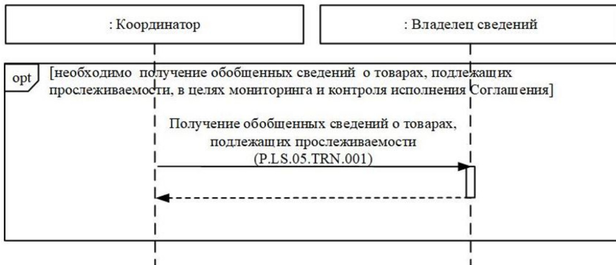
Рис. 2. Схема выполнения транзакций общего процесса при получении Комиссией сведений в целях осуществления контроля и мониторинга исполнения Соглашения
