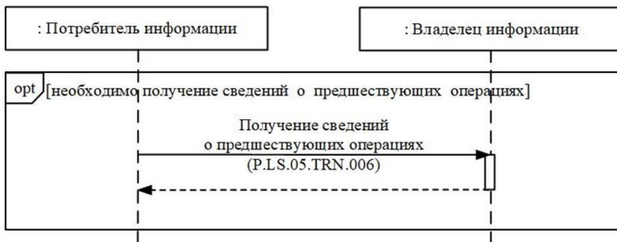
Рис. 3. Схема выполнения транзакций общего процесса при получении сведений об операциях, предшествующих перемещению товаров, подлежащих прослеживаемости
