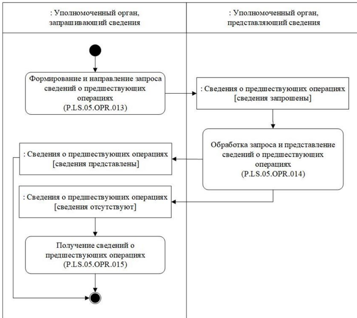
Рис. 9. Схема выполнения процедуры "Получение сведений об операциях, предшествующих перемещению товаров, подлежащих прослеживаемости" (P.LS.05.PRC.005)
