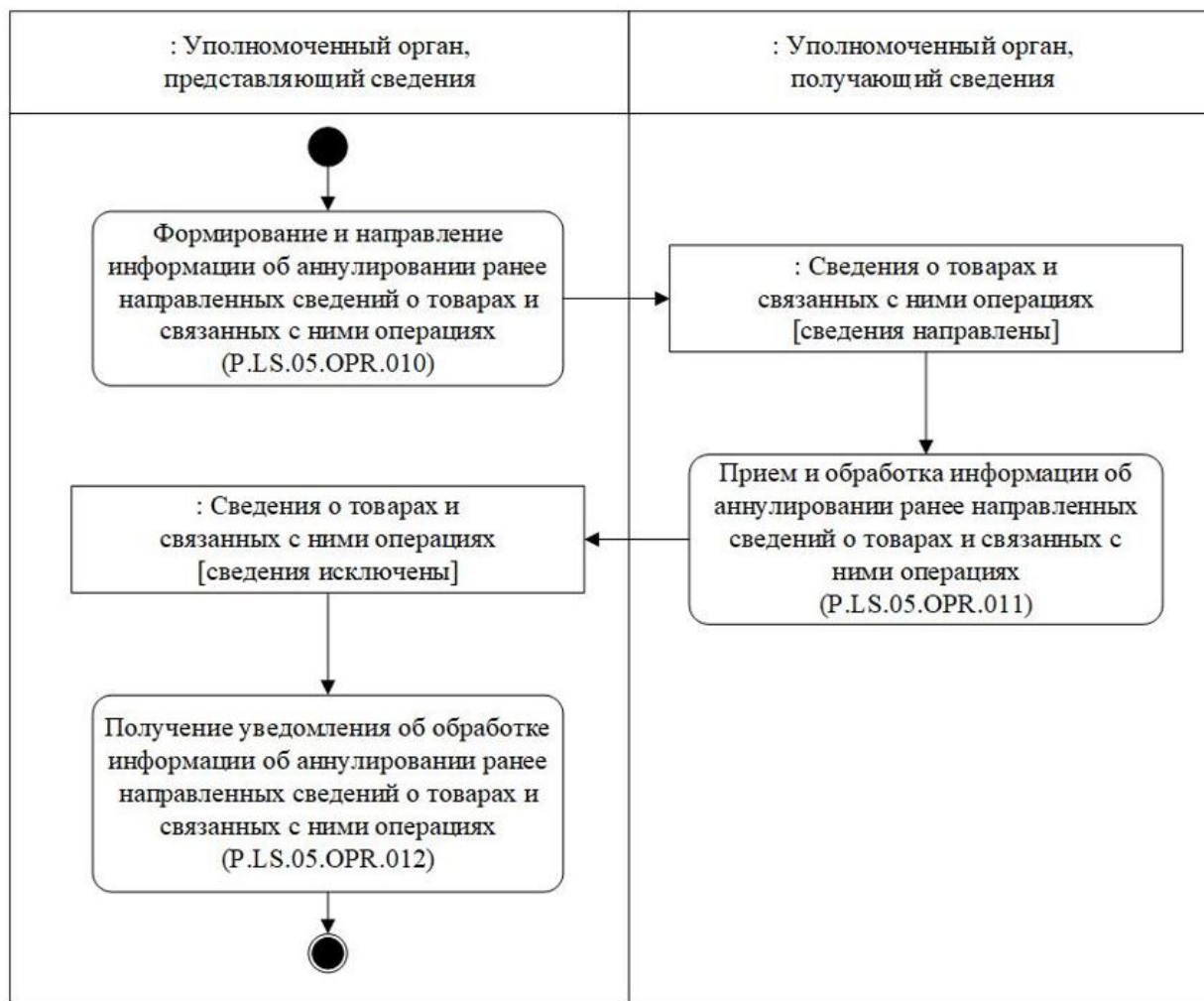
Рис. 8. Схема выполнения процедуры "Представление информации об отзыве ранее направленных сведений о товарах и связанных с ними операциях" (P.LS.05.PRC.004)
