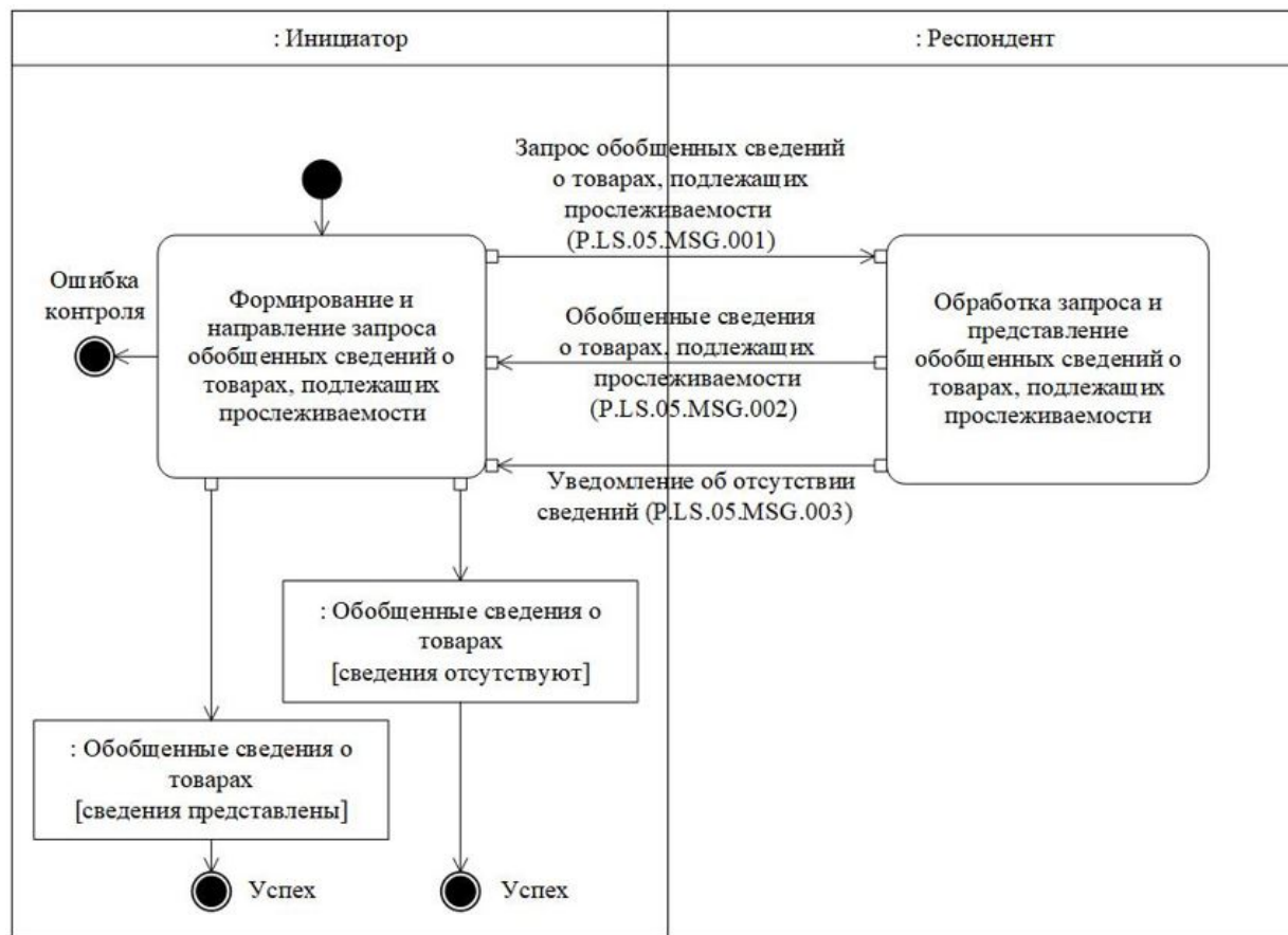
Рис. 3. Схема выполнения транзакции общего процесса "Получение обобщенных сведений о товарах, подлежащих прослеживаемости" (P.L.S.05.TRN.001)
