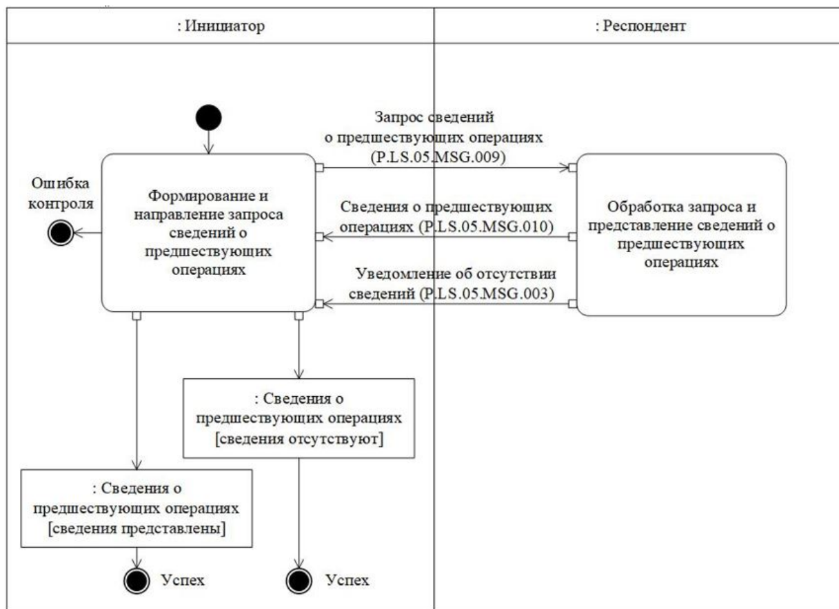
Рис. 8. Схема выполнения транзакции общего процесса "Получение сведений о предшествующих операциях" (P.L.S.05.TRN.006)
