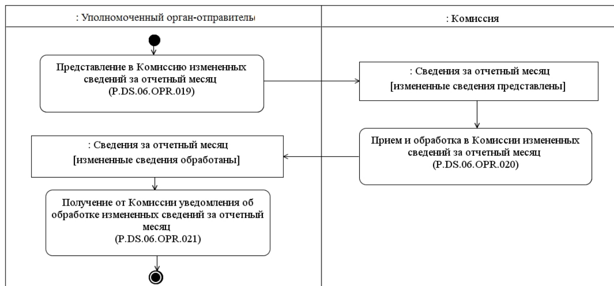
Рис. 6. Схема выполнения процедуры "Представление уполномоченными органами в Комиссию измененных сведений за отчетный месяц" (P.DS.06.PRC.005)
