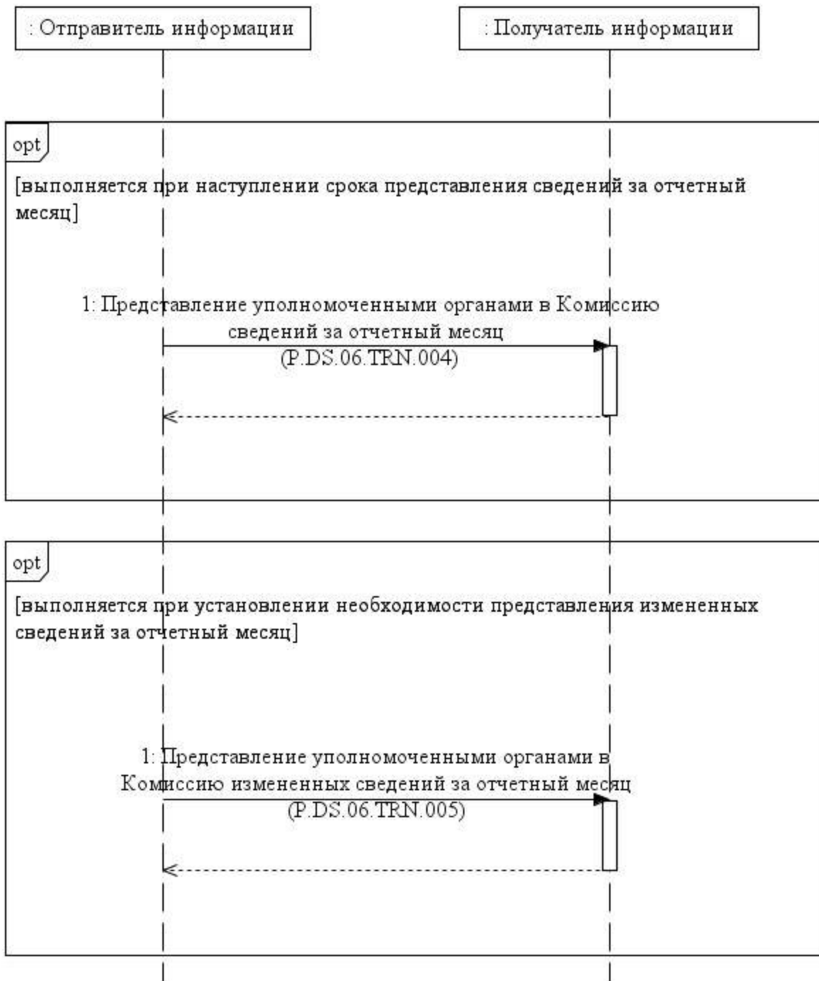
Рис. 2. Схема выполнения транзакций общего процесса при предоставлении сведений уполномоченными органами в Комиссию
