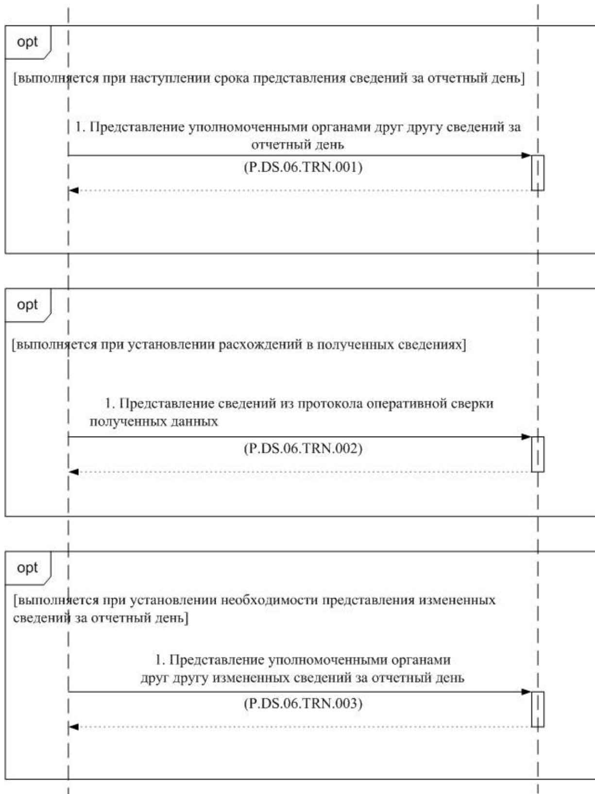
Рис. 2. Схема выполнения транзакций общего процесса при представлении сведений уполномоченными органами друг другу
