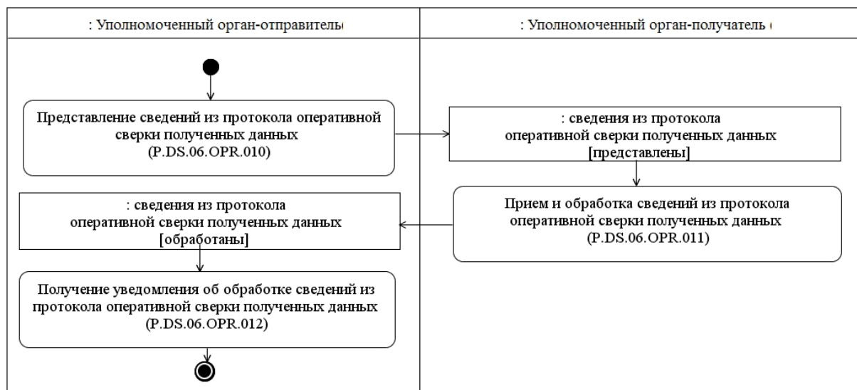
Рис. 4. Схема выполнения процедуры "Представление уполномоченными органами друг другу сведений из протокола оперативной сверки полученных данных" (P.DS.06.PRC.003)
