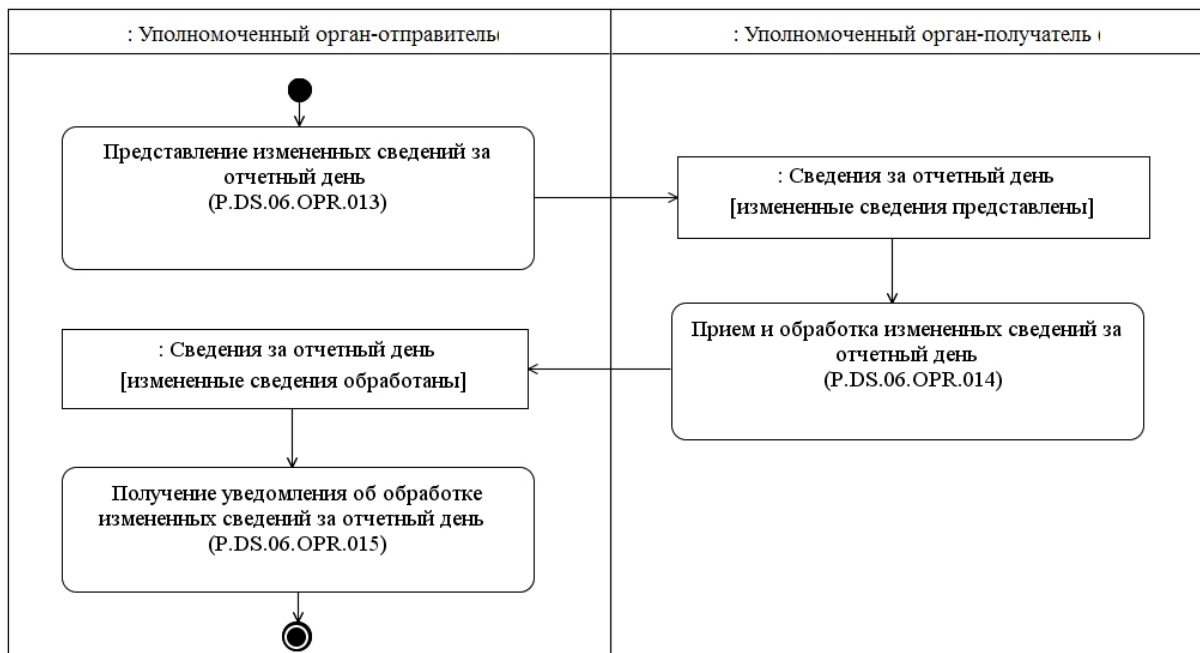
Рис. 5. Схема выполнения процедуры "Представление уполномоченными органами друг другу измененных сведений за отчетный день" (P.DS.06.PRC.004)
