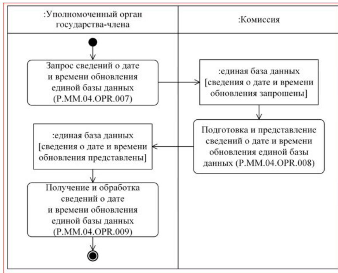
Рис. 6. Схема выполнения процедуры "Получение сведений о дате и времени обновления единой базы данных" (Р.ММ.04.PRC.003)
