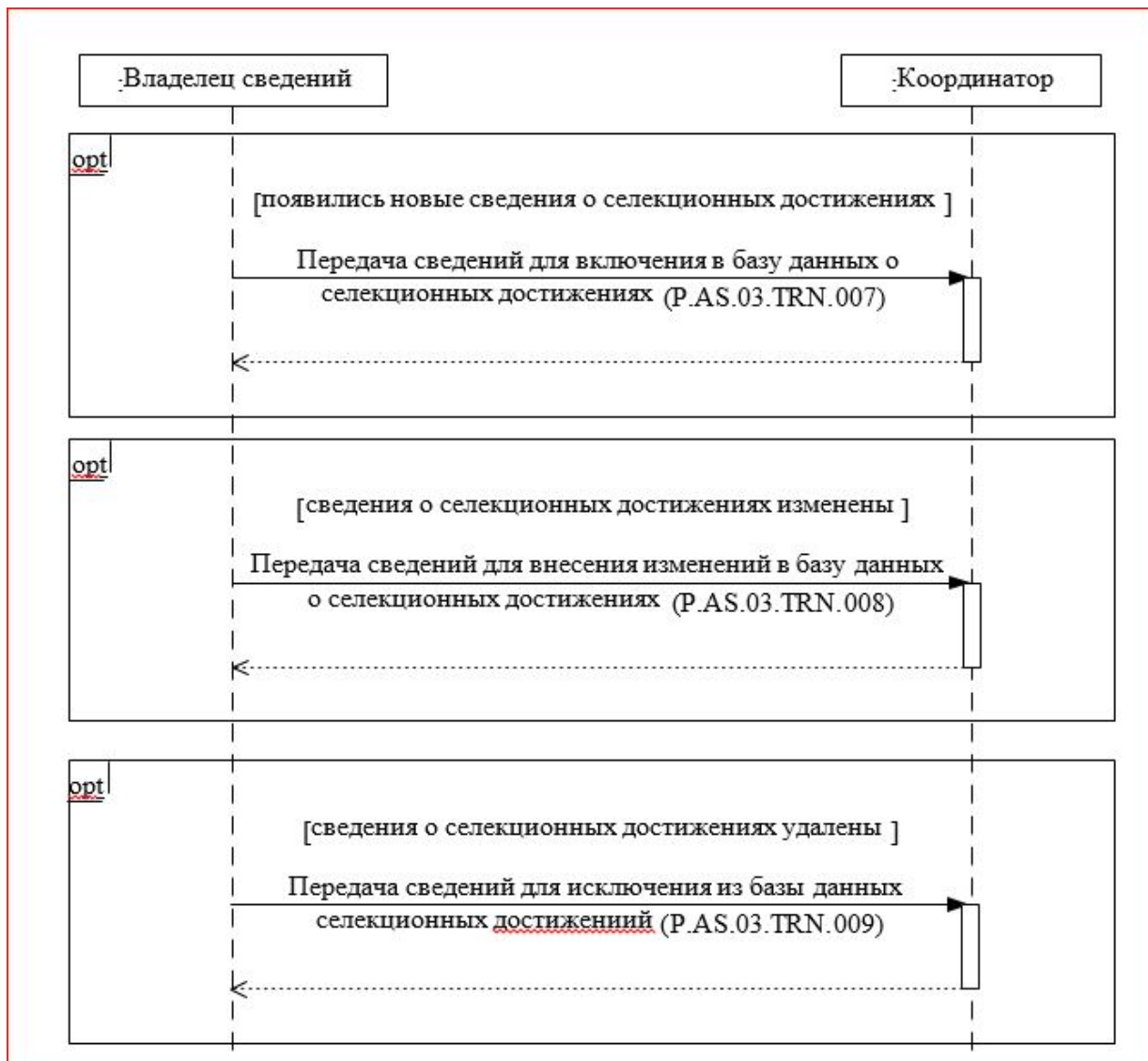
Рис. 4. Схема выполнения транзакций общего процесса при формировании и ведении базы данных о селекционных достижениях
