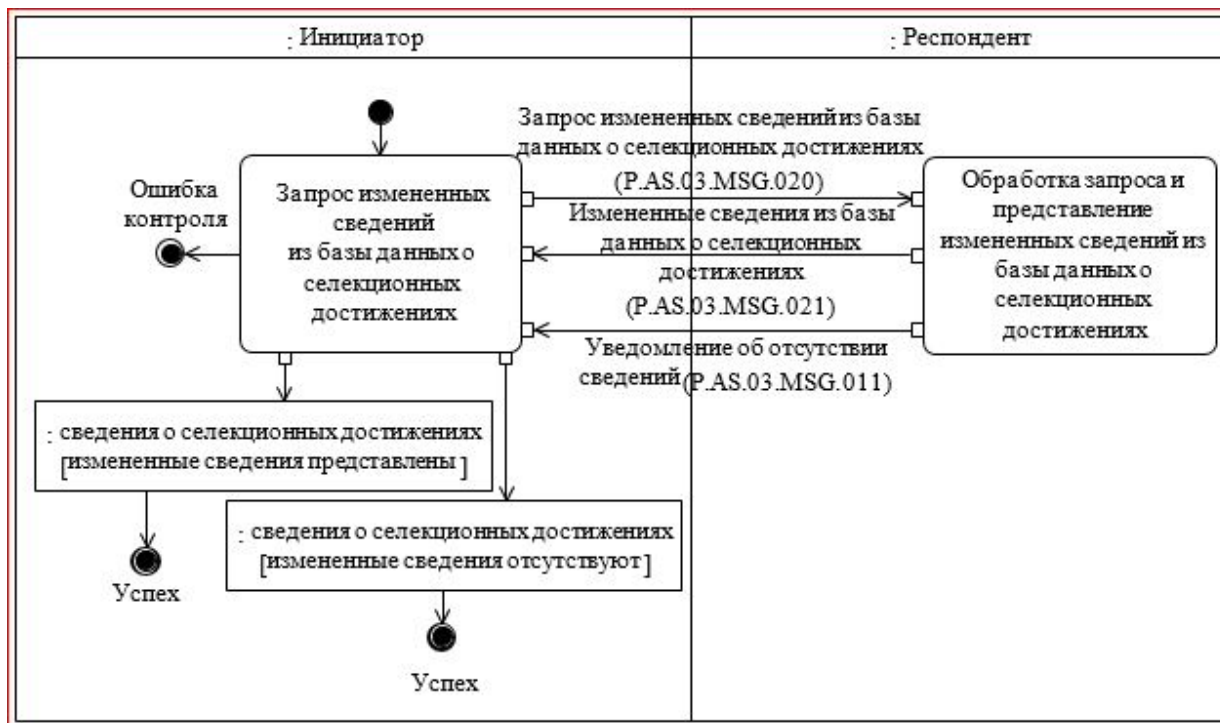
Рис. 17. Схема выполнения транзакции общего процесса "Получение измененных сведений из базы данных о селекционных достижениях" (P.AS.03.TRN.012)
