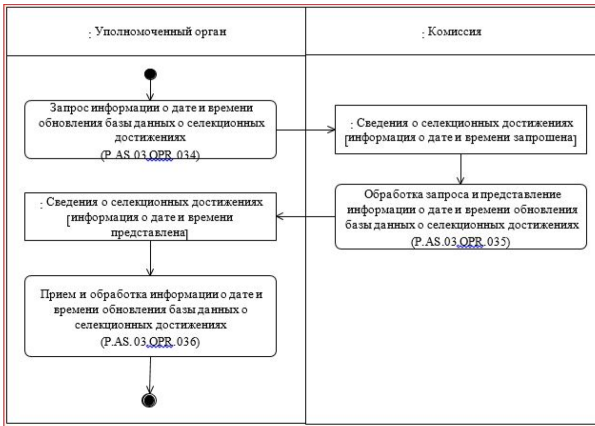
Рис. 15. Схема выполнения процедуры "Получение информации о дате и времени обновления базы данных о селекционных достижениях" (P.AS.03.PRC.010)
