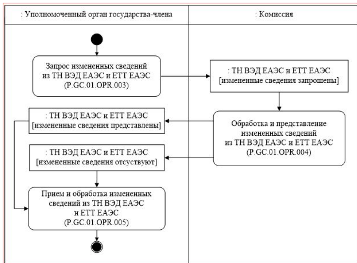
Рис. 3. Схема выполнения процедуры "Получение измененных сведений из ТН ВЭД ЕАЭС и ЕТТ ЕАЭС по запросам уполномоченных органов государств-членов" (P.GC.01.PRC.002)
