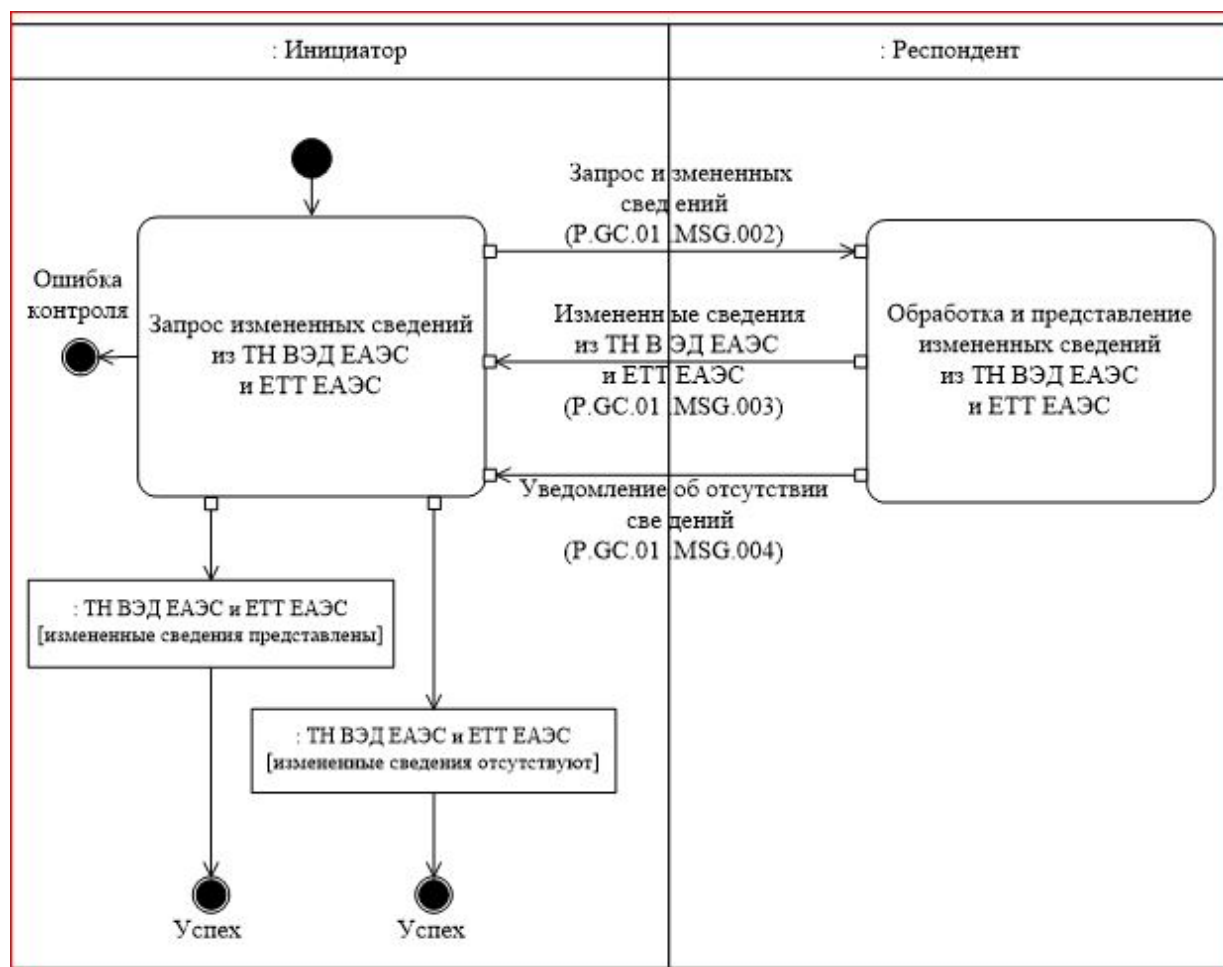
Рис. 5. Схема выполнения транзакции общего процесса "Получение измененных сведений из ТН ВЭД ЕАЭС и ЕТТ ЕАЭС" (P.GC.01.TRN.002)
