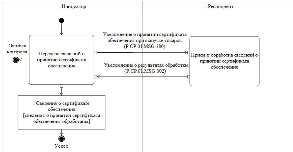
Рис. 53. Схема выполнения транзакции общего процесса "Представление сведений о принятии сертификата обеспечения" (P.SP.01.TRN.038)
