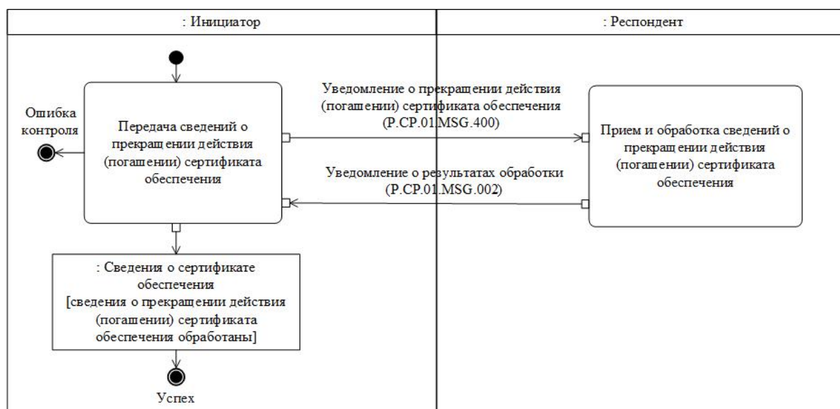
Рис. 55. Схема выполнения транзакции общего процесса "Представление сведений о прекращении действия (погашении) сертификата обеспечения" (P.SP.01.TRN.040)
