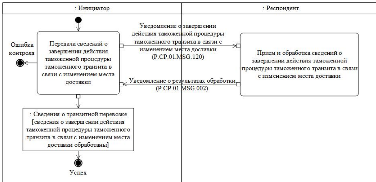
Рис. 20. Схема выполнения транзакции общего процесса "Представление сведений о завершении действия таможенной процедуры таможенного транзита в связи с изменением места доставки" (P.CP.01.TRN.005)
