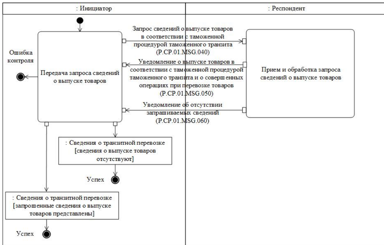
Рис. 19. Схема выполнения транзакции общего процесса "Запрос сведений о выпуске товаров" (P.SP.01.TRN.004)
