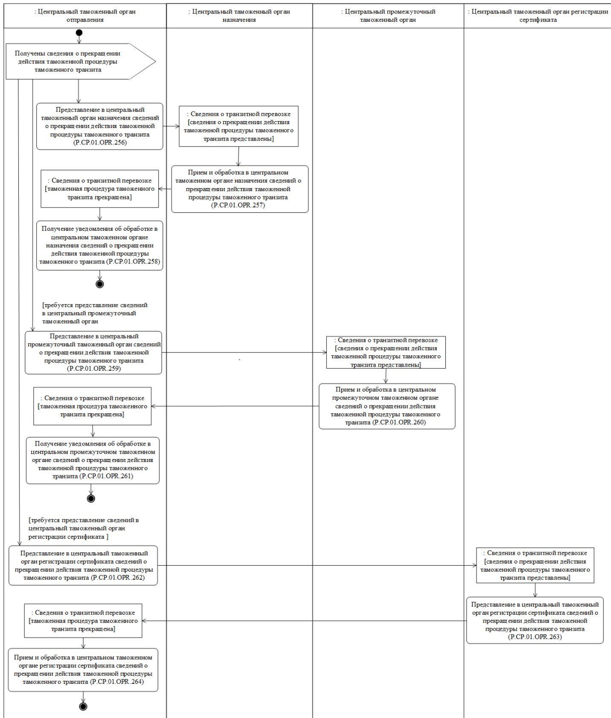
Рис. 41. Схема выполнения процедуры "Информирование о прекращении действия таможенной процедуры таможенного транзита" (P.CP.01.PRC.035)
