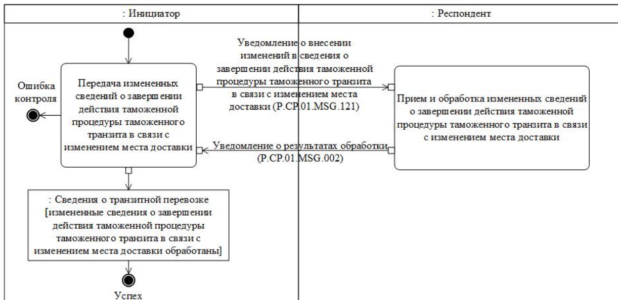
Рис. 21. Схема выполнения транзакции общего процесса "Представление измененных сведений о завершении действия таможенной процедуры таможенного транзита в связи с изменением места доставки" (P.SP.01.TRN.006)
