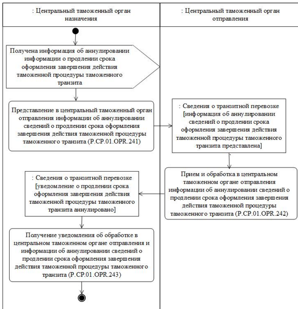
Рис. 37. Схема выполнения процедуры "Аннулирование сведений о продлении срока оформления завершения действия таможенной процедуры таможенного транзита" (Р.СР.01.ПРС.031)
