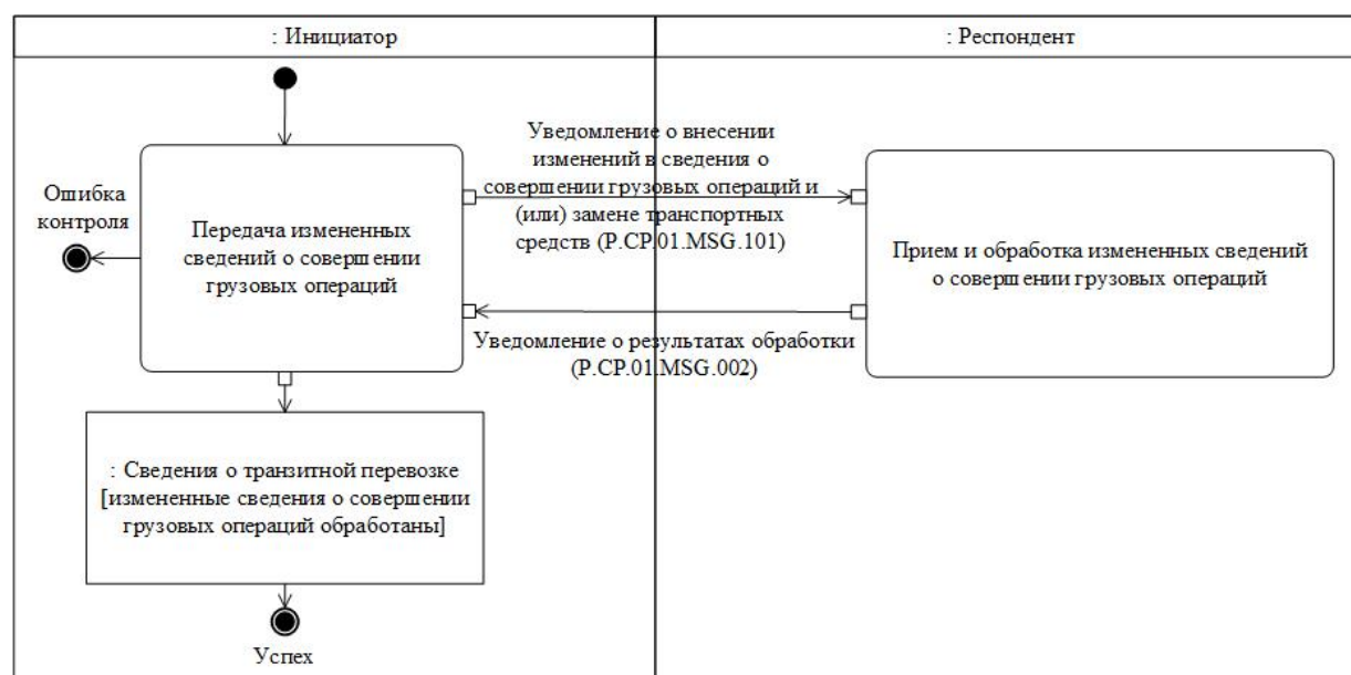
Рис. 36. Схема выполнения транзакции общего процесса "Представление измененных сведений о совершении грузовых операций" (P.SP.01.TRN.021)
