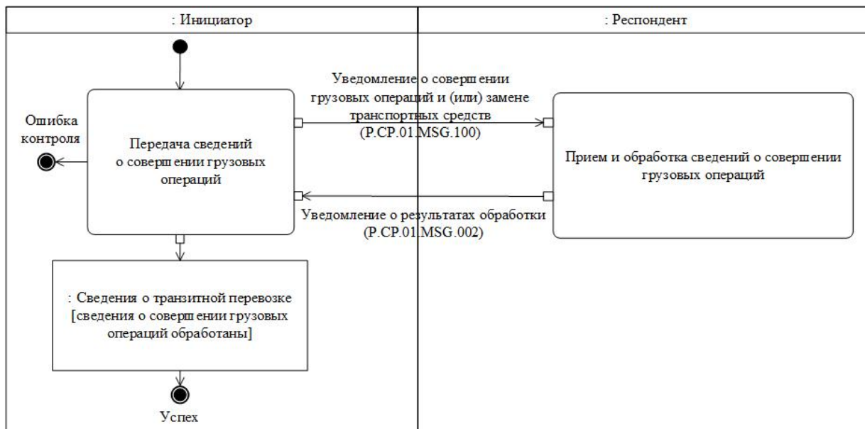
Рис. 35. Схема выполнения транзакции общего процесса "Представление сведений о совершении грузовых операций" (P.SP.01.TRN.020)
