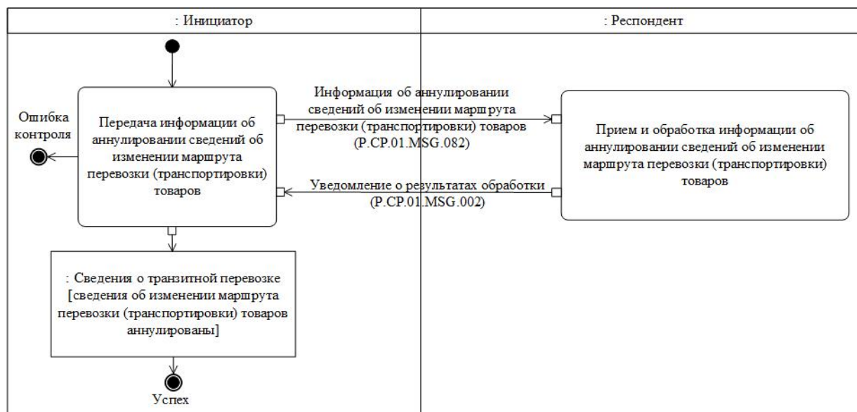
Рис. 31. Схема выполнения транзакции общего процесса "Представление информации об аннулировании сведений об изменении маршрута перевозки (транспортировки) товаров" (P.SP.01.TRN.016)
