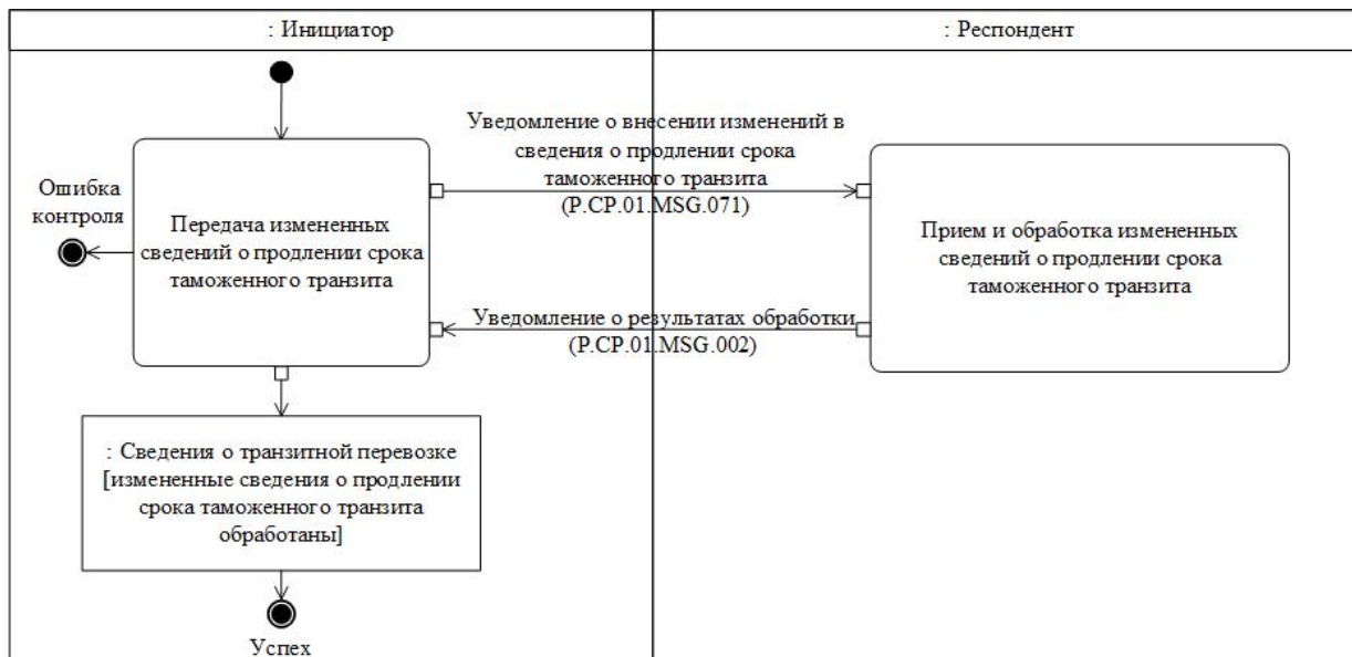
Рис. 27. Схема выполнения транзакции общего процесса "Представление измененных сведений о продлении срока таможенного транзита" (P.SP.01.TRN.012)
