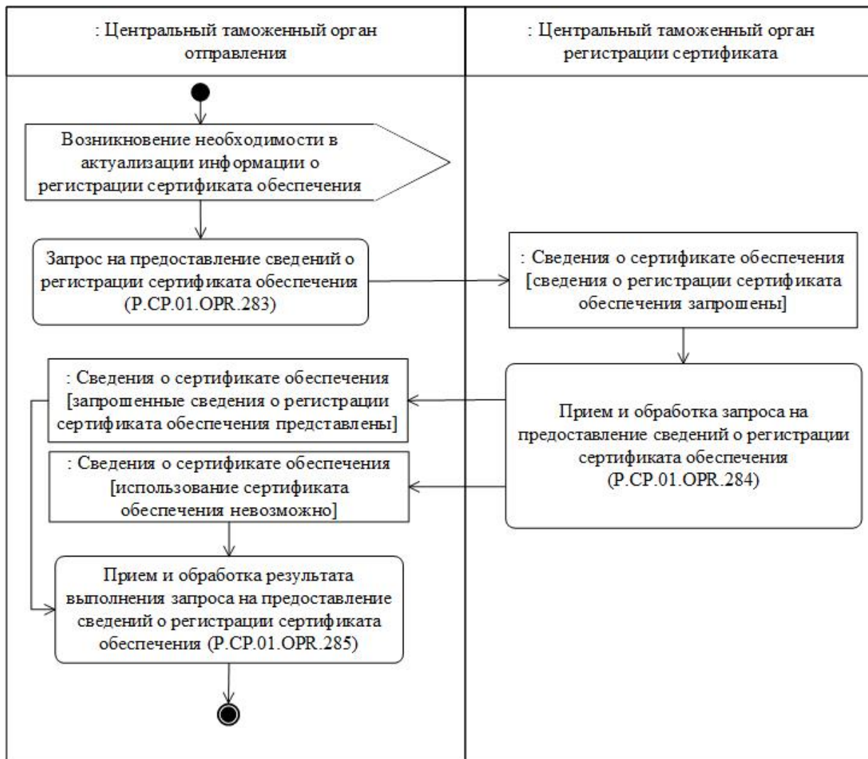
Рис. 46. Схема выполнения процедуры "Запрос сведений о регистрации сертификата обеспечения" (P.SP.01.PRC.040)
