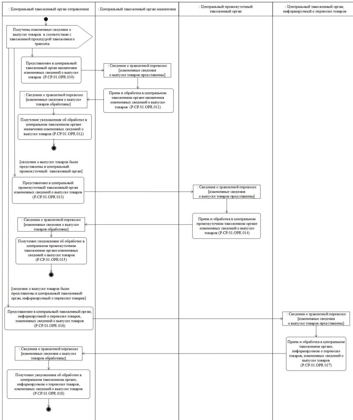
Рис. 8. Схема выполнения процедуры "Изменение сведений о выпуске товаров" (P.CP.01.PRC.002)
