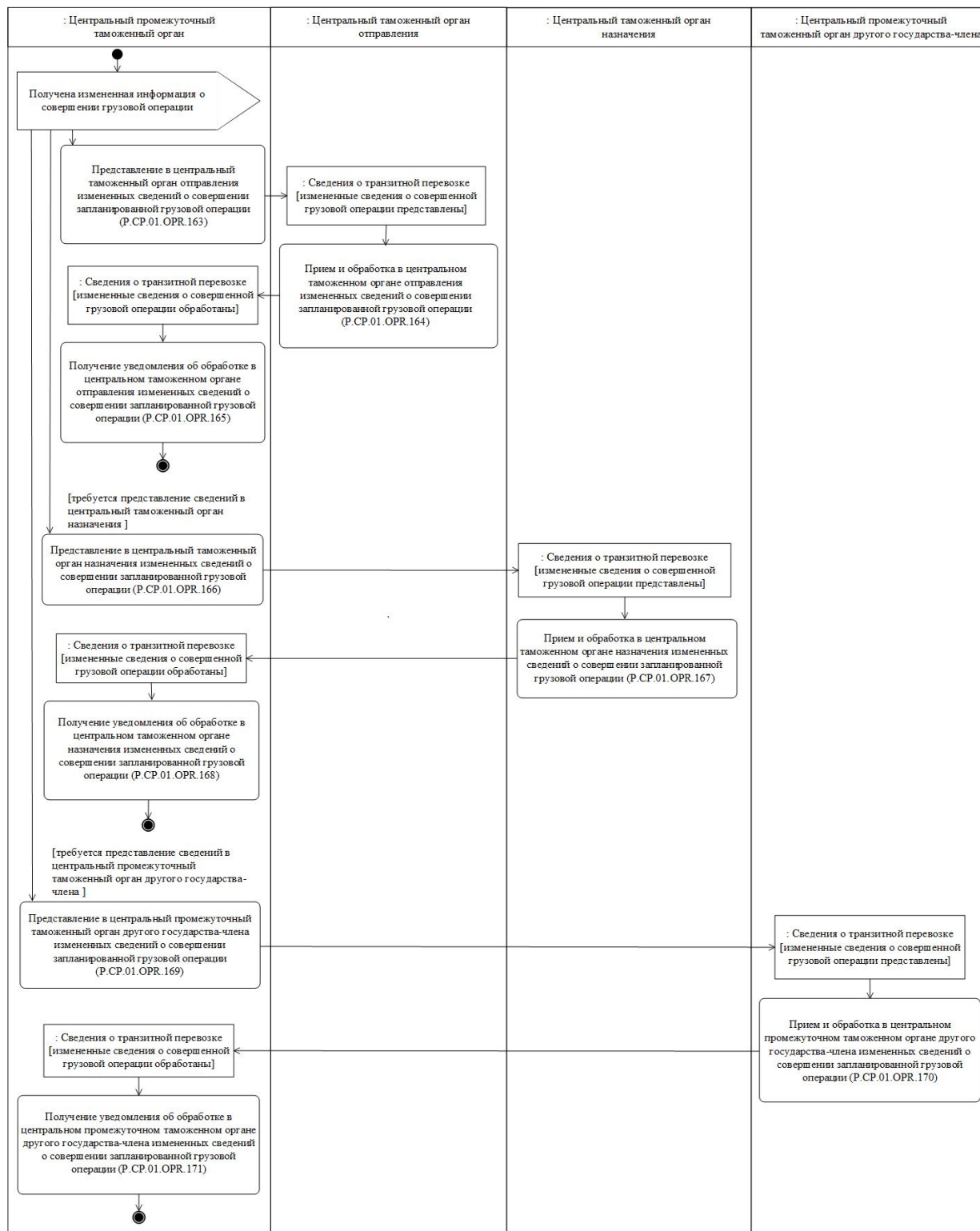
Рис. 27. Схема выполнения процедуры "Изменение сведений о совершении запланированных грузовых операций" (Р.СР.01.ПРС.021)
