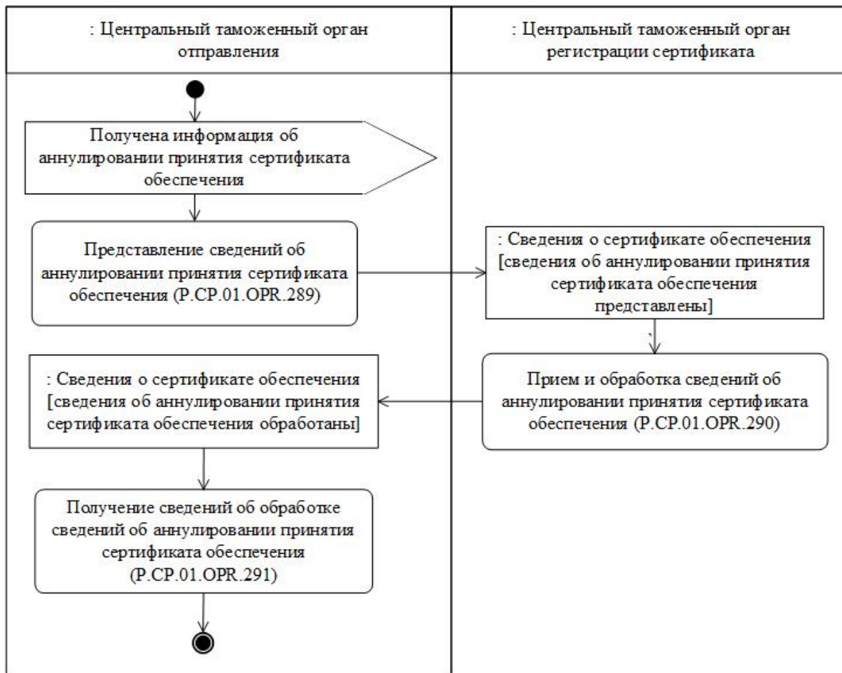
Рис. 48. Схема выполнения процедуры "Информирование об аннулировании принятия сертификата обеспечения" (Р.СР.01.ПРС.042)
