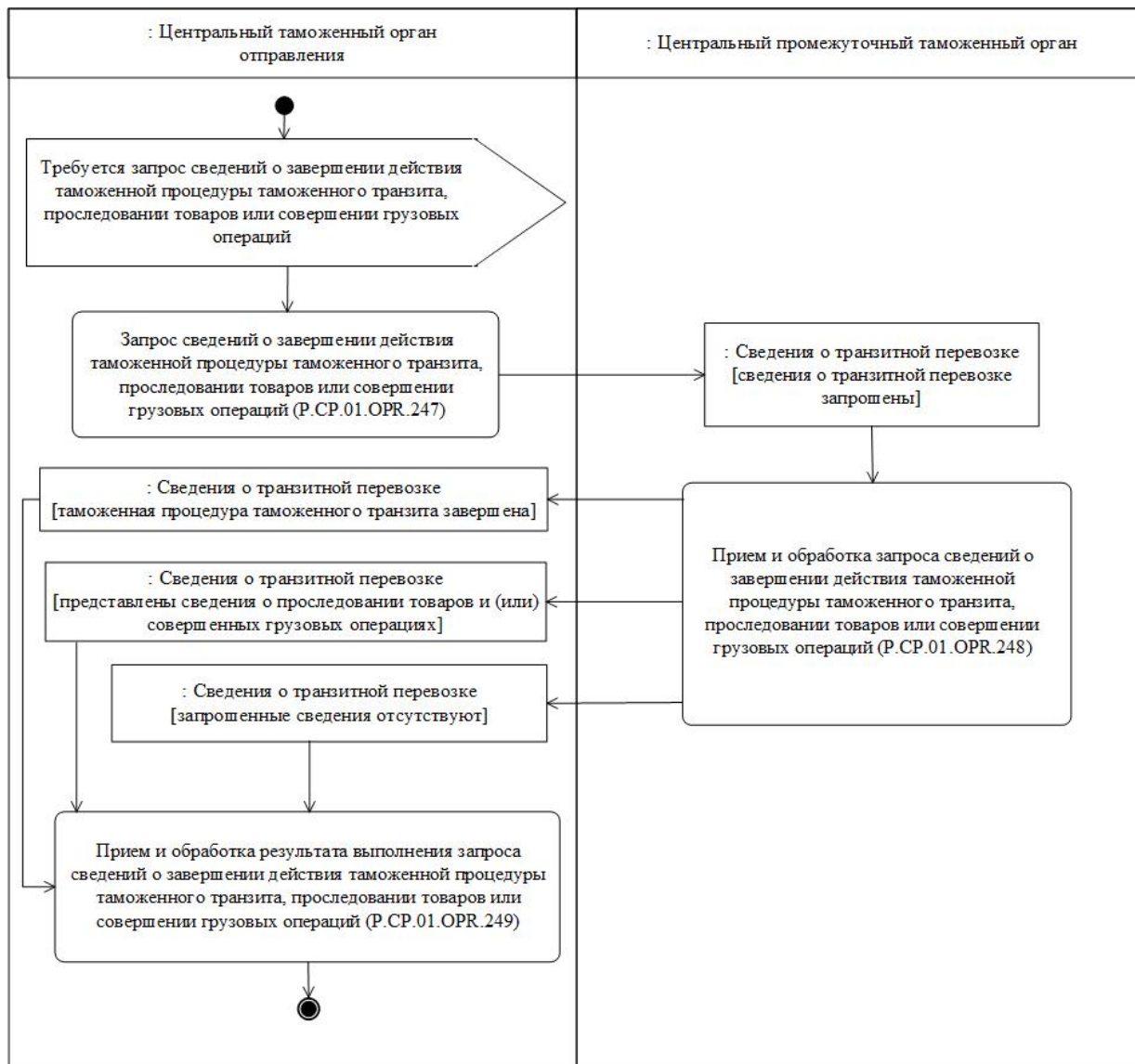
Рис. 39. Схема выполнения процедуры "Запрос сведений о завершении действия таможенной процедуры таможенного транзита, проследовании товаров или совершении грузовых операций" (Р.СР.01.ПРС.033)
