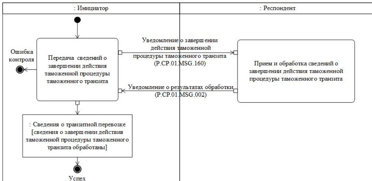
Рис. 22. Схема выполнения транзакции общего процесса "Представление сведений о завершении действия таможенной процедуры таможенного транзита" (P.SP.01.TRN.007)
