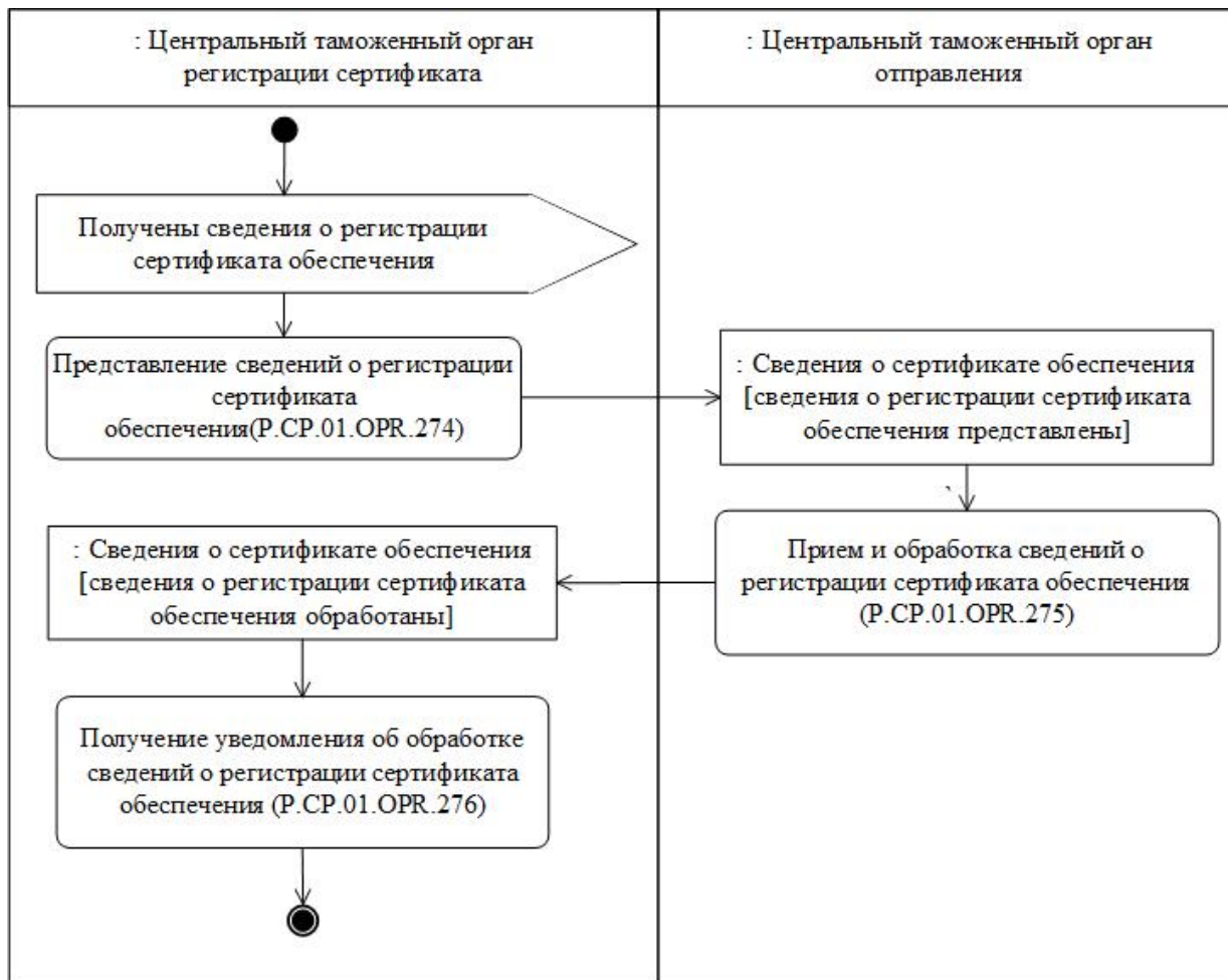
Рис. 43. Схема выполнения процедуры "Информирование о регистрации сертификата обеспечения" (Р.СР.01.ПРС.037)
