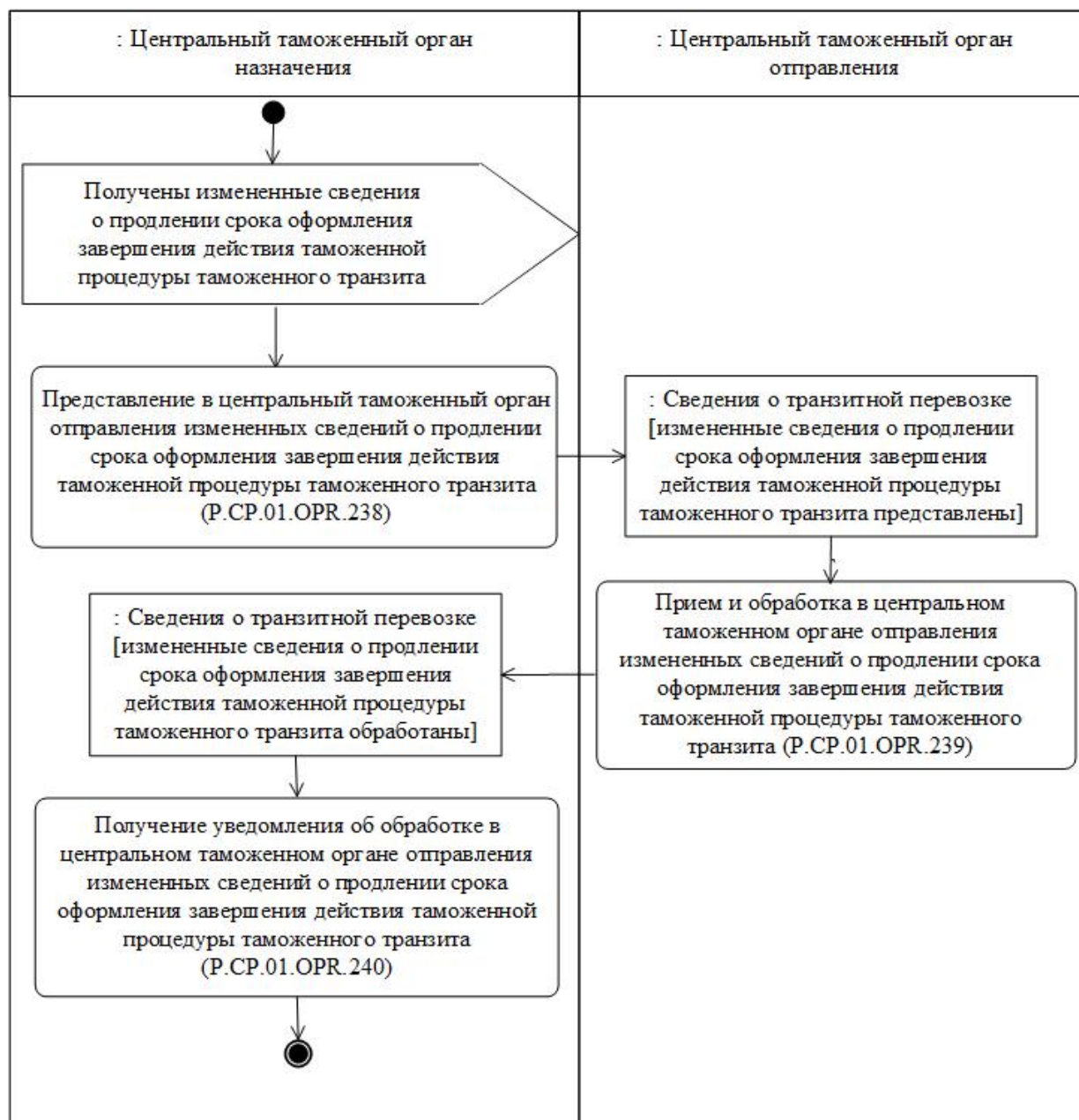
Рис. 36. Схема выполнения процедуры "Изменение сведений о продлении срока оформления завершения действия таможенной процедуры таможенного транзита" (P.SP.01.PRC.030)
