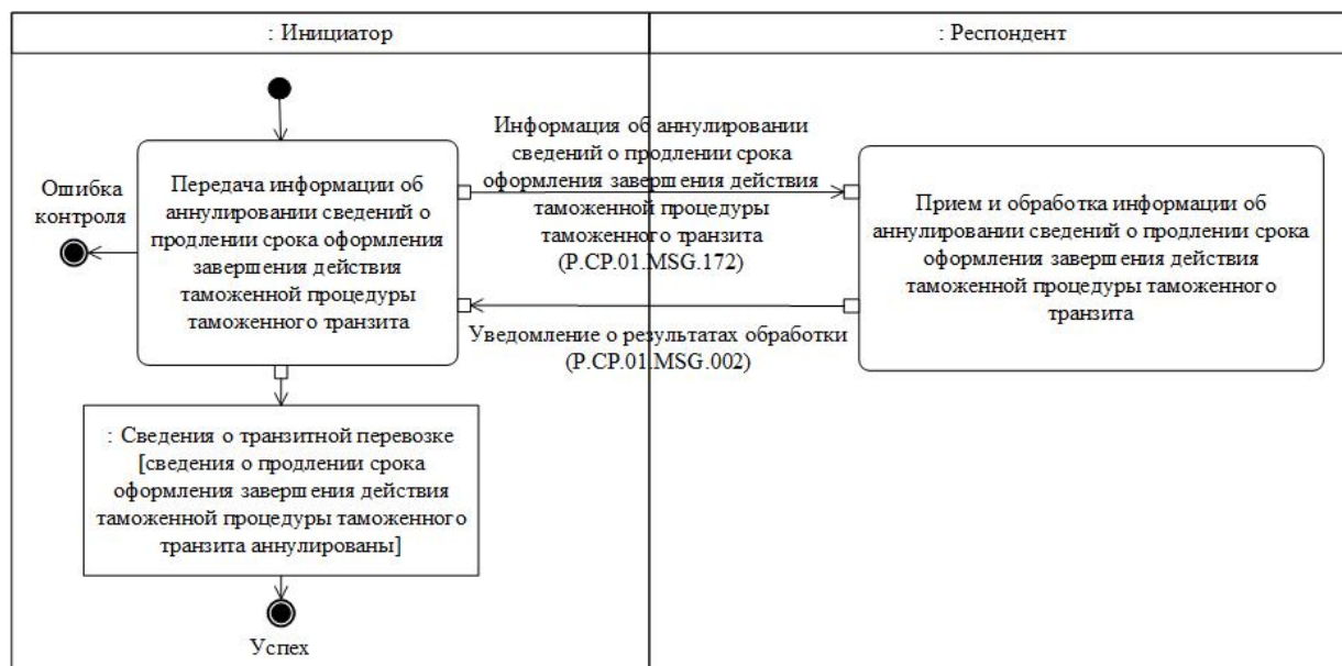
Рис. 43. Схема выполнения транзакции общего процесса "Представление информации об аннулировании сведений о продлении срока оформления завершения действия таможенной процедуры таможенного транзита" (P.CP.01.TRN.028)
