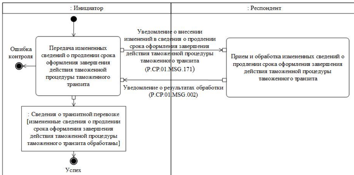
Рис. 42. Схема выполнения транзакции общего процесса "Представление измененных сведений о продлении срока оформления завершения действия таможенной процедуры таможенного транзита" (P.CP.01.TRN.027)
