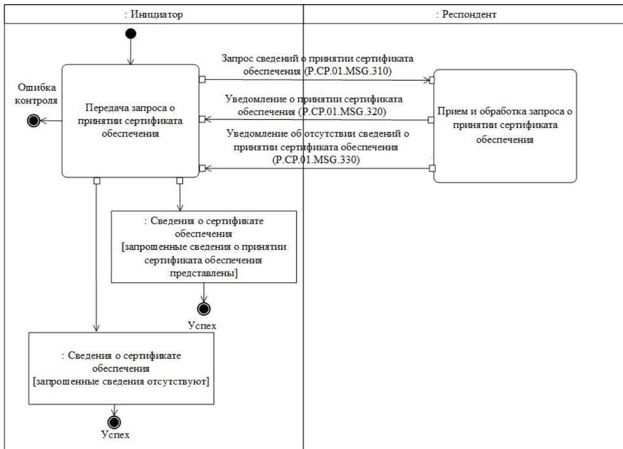
Рис. 50. Схема выполнения транзакции общего процесса "Запрос сведений о принятии сертификата обеспечения" (P.SP.01.TRN.035)
