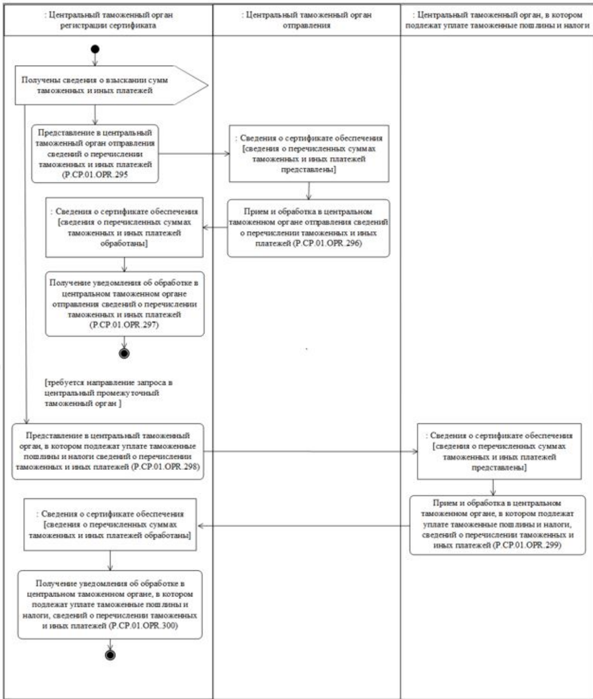
Рис. 50. Схема выполнения процедуры "Информирование о перечислении взысканных сумм таможенных и иных платежей" (Р.СР.01.ПРС.044)
