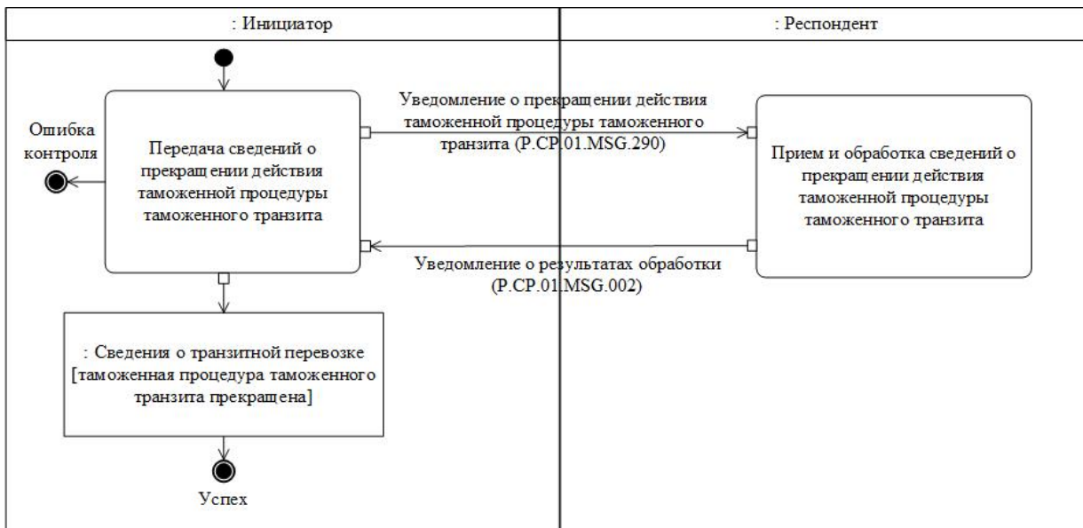
Рис. 47. Схема выполнения транзакции общего процесса "Представление сведений о прекращении действия таможенной процедуры таможенного транзита" (P.CP.01.TRN.032)
