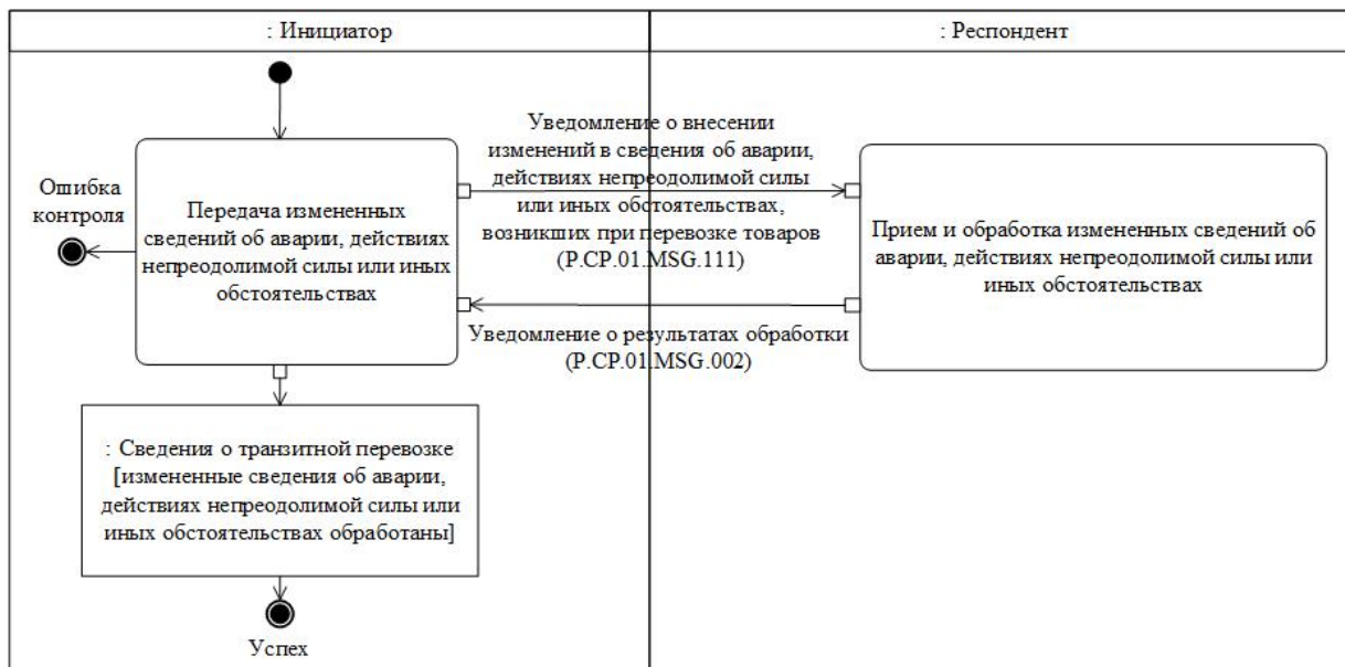
Рис. 39. Схема выполнения транзакции общего процесса "Представление измененных сведений об аварии, действиях непреодолимой силы или иных обстоятельствах" (P.SP.01.TRN.024)
