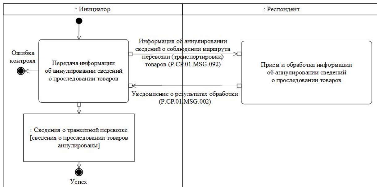
Рис. 34. Схема выполнения транзакции общего процесса "Представление информации об аннулировании сведений о проследовании товаров" (P.SP.01.TRN.019)
