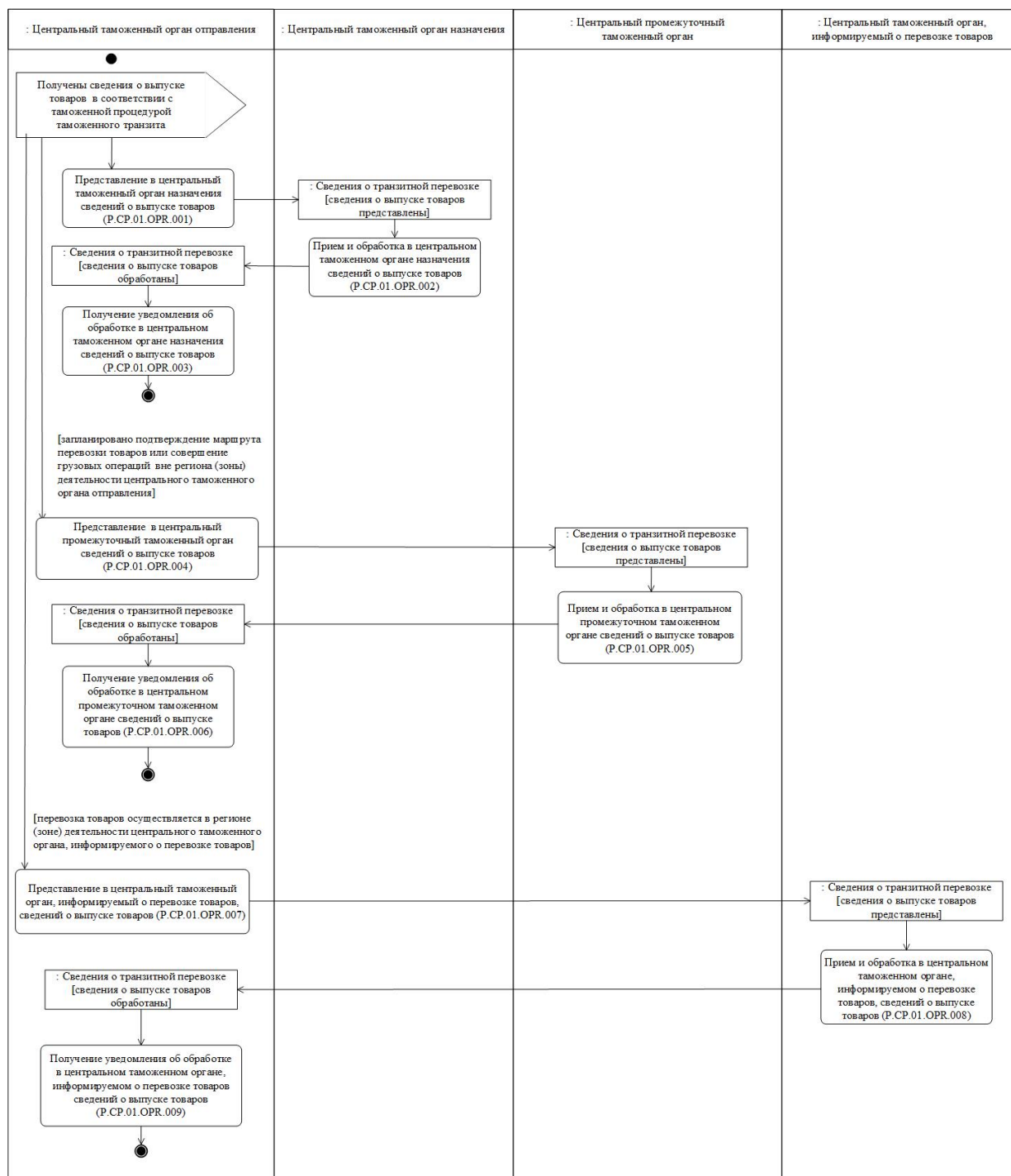
Рис. 7. Схема выполнения процедуры "Информирование о выпуске товаров в соответствии с таможенной процедурой таможенного транзита" (P.CP.01.PRC.001)
