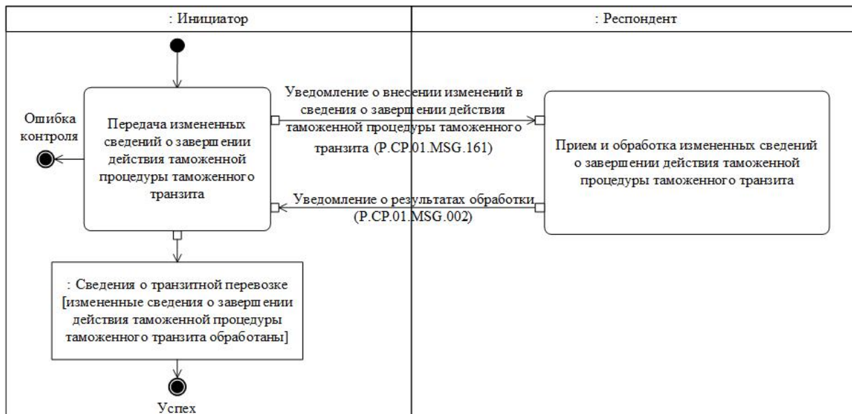
Рис. 23. Схема выполнения транзакции общего процесса "Представление измененных сведений о завершении действия таможенной процедуры таможенного транзита" (P.SP.01.TRN.008)
