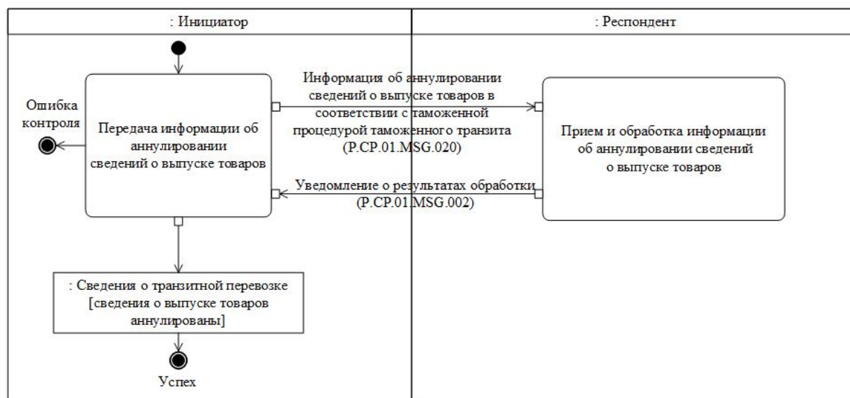
Рис. 18. Схема выполнения транзакции общего процесса "Представление информации об аннулировании сведений о выпуске товаров" (P.CP.01.TRN.003)
