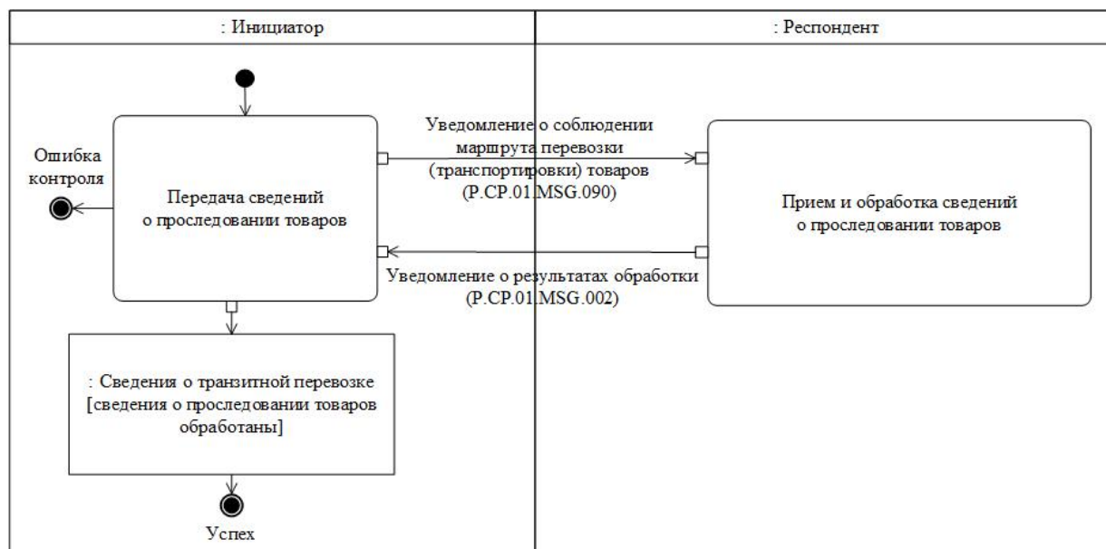
Рис. 32. Схема выполнения транзакции общего процесса "Представление сведений о проследовании товаров" (P.SP.01.TRN.017)
