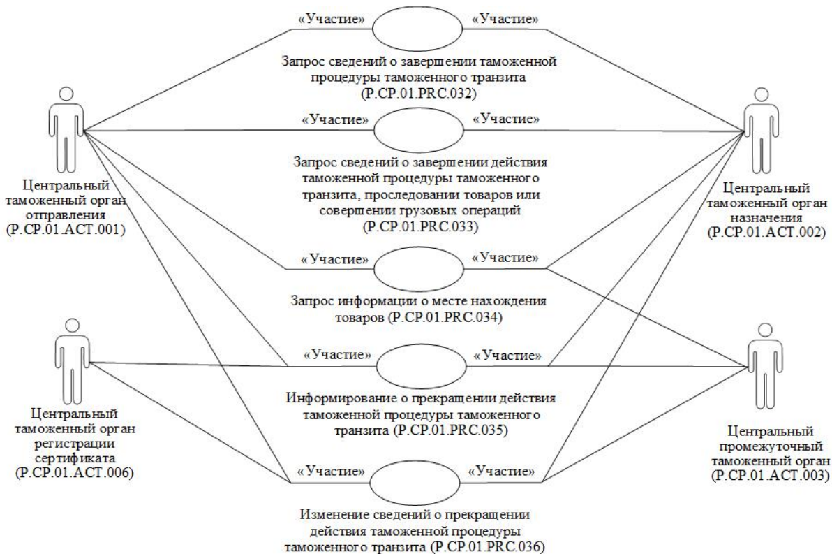
Рис. 5. Общая схема группы процедур запроса сведений о перевозке товаров в соответствии с таможенной процедурой таможенного транзита и представления сведений о прекращении действия таможенной процедуры таможенного транзита
