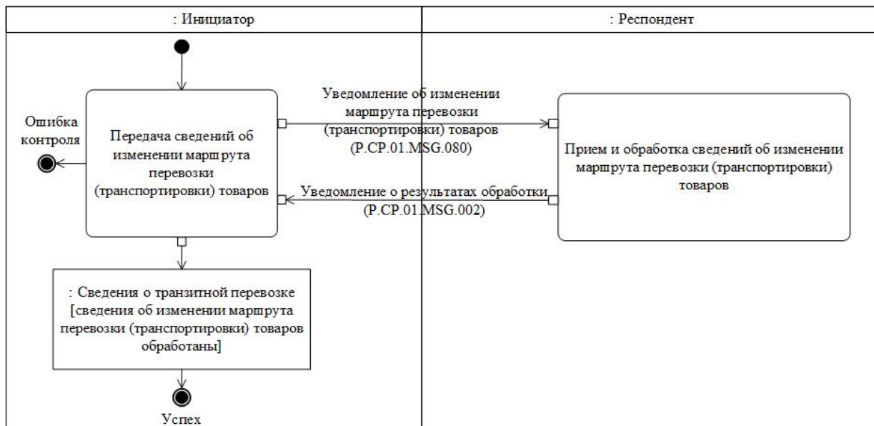
Рис. 29. Схема выполнения транзакции общего процесса "Представление сведений об изменении маршрута перевозки (транспортировки) товаров" (P.SP.01.TRN.014)
