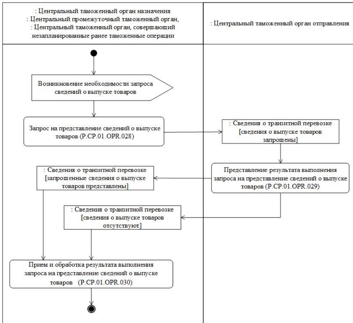
Рис. 10. Схема выполнения процедуры "Запрос сведений о выпуске товаров в соответствии с таможенной процедурой таможенного транзита" (P.SP.01.PRC.004)
