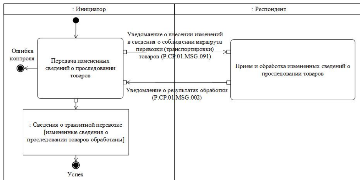
Рис. 33. Схема выполнения транзакции общего процесса "Представление измененных сведений о проследовании товаров" (P.SP.01.TRN.018)
