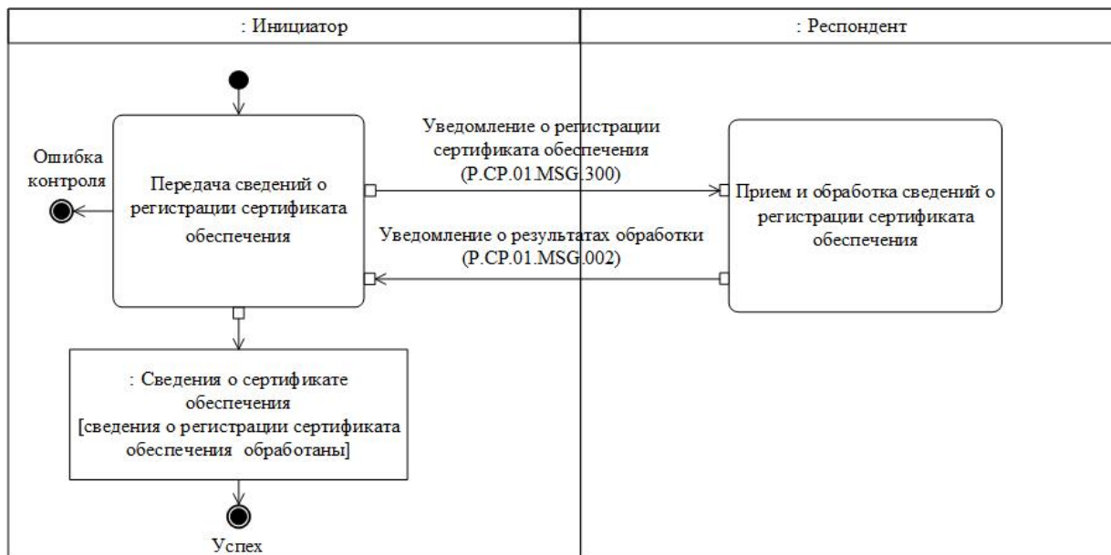
Рис. 49. Схема выполнения транзакции общего процесса "Представление сведений о регистрации сертификата обеспечения" (P.SP.01.TRN.034)
