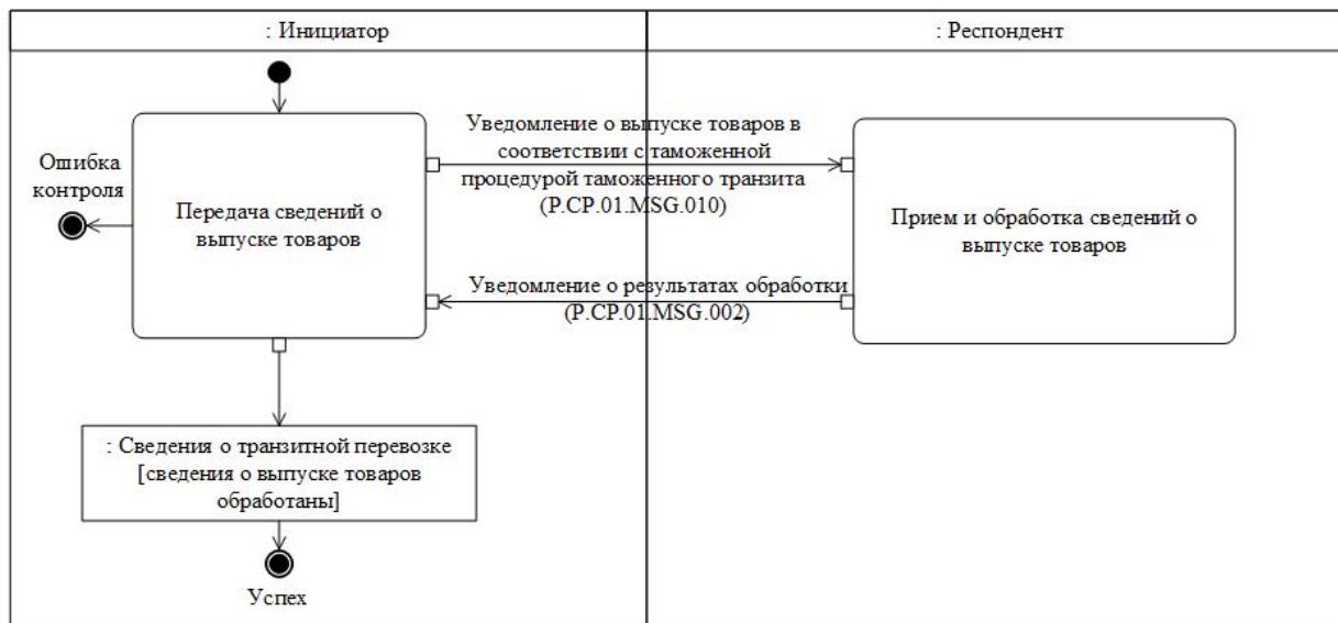
Рис. 16. Схема выполнения транзакции общего процесса "Представление сведений о выпуске товаров" (P.SP.01.TRN.001)
