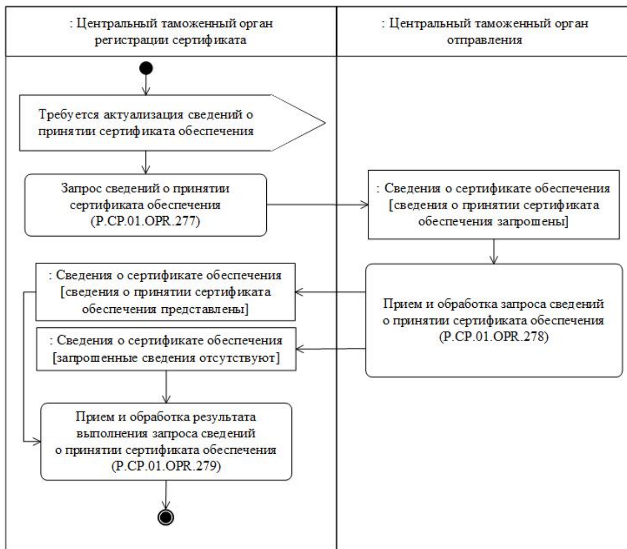
Рис. 44. Схема выполнения процедуры "Запрос сведений о принятии сертификата обеспечения" (P.SP.01.PRC.038)
