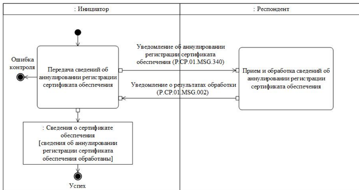
Рис. 51. Схема выполнения транзакции общего процесса "Представление сведений об аннулировании регистрации сертификата обеспечения" (P.SP.01.TRN.036)
