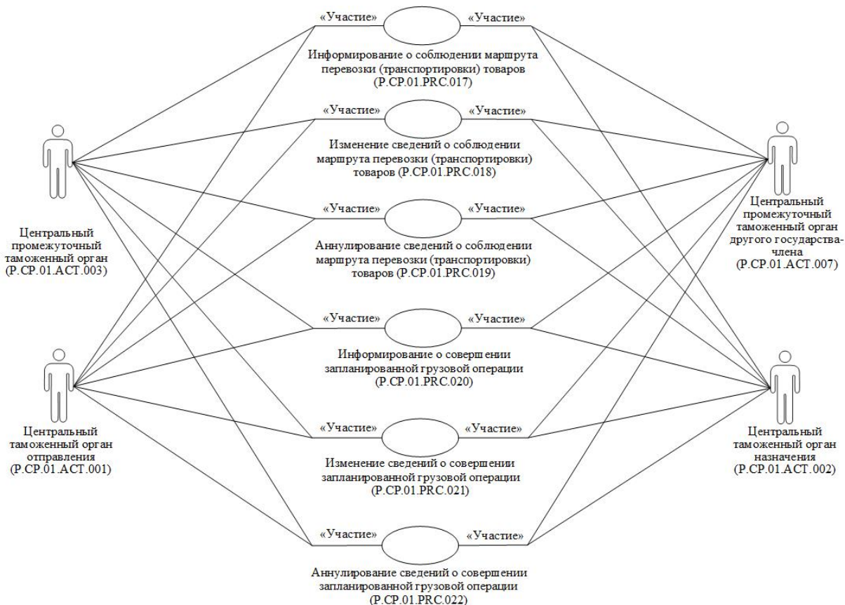
Рис. 4. Общая схема группы процедур представления сведений об операциях, совершаемых в ходе таможенной процедуры таможенного транзита (часть 1)
