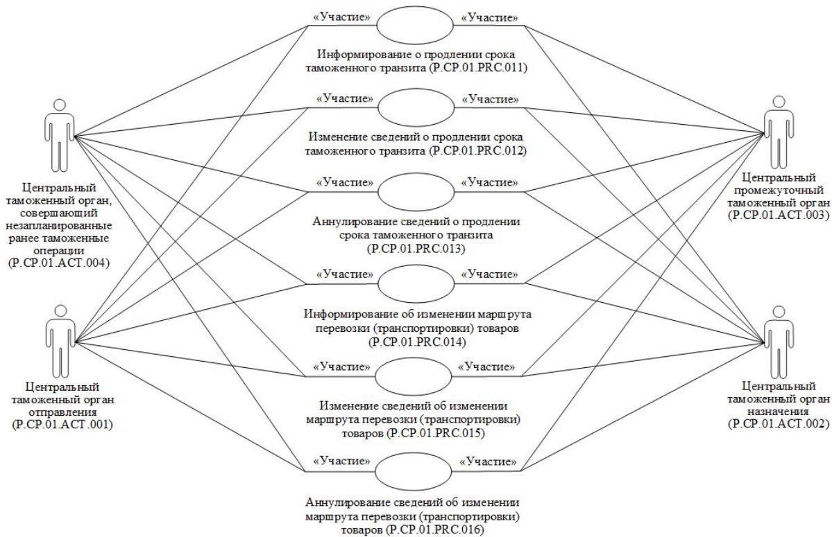
Рис. 4. Общая схема группы процедур представления сведений об операциях, совершаемых в ходе таможенной процедуры таможенного транзита (часть 1)
