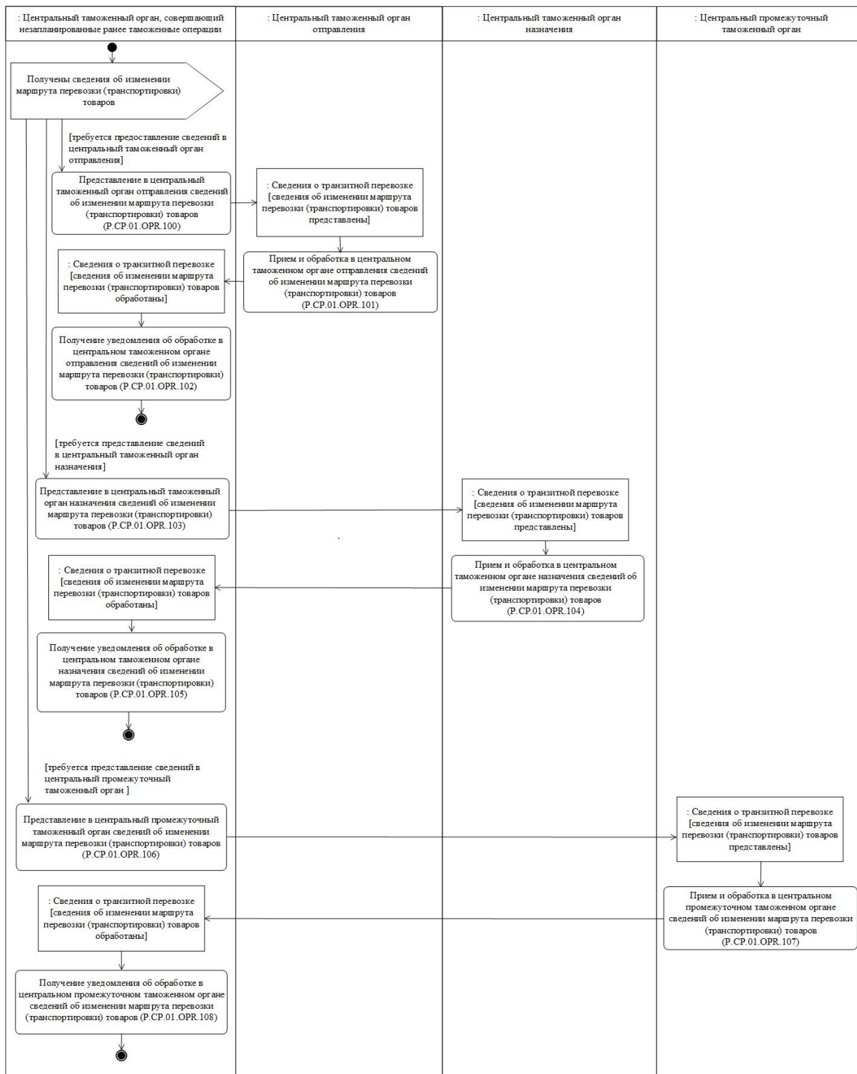
Рис. 20. Схема выполнения процедуры "Информирование об изменении маршрута перевозки (транспортировки) товаров" (Р.СР.01.ПРС.014)
