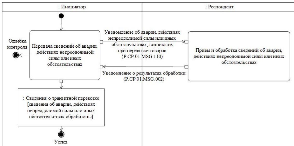
Рис. 38. Схема выполнения транзакции общего процесса "Представление сведений об аварии, действиях непреодолимой силы или иных обстоятельствах" (P.SP.01.TRN.023)
