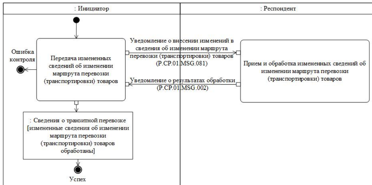
Рис. 30. Схема выполнения транзакции общего процесса "Представление измененных сведений об изменении маршрута перевозки (транспортировки) товаров" (P.SP.01.TRN.015)
