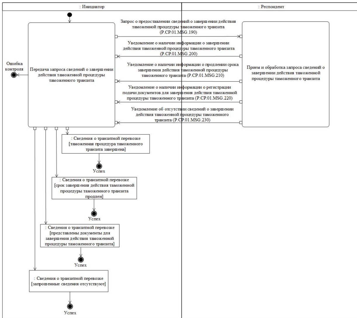
Рис. 44. Схема выполнения транзакции общего процесса "Запрос сведений о завершении действия таможенной процедуры таможенного транзита" (P.SP.01.TRN.029)
