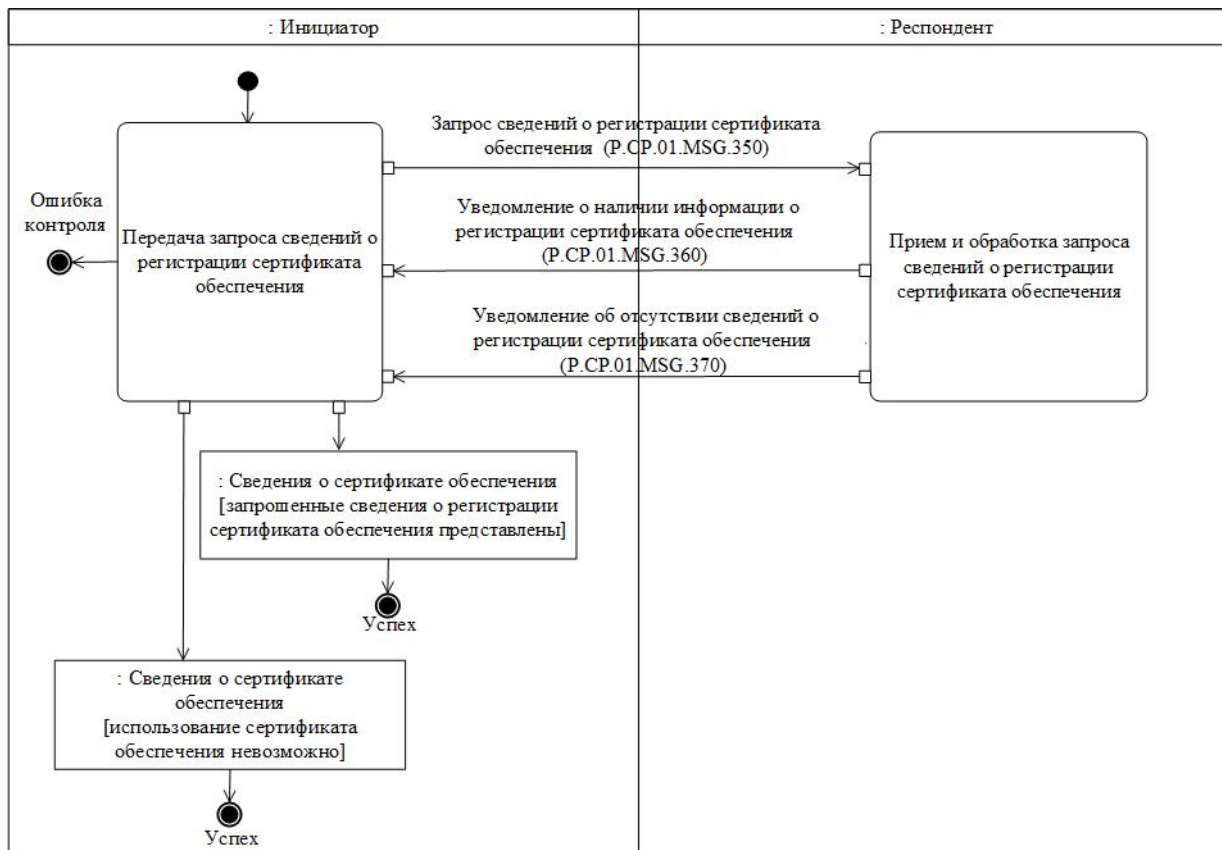
Рис. 52. Схема выполнения транзакции общего процесса "Запрос сведений о регистрации сертификата обеспечения" (P.SP.01.TRN.037)
