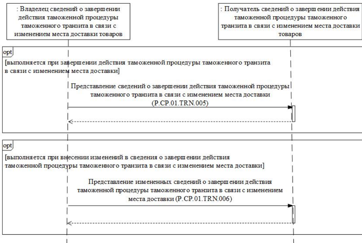
Рис. 4. Схема выполнения транзакций общего процесса при завершении действия таможенной процедуры таможенного транзита в связи с изменением места доставки
