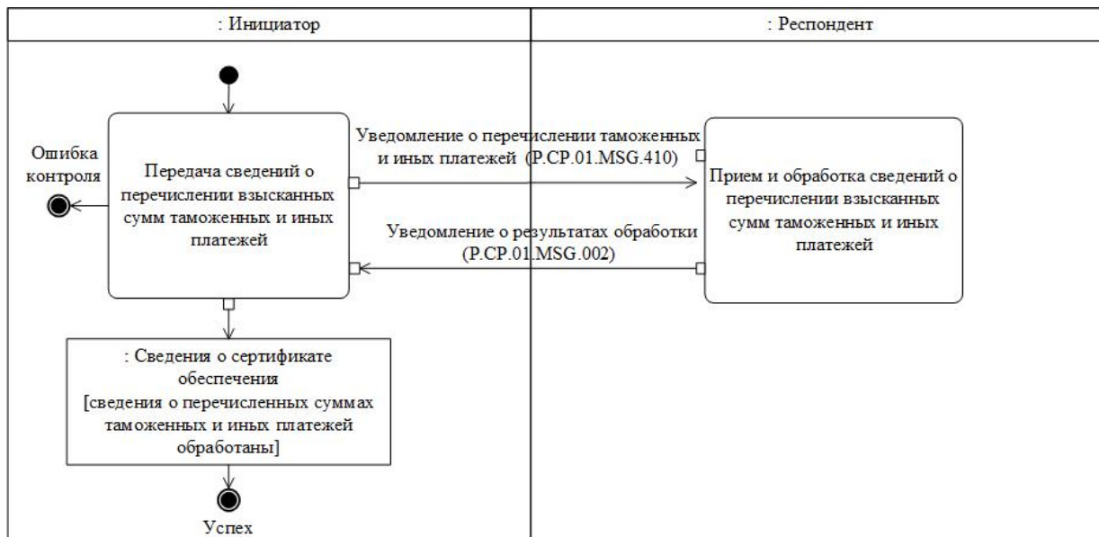
Рис. 56. Схема выполнения транзакции общего процесса "Представление сведений о перечислении взысканных сумм таможенных и иных платежей" (P.SP.01.TRN.041)
