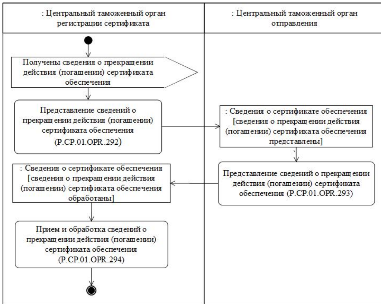
Рис. 49. Схема выполнения процедуры "Информирование о прекращении действия (погашении) сертификата обеспечения" (Р.СР.01.ПРС.043)
