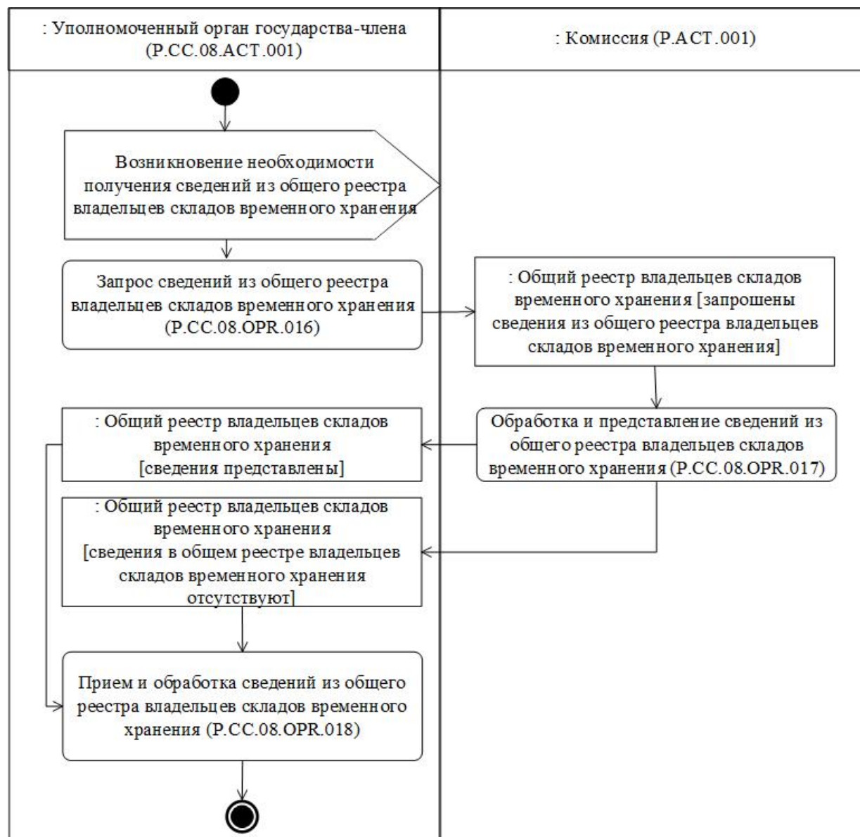
Рис. 10. Схема выполнения процедуры "Получение сведений из общего реестра владельцев складов временного хранения" (Р.СС.08.PRC.005)
