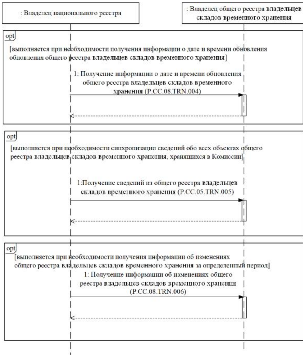
Рис. 3. Схема выполнения транзакций общего процесса при представлении уполномоченным органам государств-членов сведений, содержащихся в общем реестре владельцев складов временного хранения
