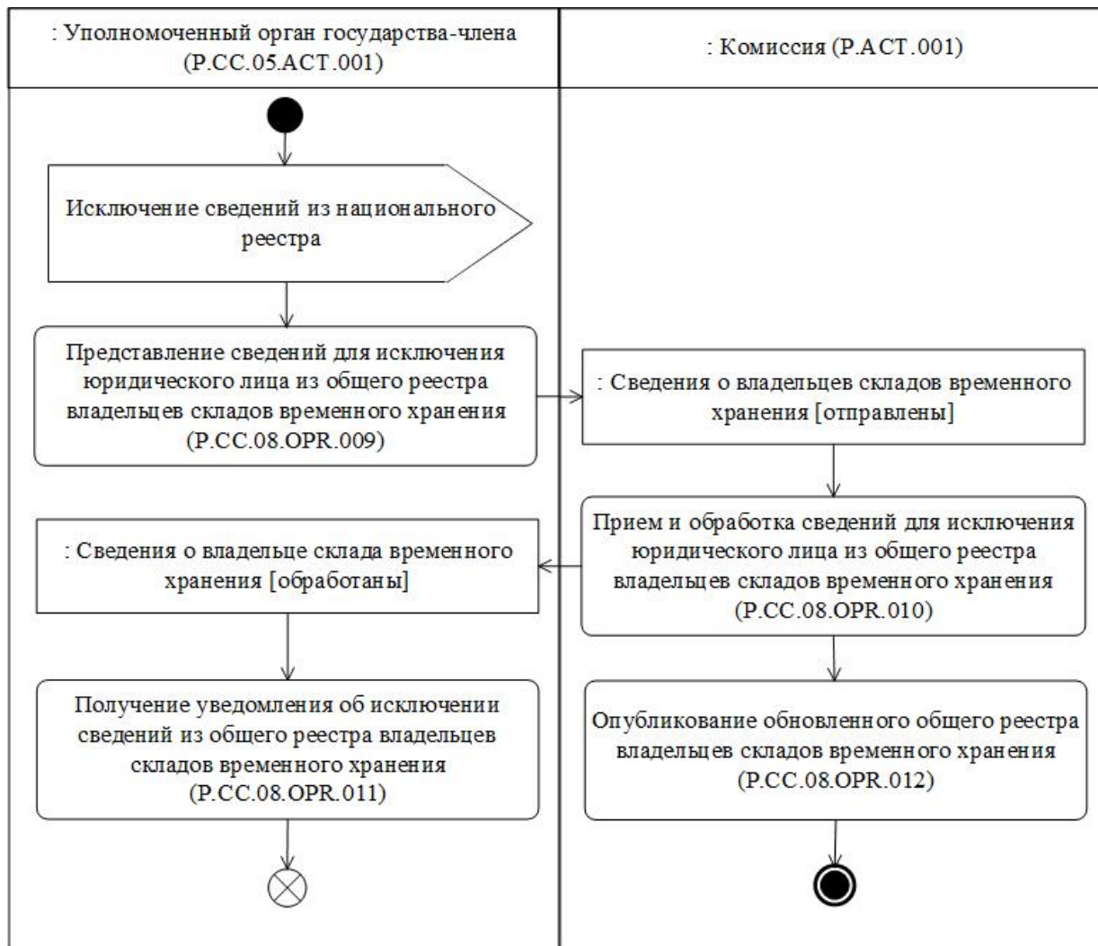
Рис. 7. Схема выполнения процедуры "Исключение сведений из общего реестра владельцев складов временного хранения" (P.CC.08.PRC.003)
