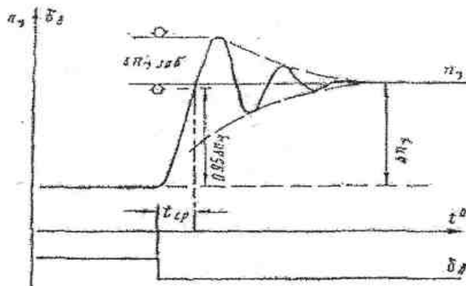
Рисунок 5. Изменение нормальной перегрузки при ступенчатом отклонении руля высоты
