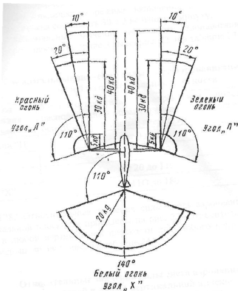
Рис. 22. Светораспределение в горизонтальной плоскости
