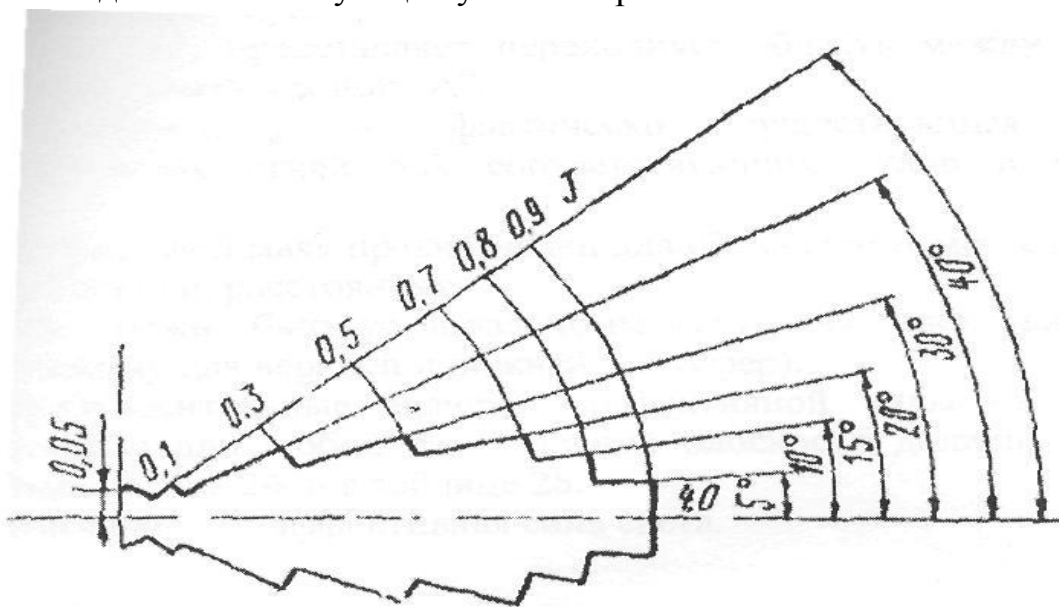
Рис. 23. Светораспределение в вертикальной плоскости
