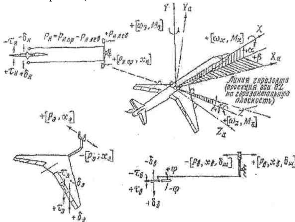
Рисунок 4. Система координат и правила знаков
