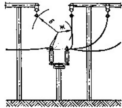
Рис. 9. Наименьшие расстояния от контактов и ножей разъединителей в отключенном положении до заземленных и токоведущих частей
