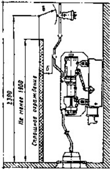
Рис. 13. Наименьшие расстояния между неизолированными токоведущими частями в ЗРУ и сплошными ограждениями (по таблице 133)
