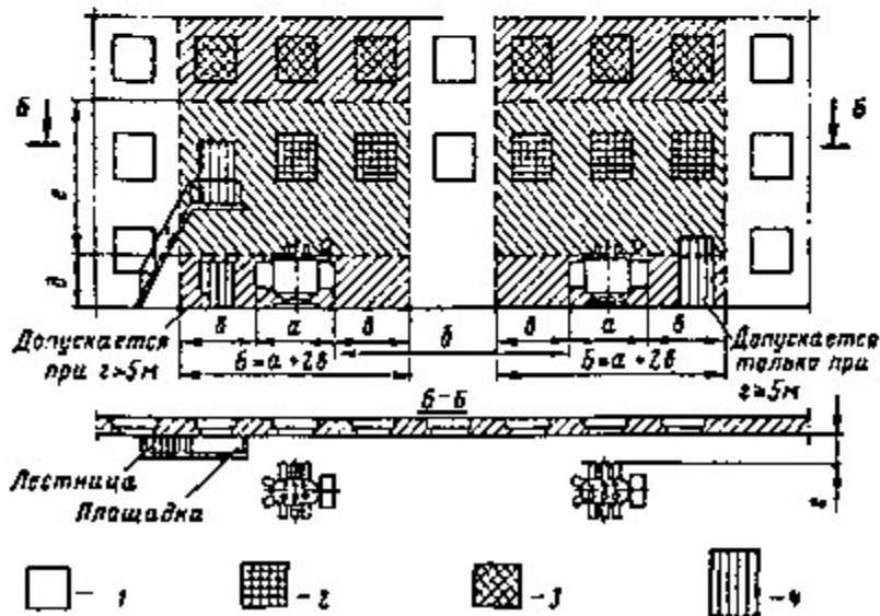
Рис. 11. Требования к открытой установке маслонаполненных трансформаторов у зданий с производствами категории Г и Д (по противопожарным нормам):
