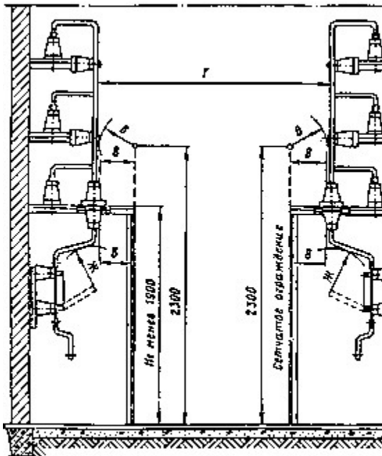
Рис. 14. Наименьшие расстояния от неизолированных токоведущих частей в ЗРУ до сетчатых ограждений и между неогражденными неизолированными токоведущими частями разных цепей (по таблице 133)
