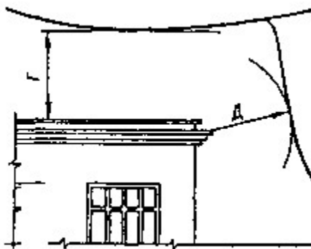
Рис. 10. Наименьшие расстояния между токоведущими частями и зданиями и сооружениями.
