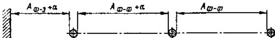
Рис. 2. Наименьшие расстояния в свету при гибких шинах между токоведущими и заземленными частями и между токоведущими частями разных фаз, расположенными в одной горизонтальной плоскости.
