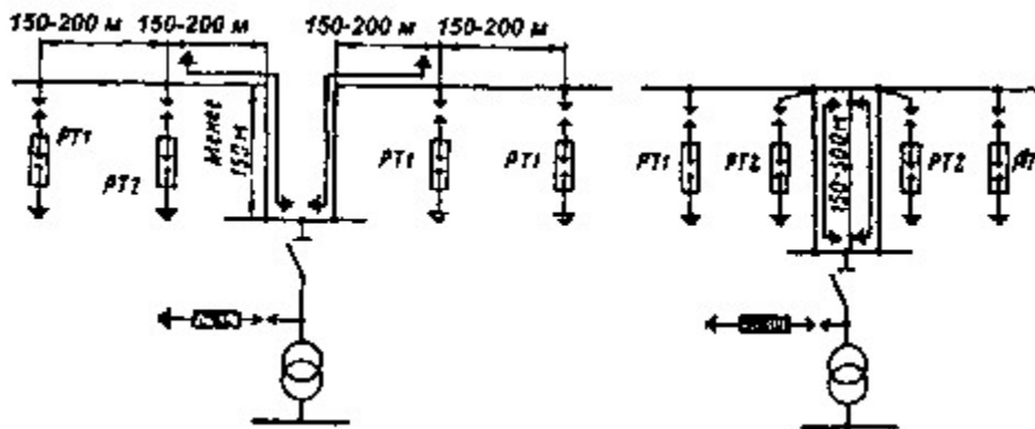
Рис. 17. Схемы защиты от грозовых перенапряжений подстанций, присоединенных к ВЛ с помощью заходов длиной до 150 и более 150 м
