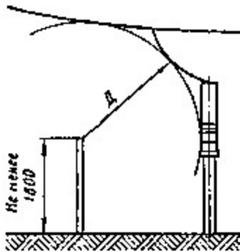
Рис. 8. Наименьшие расстояния от токоведущих частей верхней кромки внешнего ограждения
