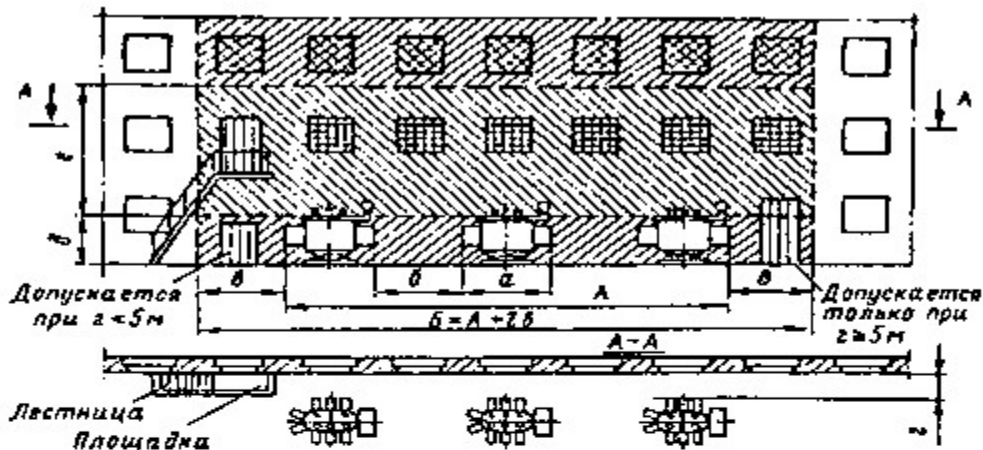
Второй вариант (b > 4м)
