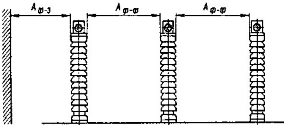
Рис. 1. Наименьшие расстояния в свету при жестких шинах между токоведущими и заземленными частями ( A_{\phi-з} ) и между токоведущими частями разных фаз ( A_{\phi-\phi} )
