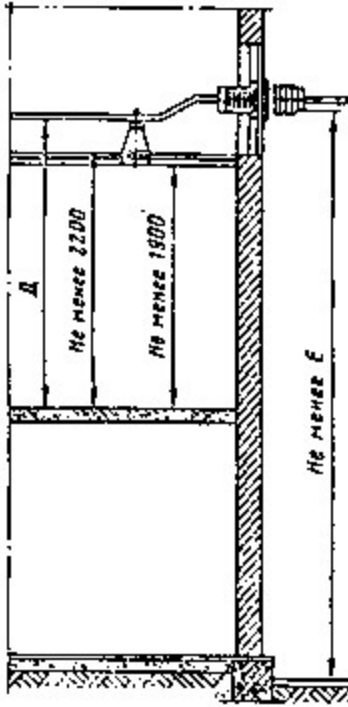
Рис. 15. Наименьшие расстояния от пола до неогражденных неизолированных токоведущих частей и до нижней кромки фарфора изолятора и высота прохода в ЗРУ. Наименьшие расстояния от земли до неогражденных линейных выводов из ЗРУ вне территории ОРУ и при отсутствии проезда транспорта под выводами
