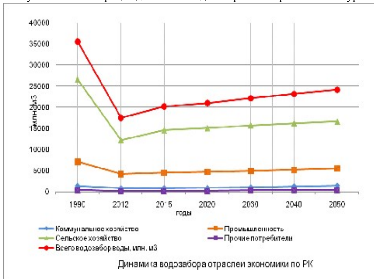
Рисунок 3. Иллюстрация динамики водозаборов на перспективные уровни
