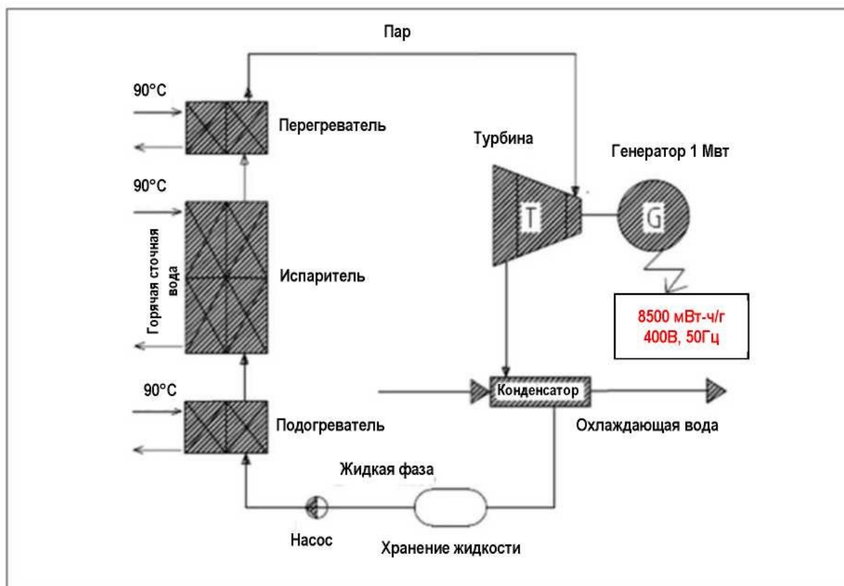
Рисунок 5.11. Производство электроэнергии из низкопотенциального тепла
