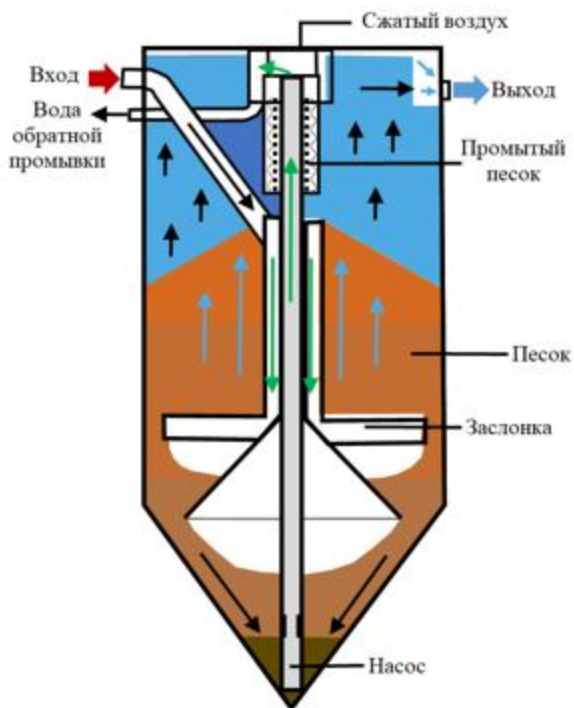
Рисунок 5.7. Принципиальная схема песчаного фильтра
