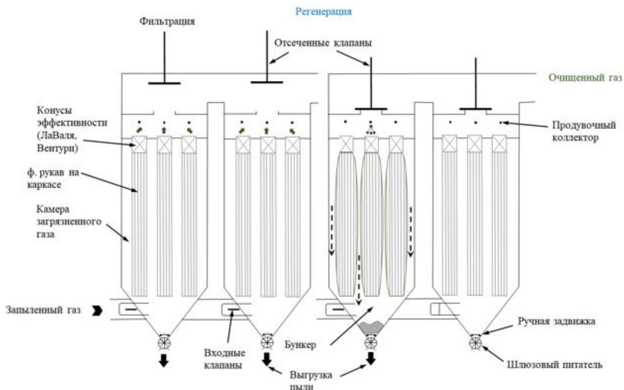
Рисунок 5.2. Принцип работы рукавного фильтра
