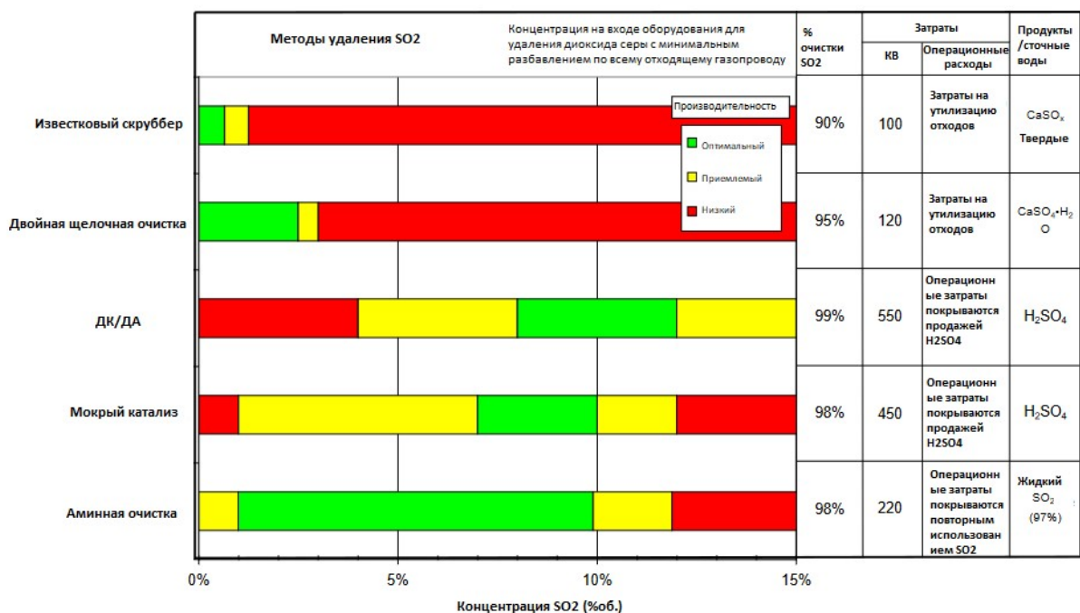
Рисунок 5.6. Эксплуатационные характеристики процессов очистки технологических газов от SO 2 , применяемых в цветной металлургии
