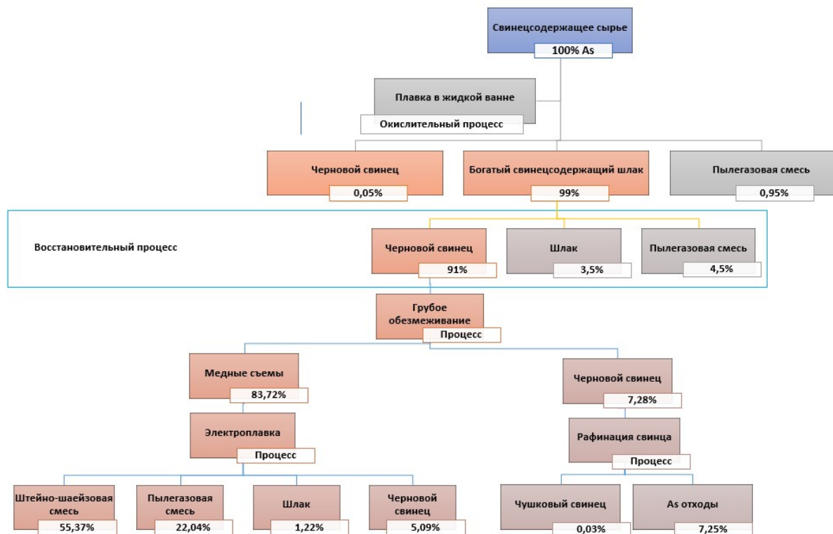
Рисунок 5.9. Схема производства свинца (автогенная окислительная плавка)
