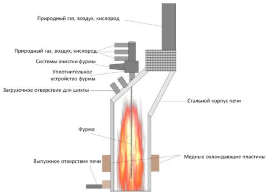
Рисунок 3.3. Схема реактора "Айзасмелт"
