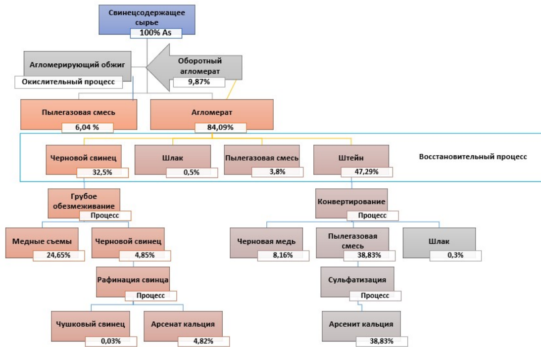
Рисунок 5.8. Схема производства свинца (агломерационный обжиг)
