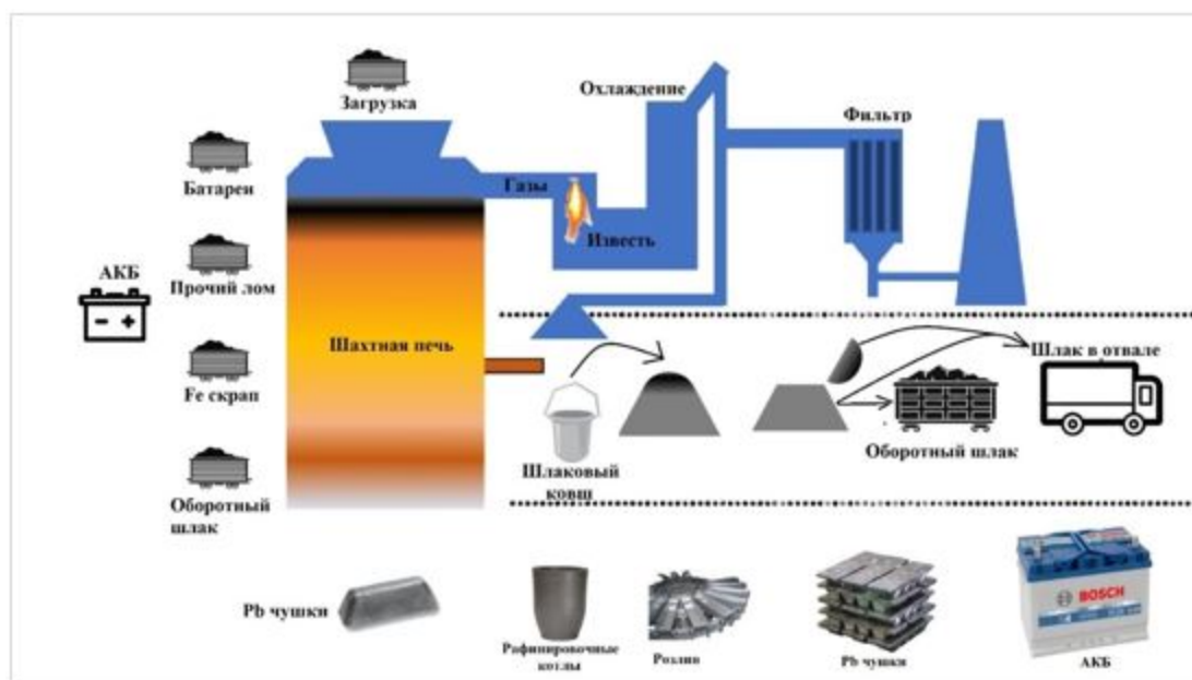
Рисунок 3.5. Схема типичного процесса восстановления аккумуляторных батарей в шахтной печи
