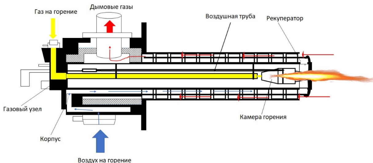
Рисунок 5.10. Рекуперативная горелка Ecomax
