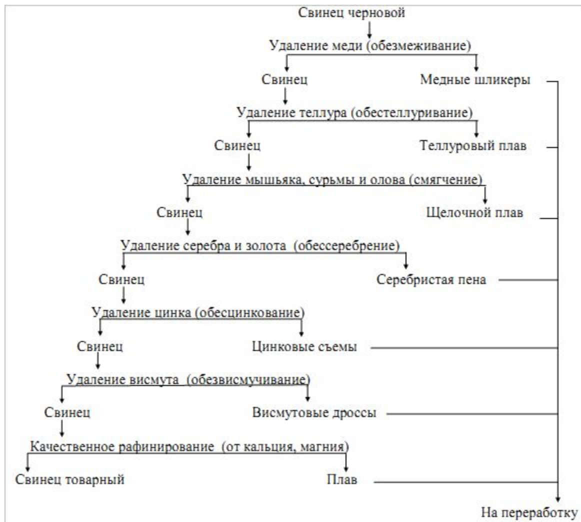
Рисунок 3.6. Схема рафинирования свинца
