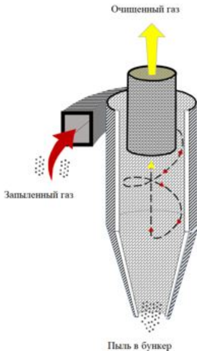
Рисунок 5.1. Конструкция циклона
