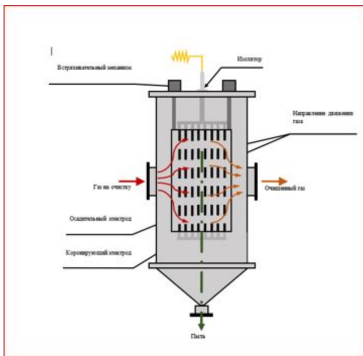
Рисунок 5.2. Принцип действия электрофилтра
