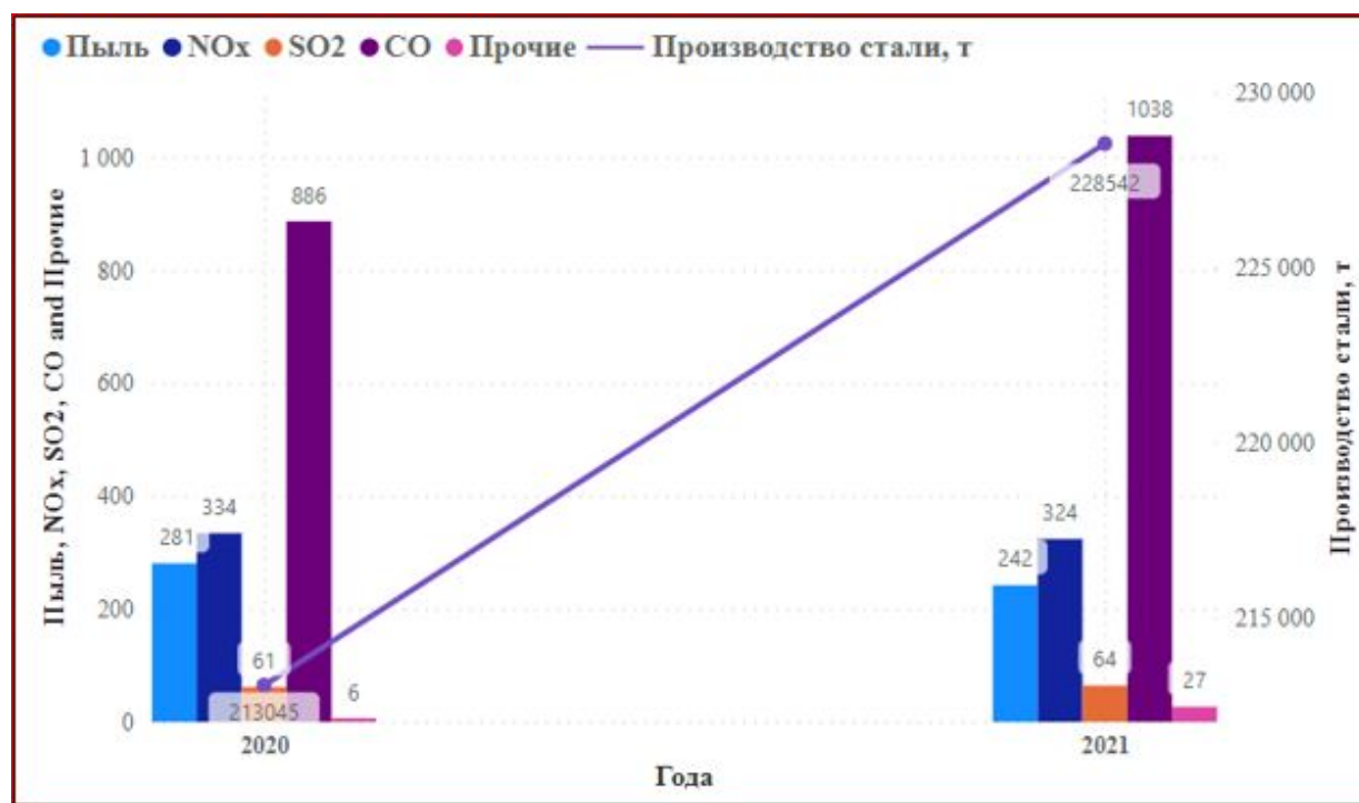
Рисунок 1.9. Выбросы загрязняющих веществ при производстве стали за 2020 – 2021 гг.
